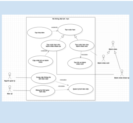
Sơ đồ ca sử dụng
