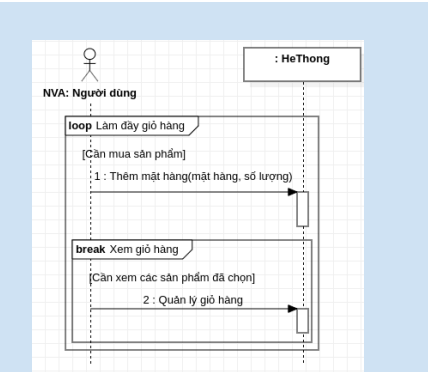
Sơ đồ tuần tự
