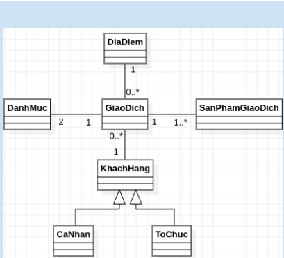
Sơ đồ lớp
