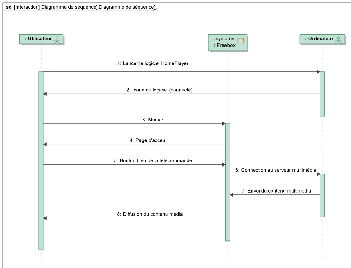
Figure 11 – Diagramme de Séquence
