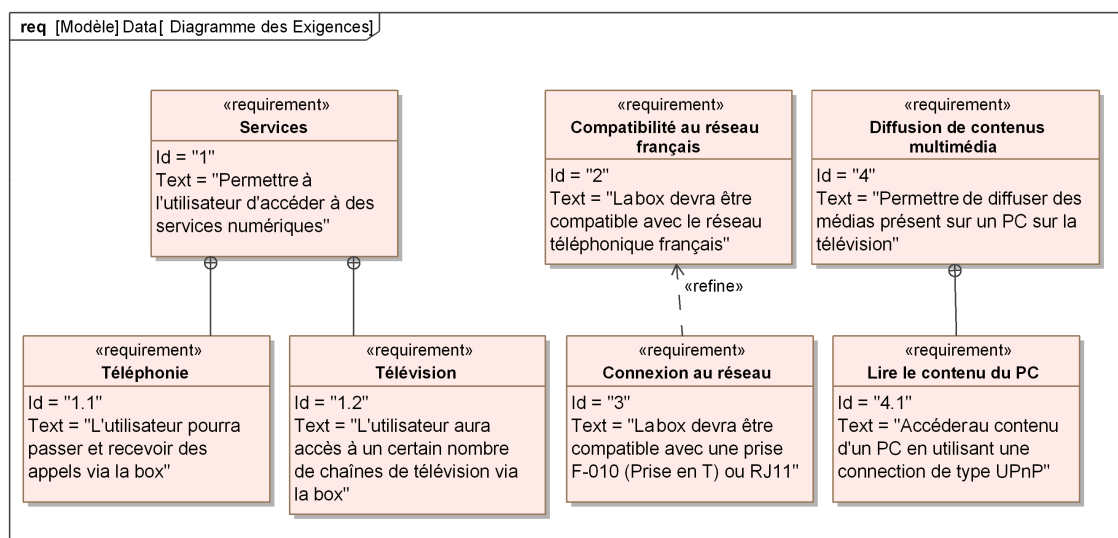
Figure 7 – Diagramme des Exigences
