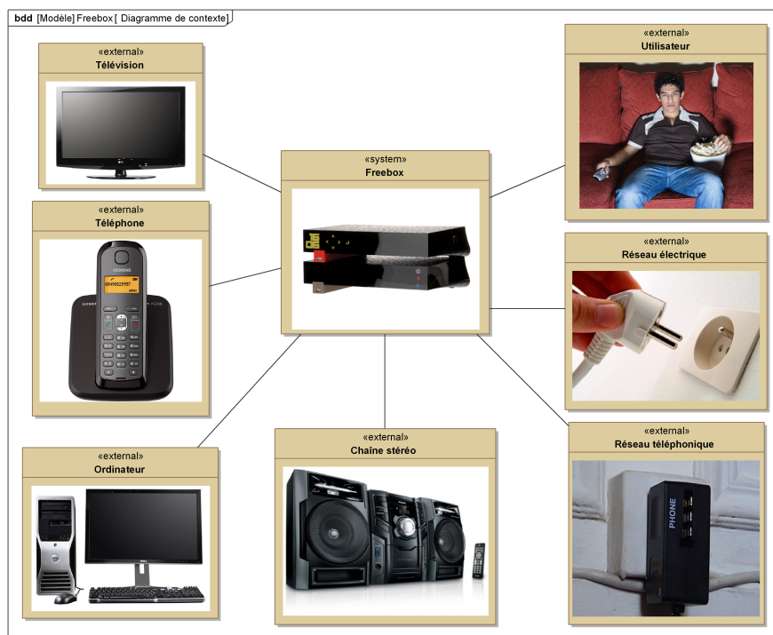
Figure 9 – Diagramme de Contexte
