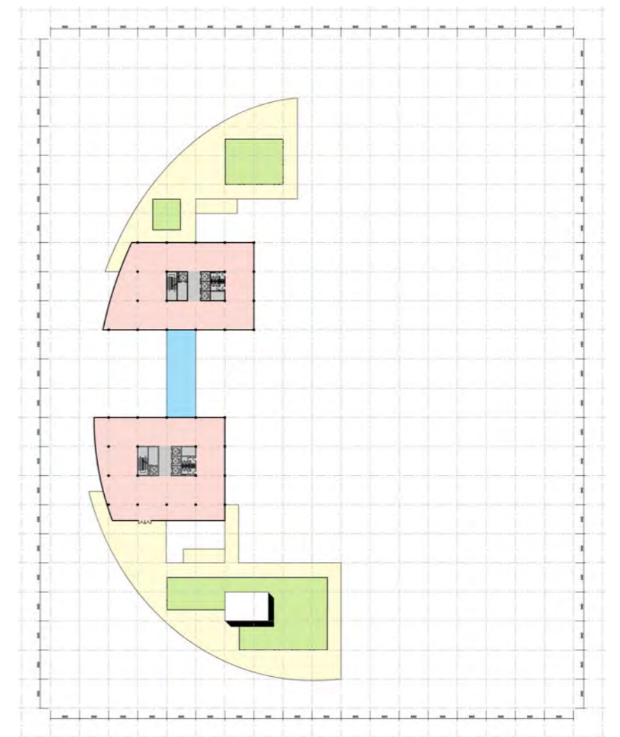
五层平面图
