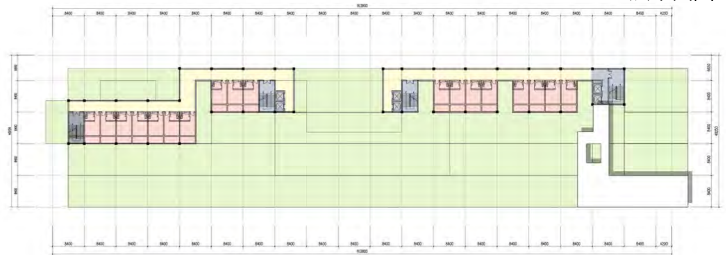
六层平面图
