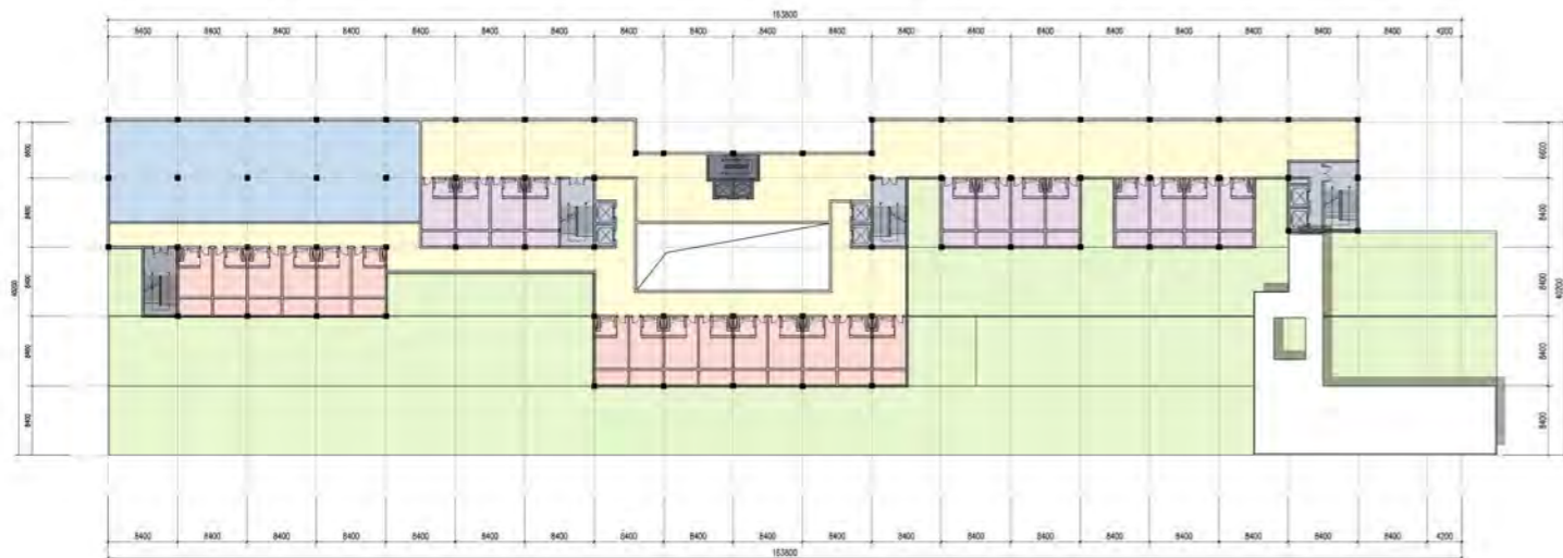
四层平面图
