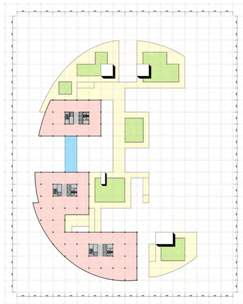
二层平面图
