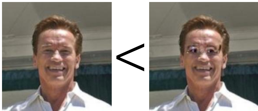
(d) New augmented constraint B < B'
