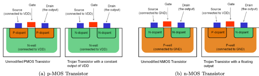
Figura 16.2.: Os Cavalos de Tróia Dopant-Level Escondidos no Hardware por Becker, Regazzoni, Paar, Burleson
