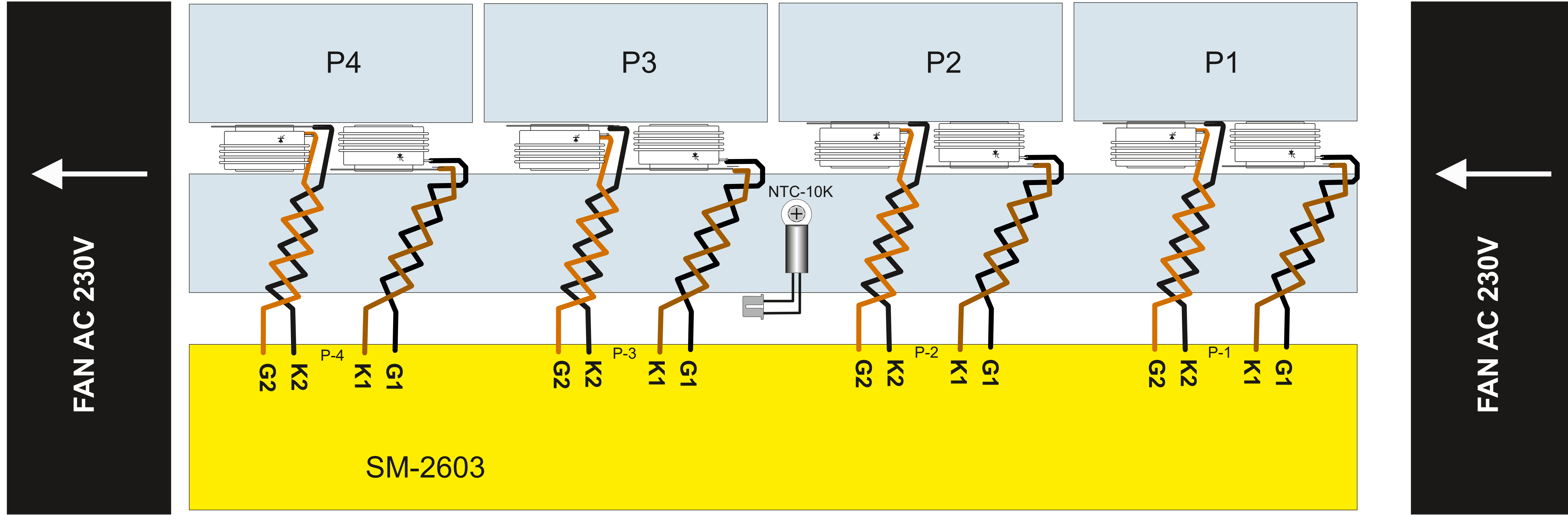
SM-2603 disk tristörün statik voltaj regülatöründe gate kablolarının bağlantı yöntemi Connection method of gate cables in the static voltage regulator of the SM-2603 disk thyristor
