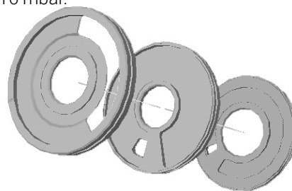
MacroTorr Stages
