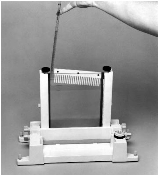
Fig. 5.5. Pouring a heteroduplex analysis gel.
