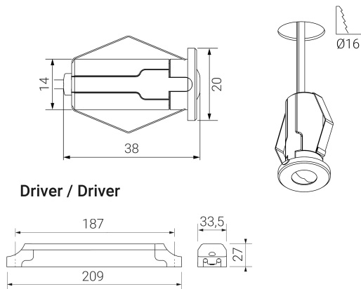
Dimensiones (mm):
