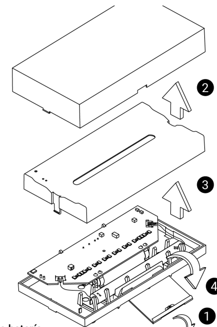
Cambio de batería Battery replacement
