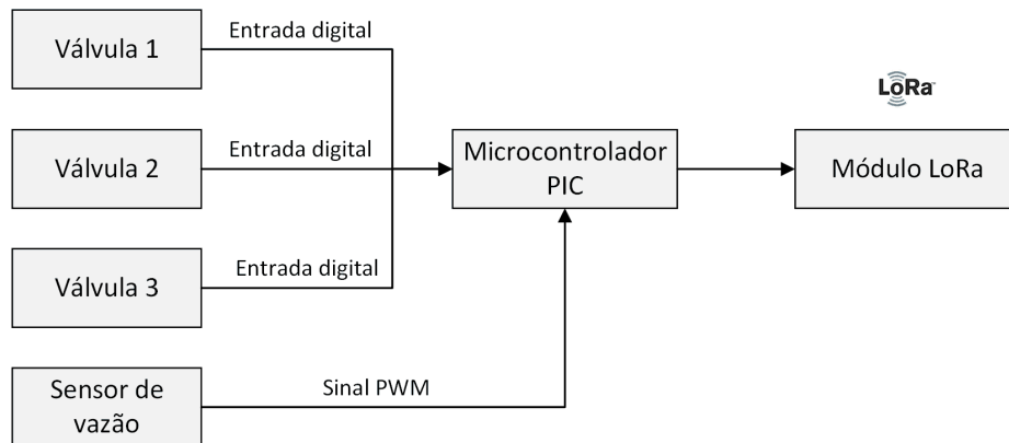
Figura 3 - Fluxograma do processo de captação de dados de vazão
