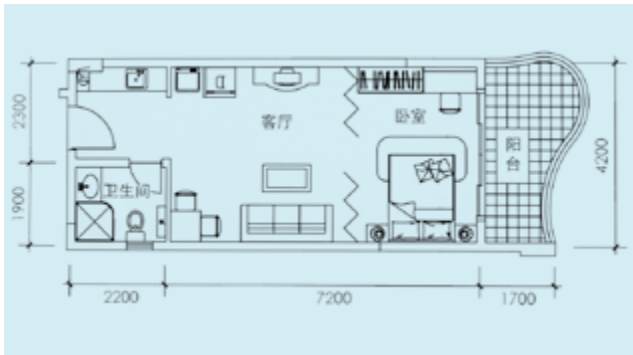
家居设计平面图
