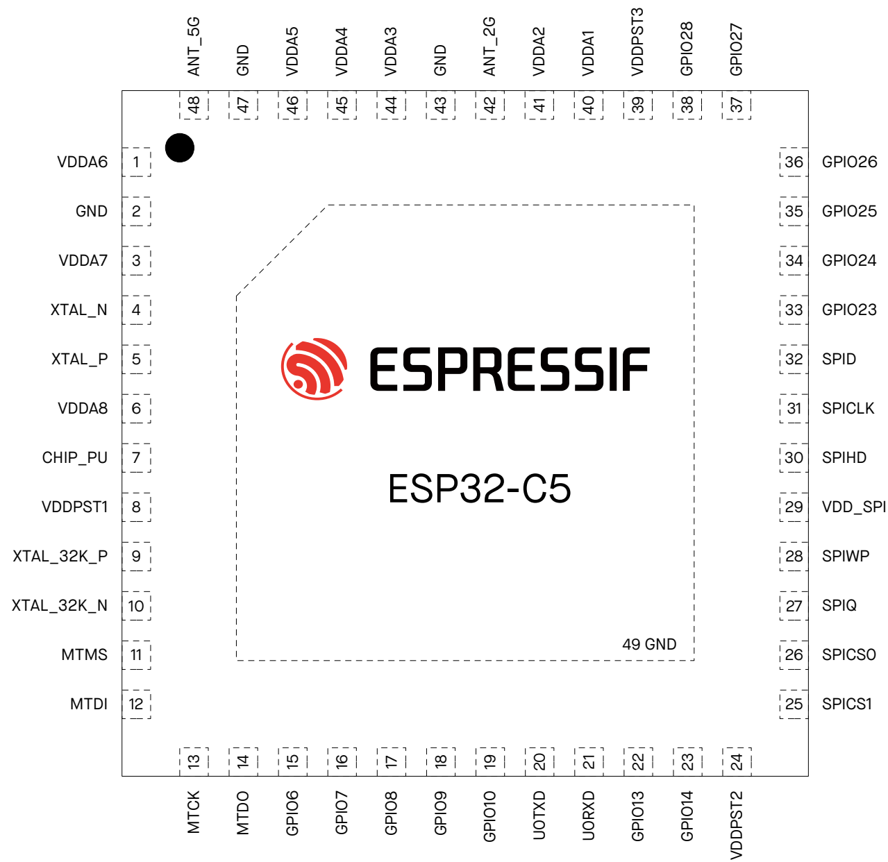
图 2-1. ESP32-C5HR8 管脚布局（俯视图）
