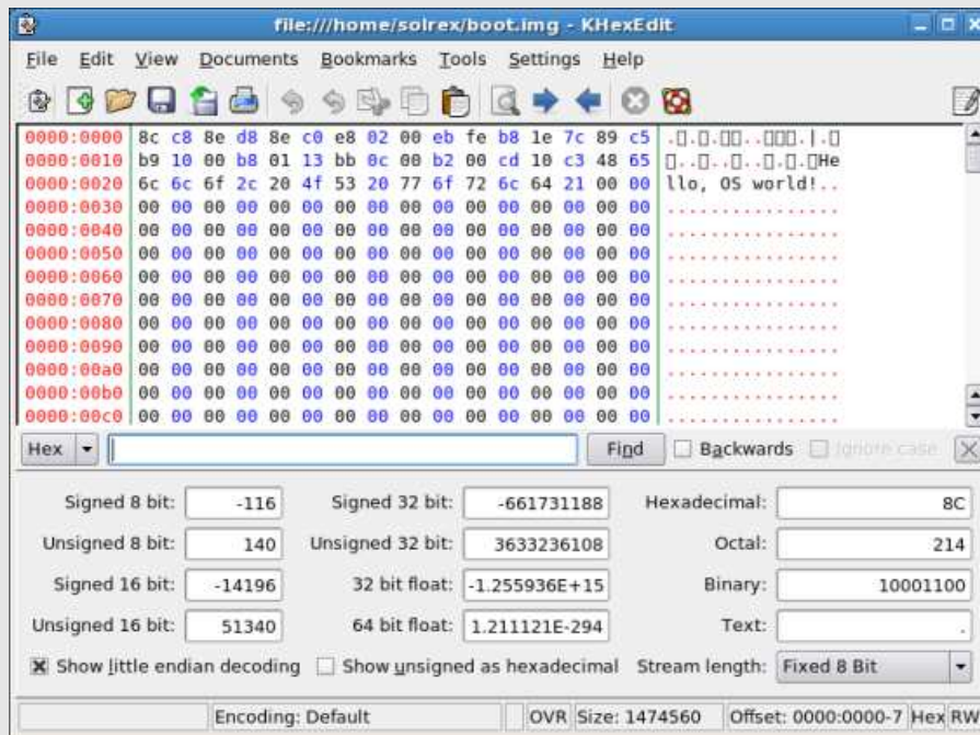
Fig 2.7: 使用 kde 圖形界面工具 khexedit 打開 boot.img
