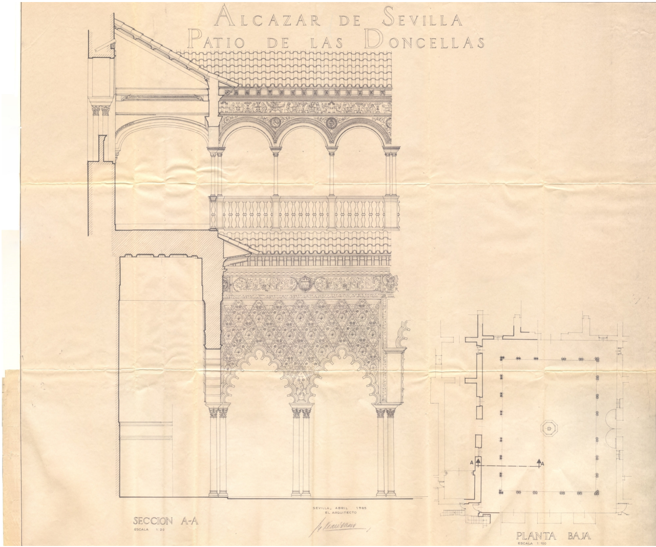
Figure 1.3 – Plano. Sección A-A y Planta Baja del Patio de las Doncellas. Instituto Andaluz del Patrimonio Histórico.
