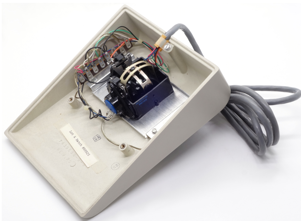
Рис. 5: Джойстик DEC H3060 в разобранном виде
