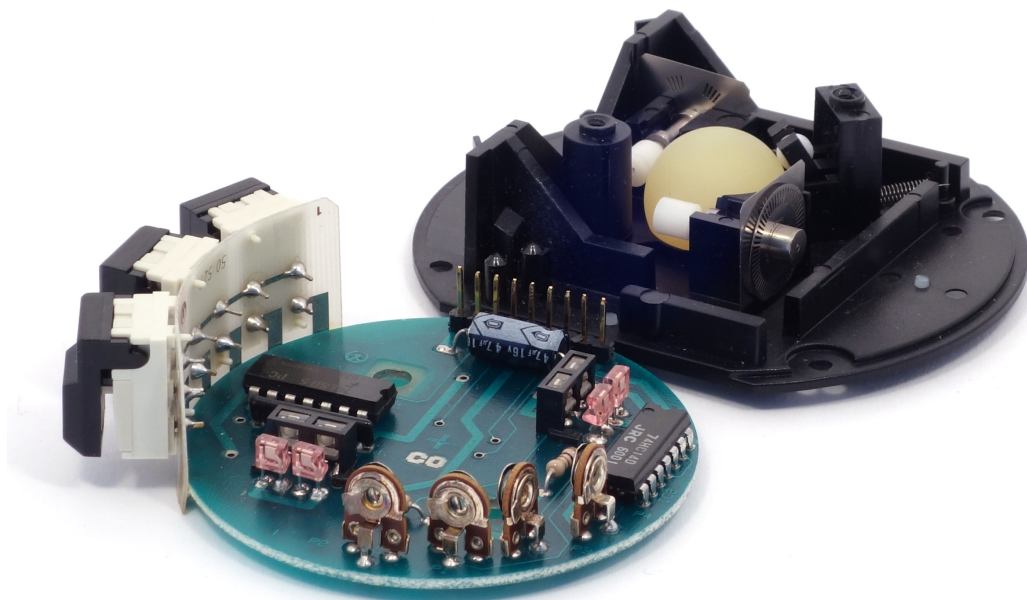
Рис. 5: DIGIMOUSE P4 в разобранном виде
