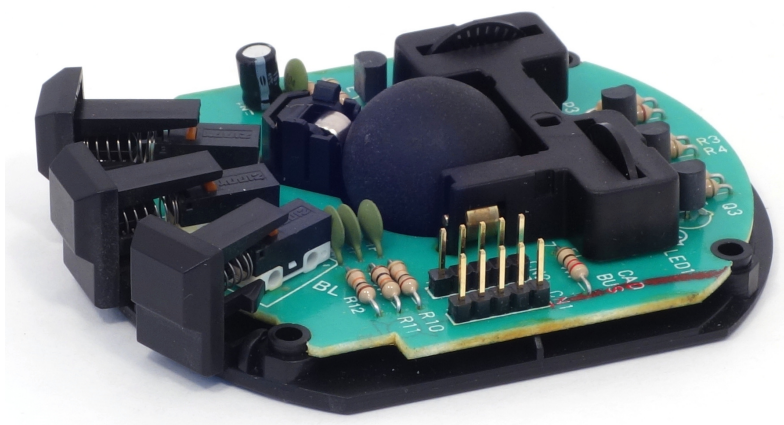
Рис. 7: Sunnyline Hit Mouse в разобранном виде
