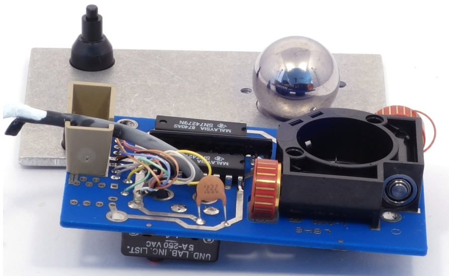
Рис. 5: DEC VS10X-EA в разобранном виде
