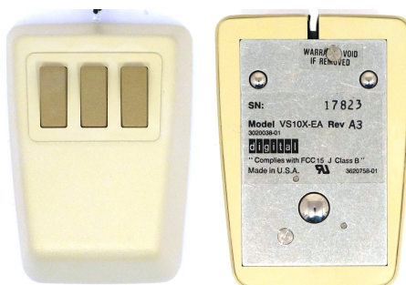
Рис. 2: DEC VS10X-EA Mouse, вид сверху и снизу
