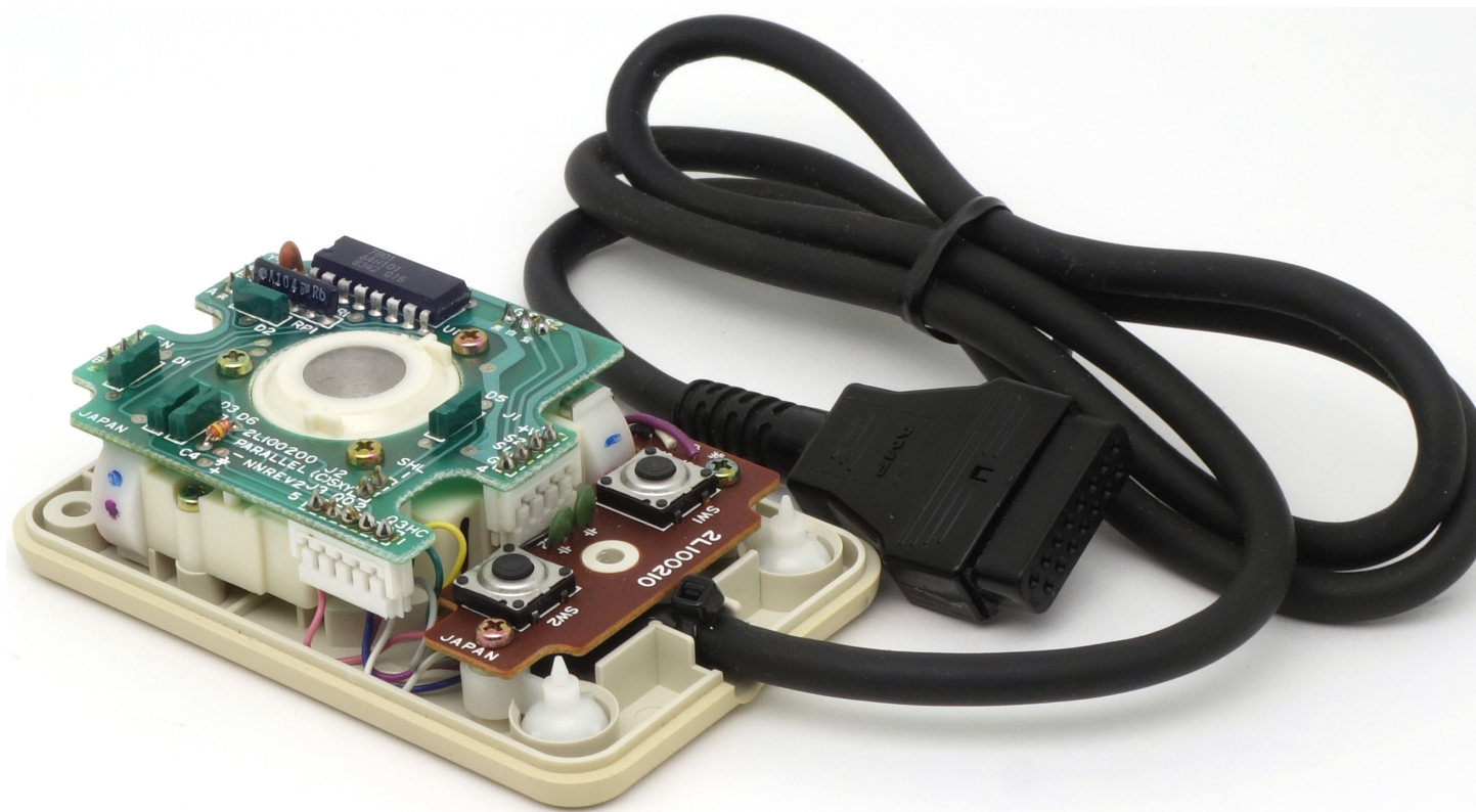
Рис. 5: Mindset Mouse в разобранном виде
