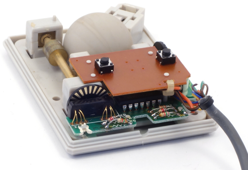
Рис. 5: Commodore C300 Mouse в разобранном виде
