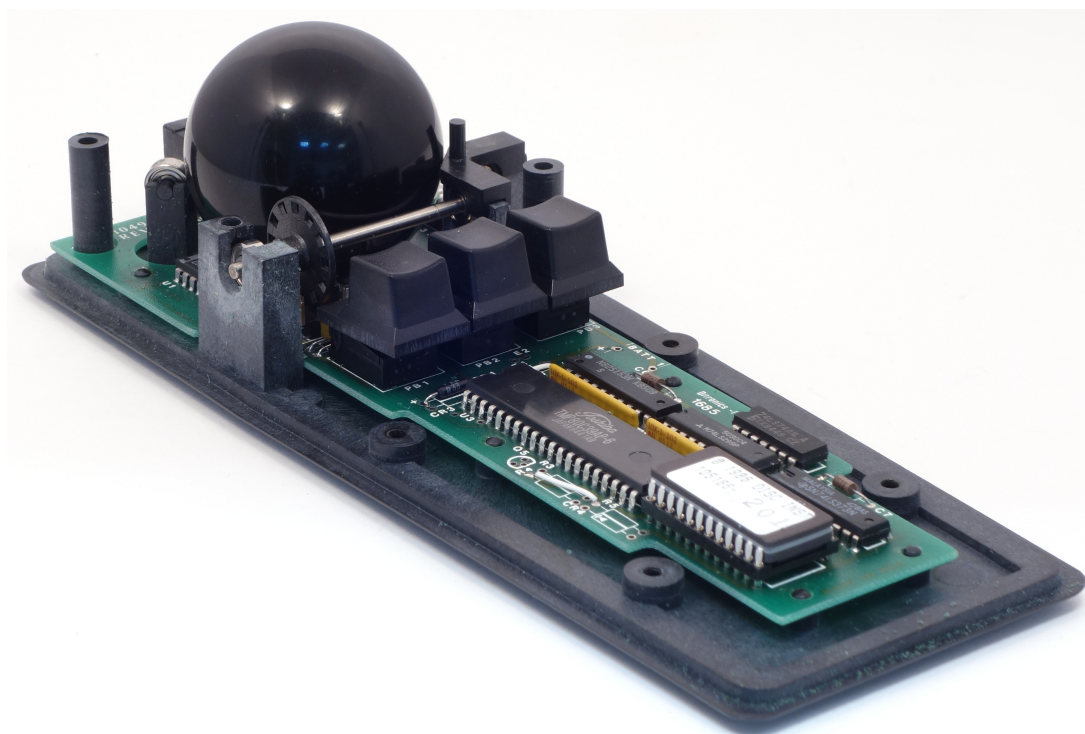
Рис. 5: microLYNX в разобранном виде
