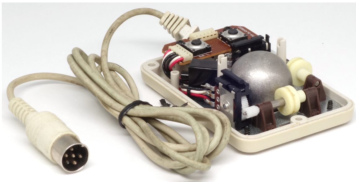
Рис. 5: Tandy Deluxe Mouse в разобранном виде
