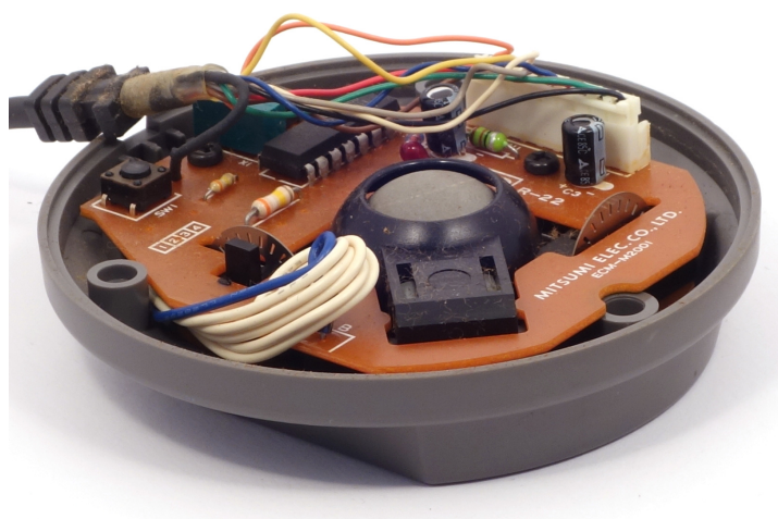
Рис. 5: Мышь Fujitsu FMT-MO101 в разобранном виде
