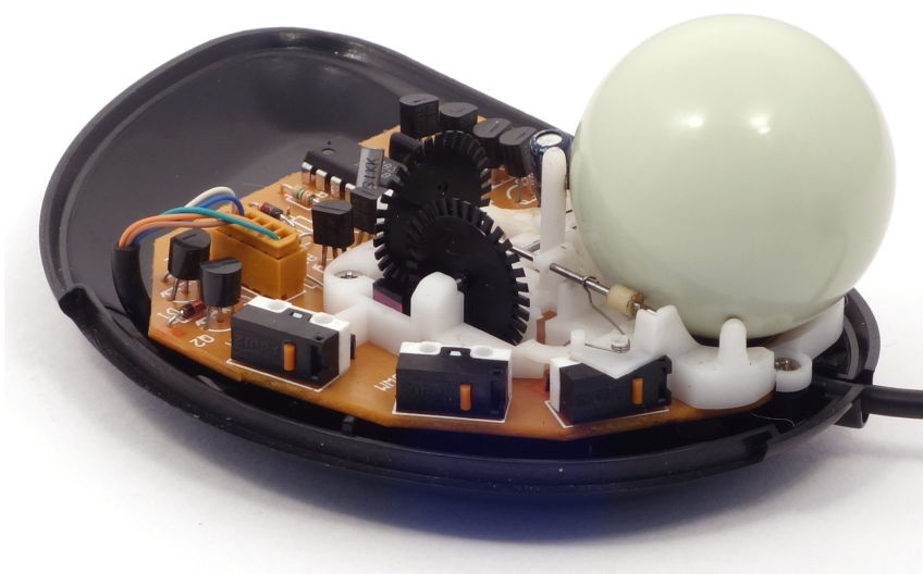
Рис. 5: Colani Trackball в разобранном виде
