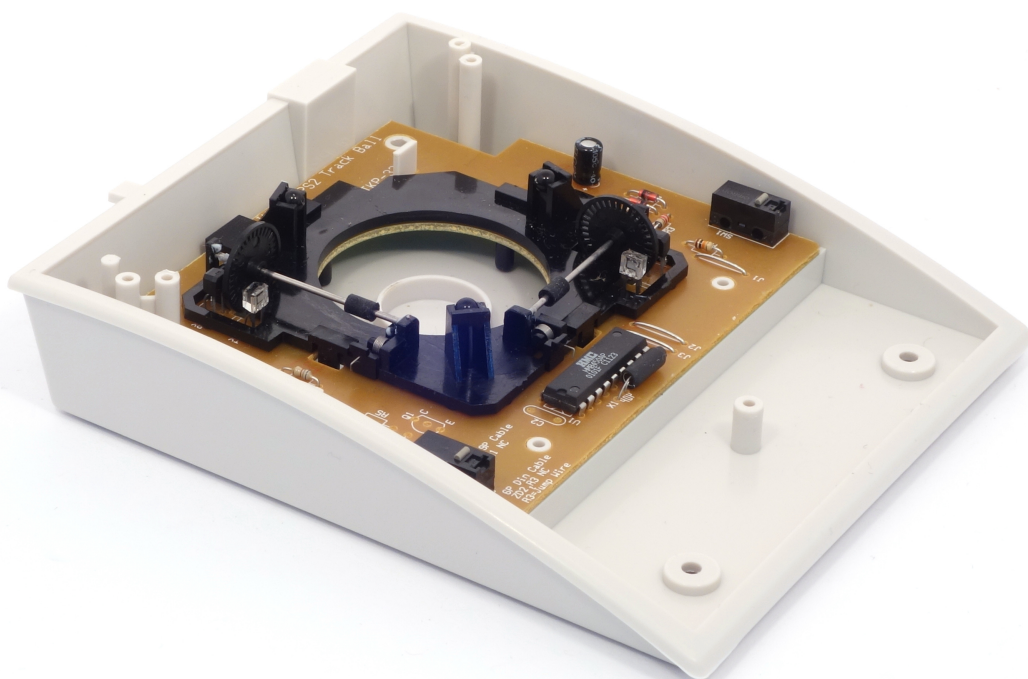
Рис. 5: Fellowes Trackball в разобранном виде
