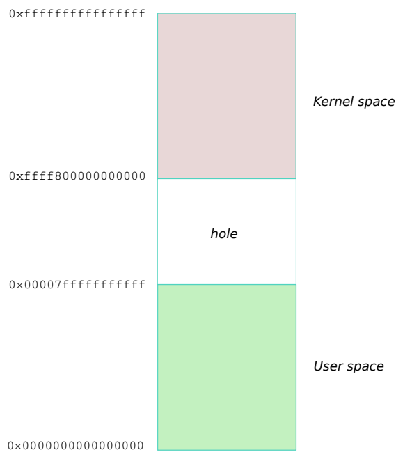
Figura 5.6: Espacios de memoria para usuario y kernel en Linux.
