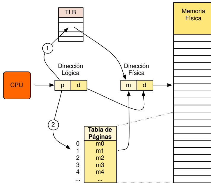
Figura 5.12: Esquema de paginación con TLB, en el paso 1 se consulta la TLB y si no encuentra el número de página, en el paso 2 se consulta la tabla de páginas.
