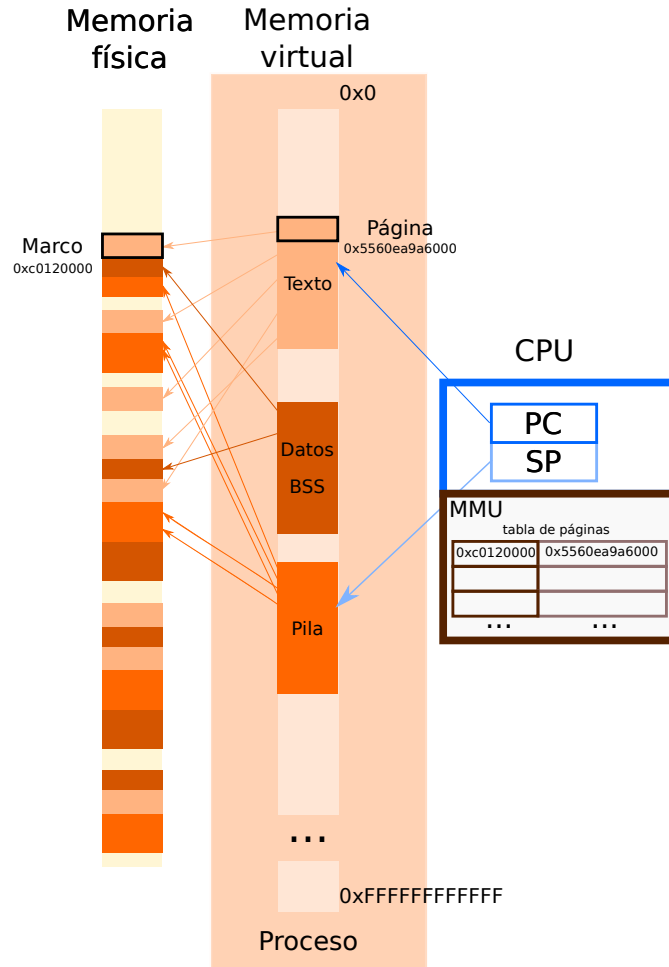
Figura 5.7: Los procesos tienen un espacio virtual que se traduce a partes no contiguas en la memoria física.
