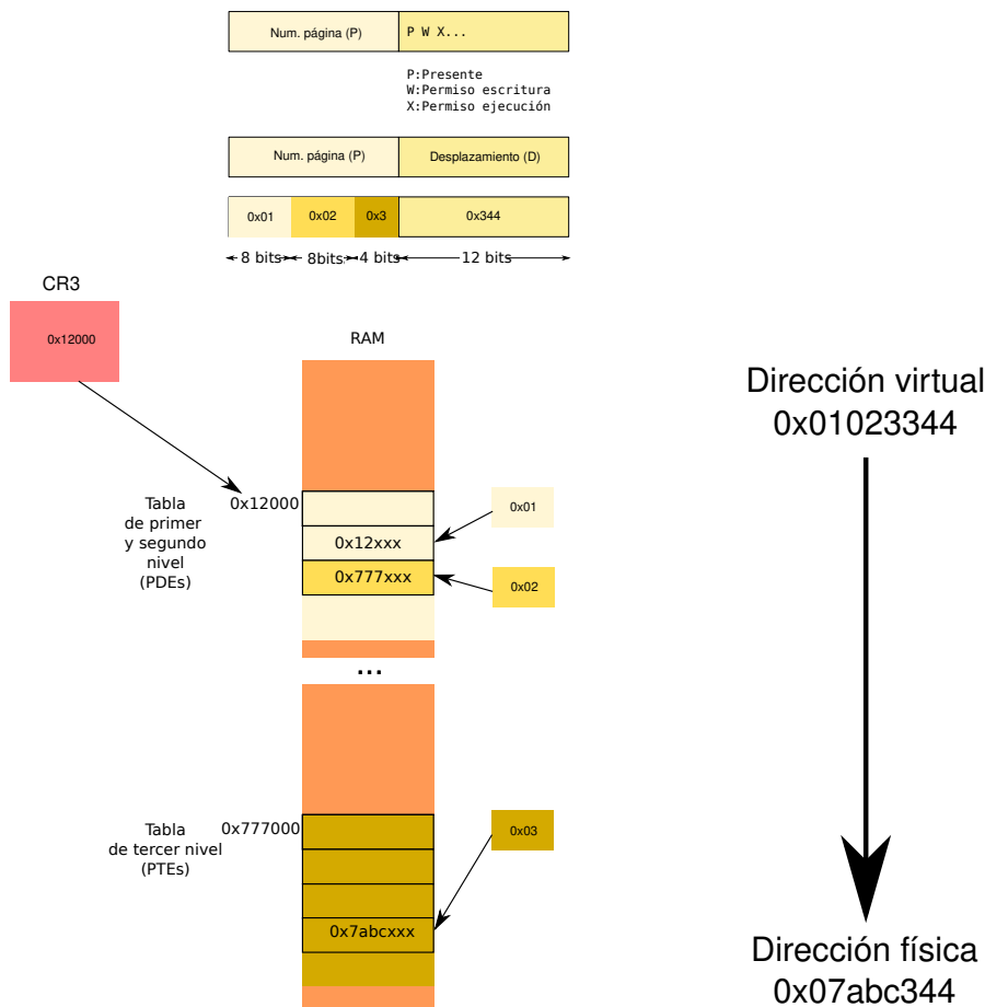
Figura 5.16: Ejemplo de traducción multinivel con entrada autorreferente.
