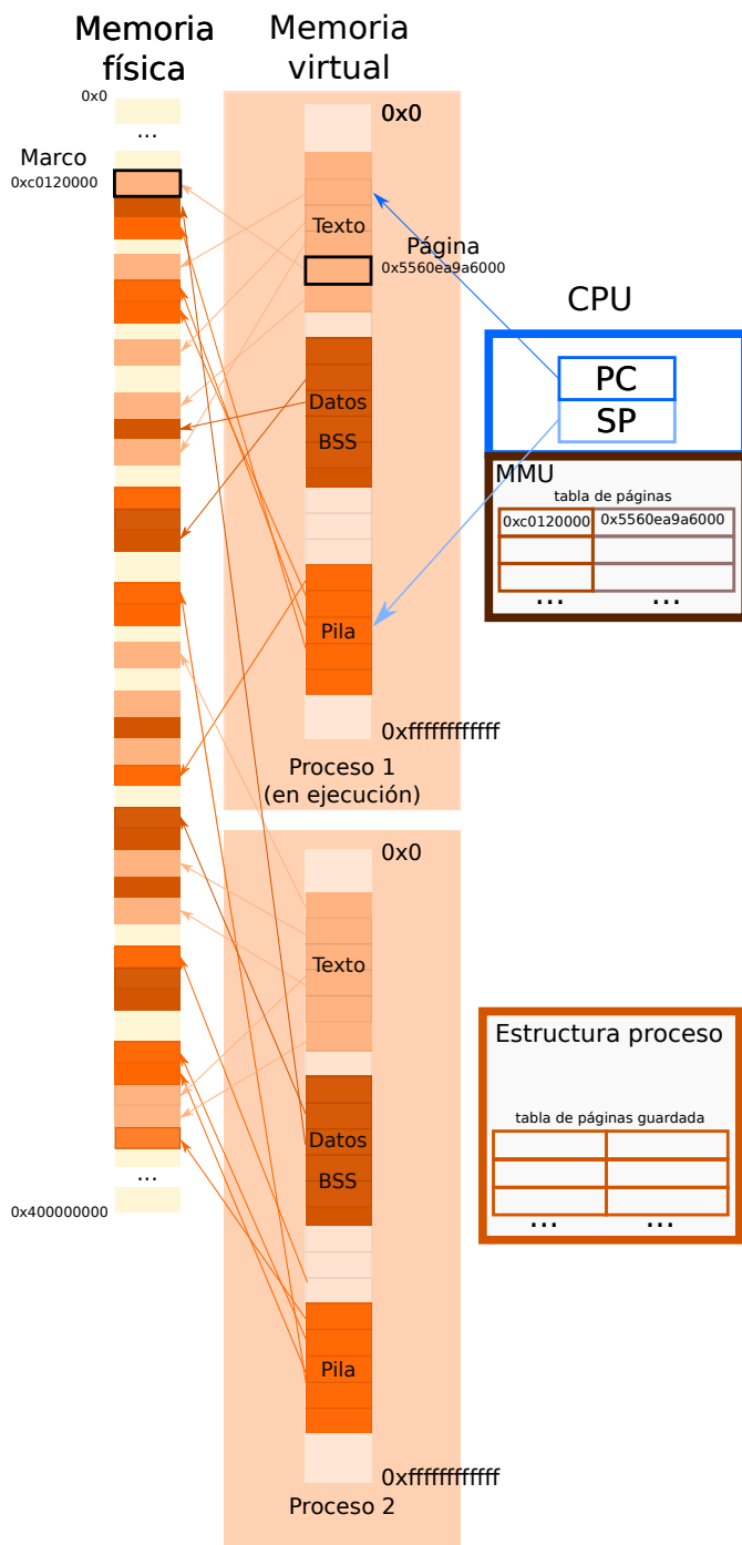
Figura 5.8: Cada proceso tiene su propio espacio de direcciones virtuales (que suele ser mucho más grande que la física).
