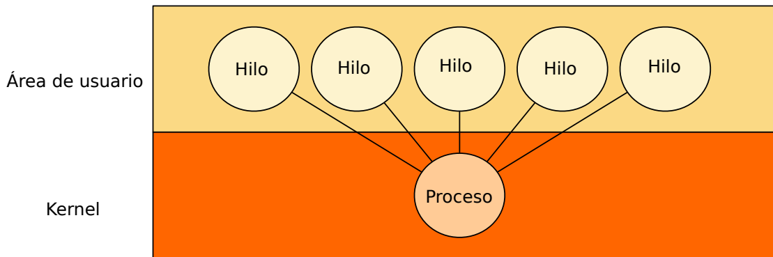
Figura 7.2: Hilos de biblioteca (N-1).
