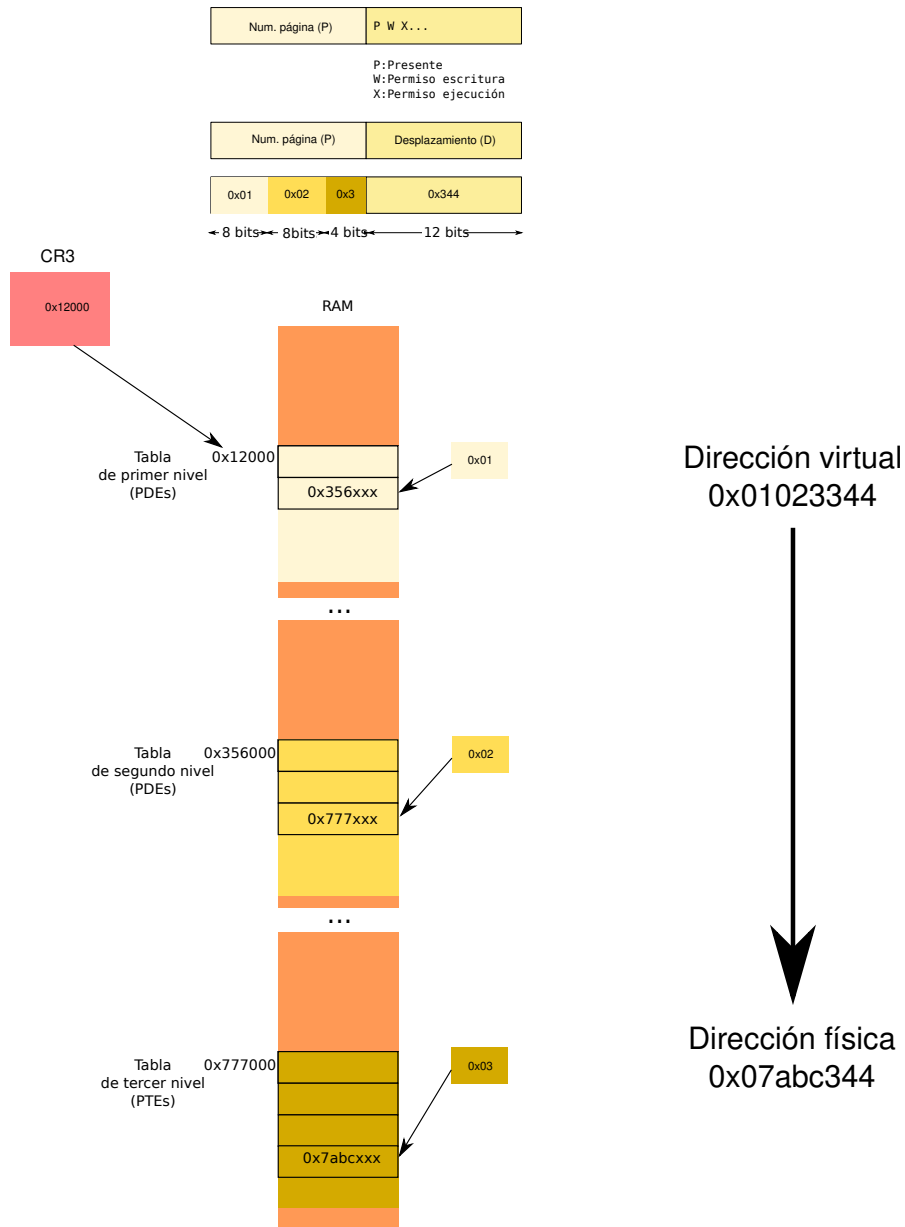
Figura 5.15: Ejemplo de traducción multinivel.
