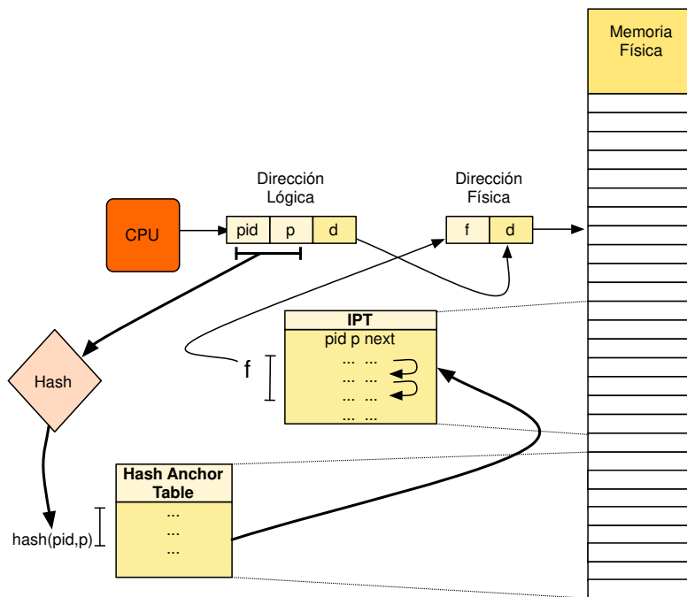
Figura 5.14: Esquema de paginación con IPT y hash
