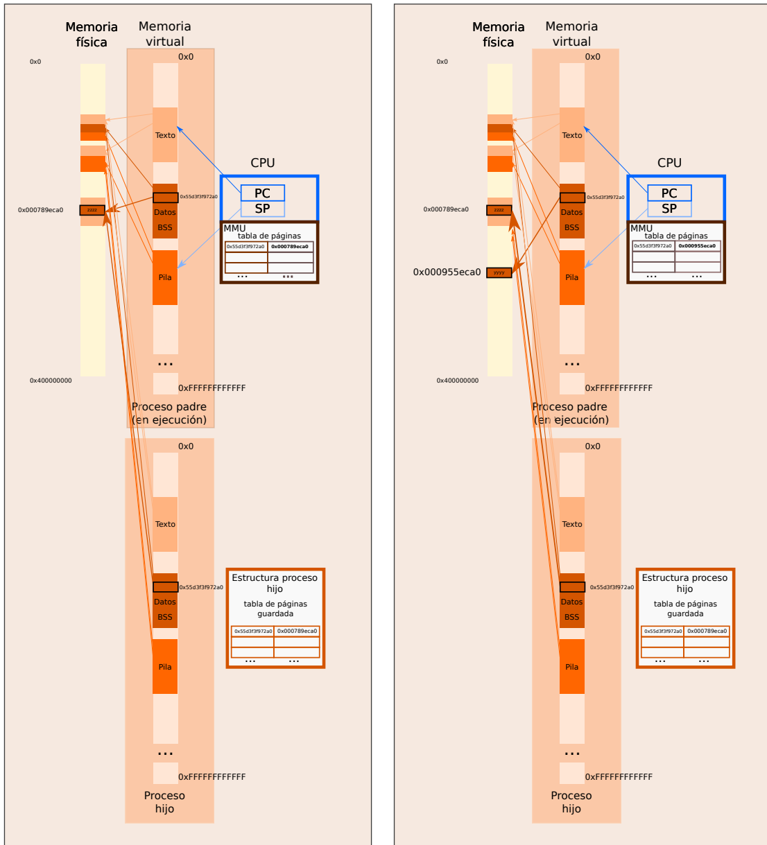
Figura 5.18: Cuando una página se modifica, su marco se duplica y se instala una nueva traducción.
