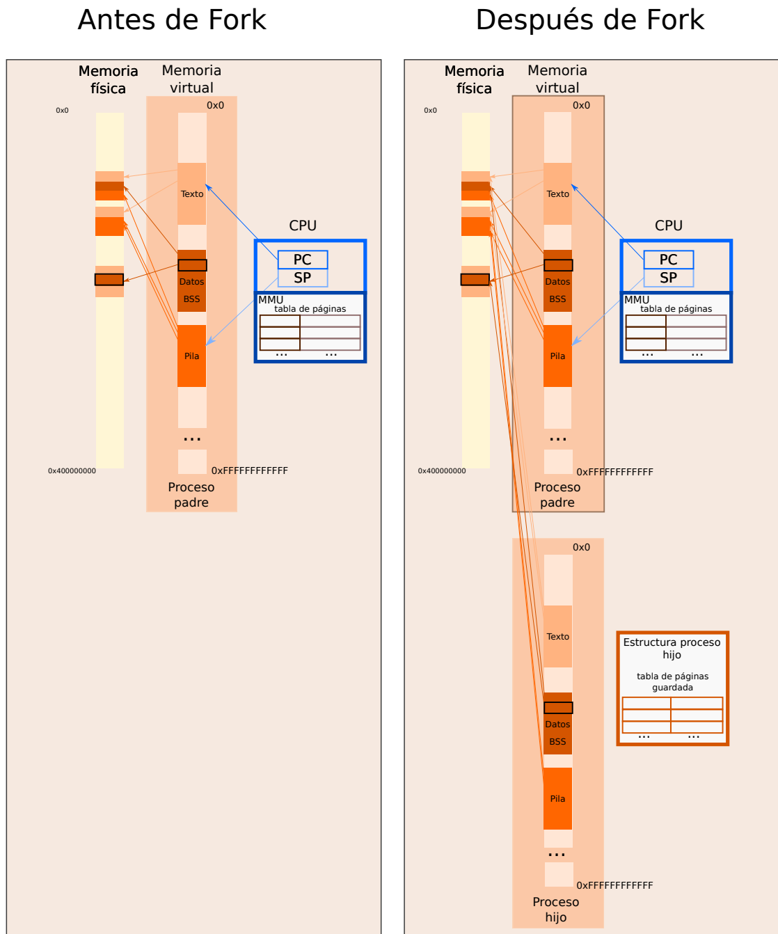
Figura 5.17: Justo después de fork , los procesos comparten todos los marcos de página.
