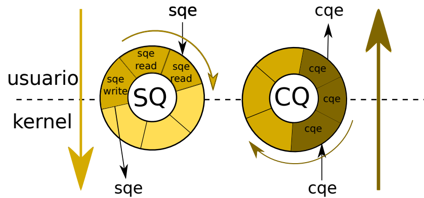
Figura 4.12: Anillos compartidos entre memoria y kernel en io_uring
