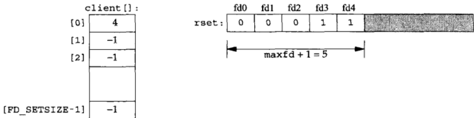
图6-17 第一个客户连接建立后的数据结构
