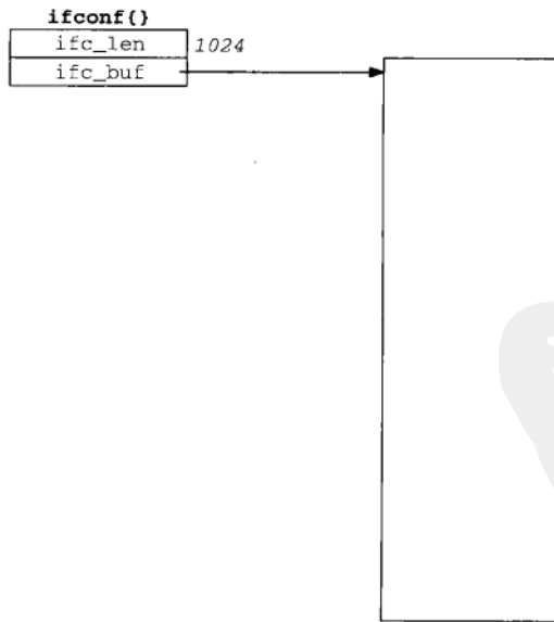
图17-3 SIOCIFCONF前ifconf结构的初始化结果
