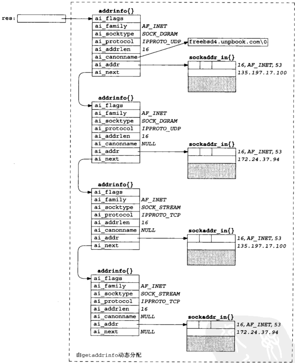
图11-5 getaddrinfo 返回信息的实例
