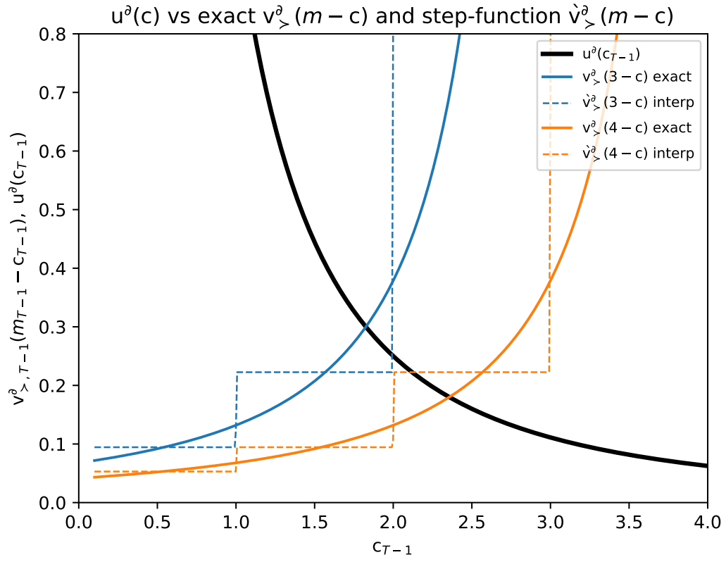
Figure 6 u^c(c) versus v_{>(T-1)}^\delta(3-c) , v_{>(T-1)}^\delta(4-c) , \hat{v}_{>(T-1)}^\delta(3-c) , \hat{v}_{>(T-1)}^\delta(4-c)
