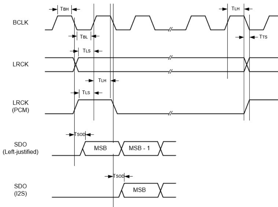
图表 2-17 I2S &amp; PCM 接口发送时序图
