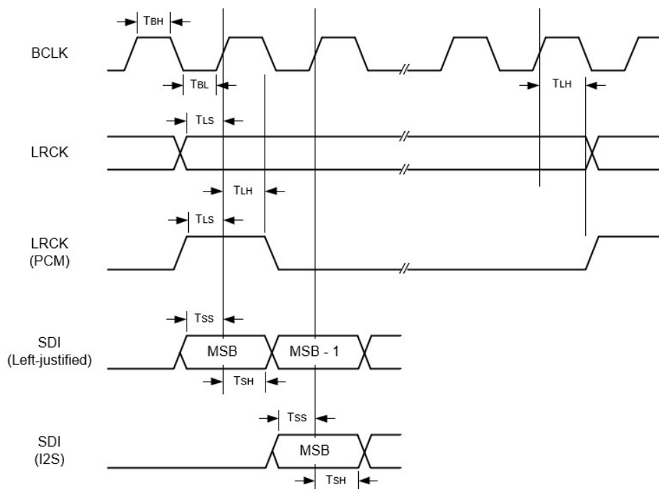
图表 2-16 I2S &amp; PCM 接口接收时序图
