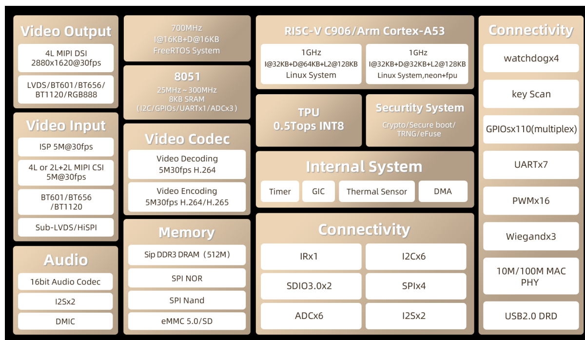
图表 1-3 SG2000 框图
