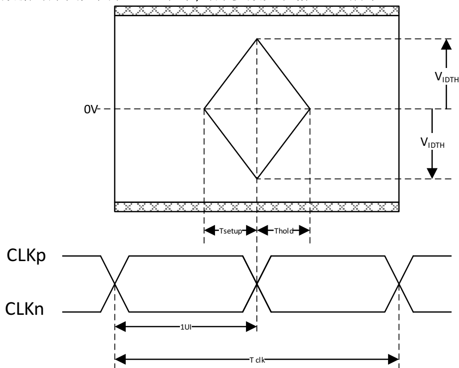
图表 2-22. HiSPi 时钟数据时序图
