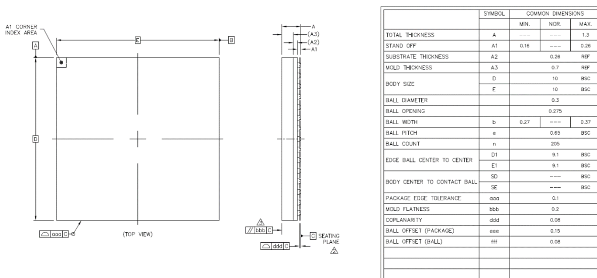
图表 2-1 SG2000 封装外观尺寸, 上视图
