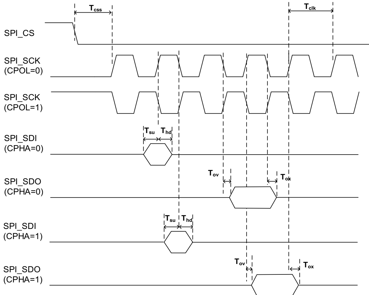
图表 2-19 SPI 接口时序图
