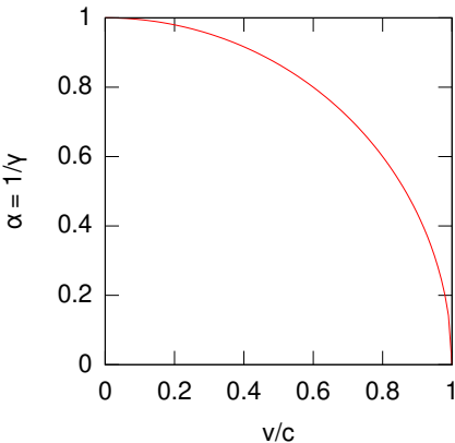
'Lorentz_factor_inverse.svg' see 'ATtribution'
