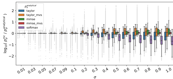
(d) FMNIST, CNN
