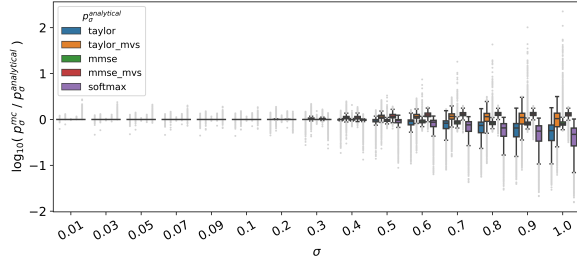
(b) MNIST, CNN
