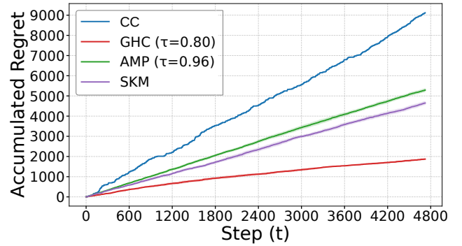
(d) Regret vs. step, Nomic, ComQA.
