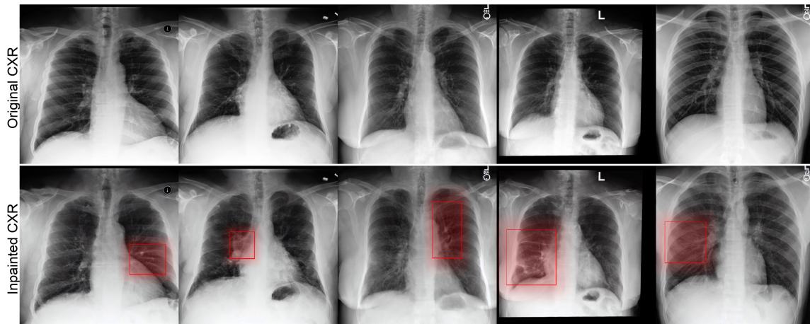
(d) Edema
