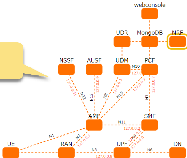
構成図
