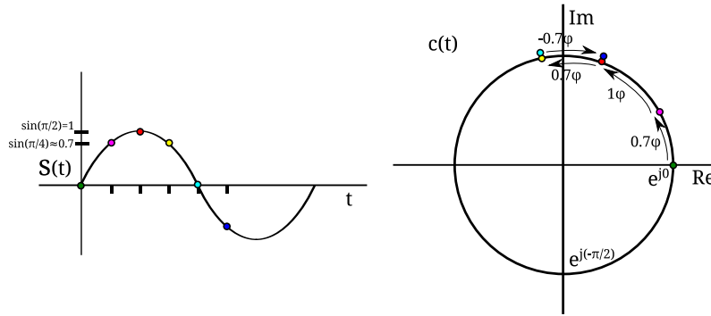
2. ábra. Komplex forgó vektor szinuszos jel esetén
