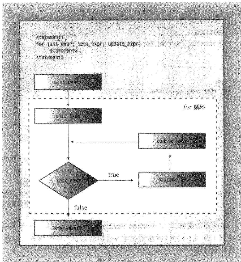
图 5.1 for 循环
