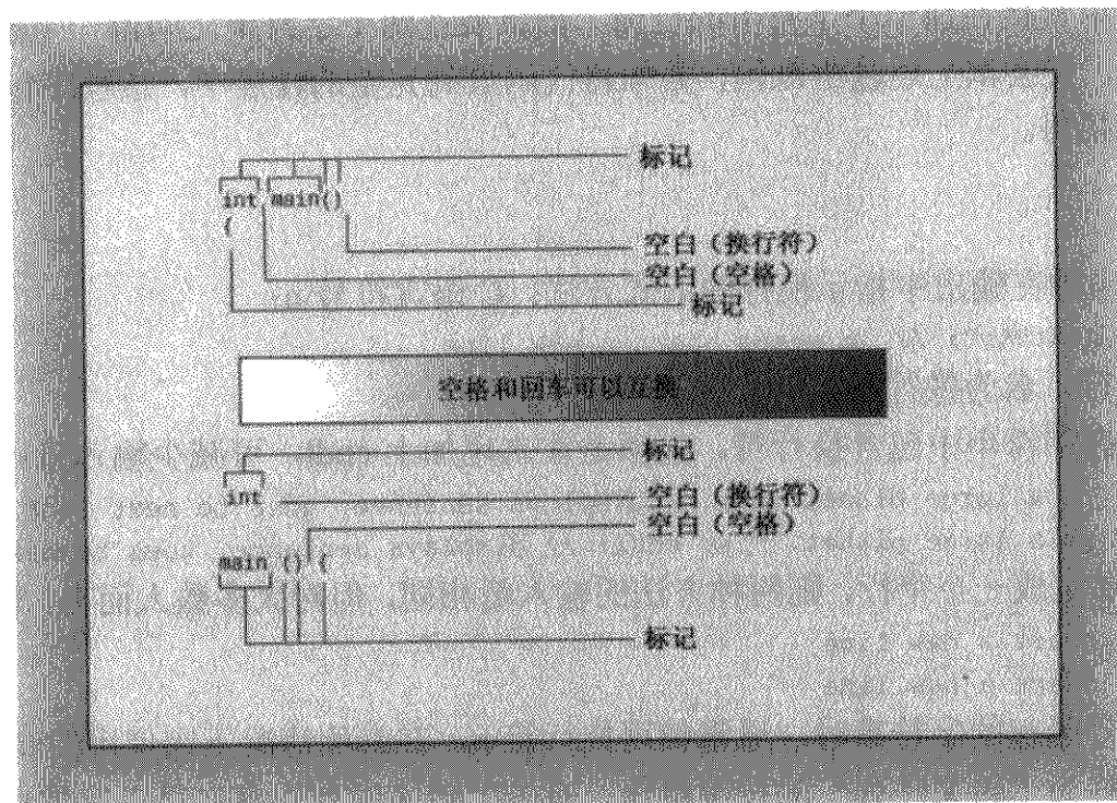
图 2.3 标记和空白
