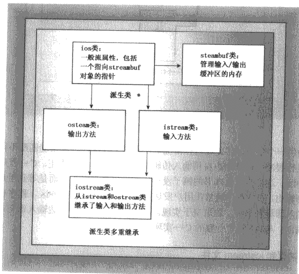
图 17.3 一些 I/O 类
