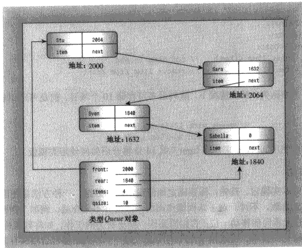
图 12.9 Queue 对象
