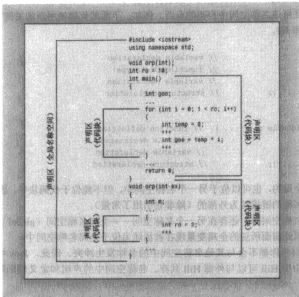
图 9.5 声明区域
