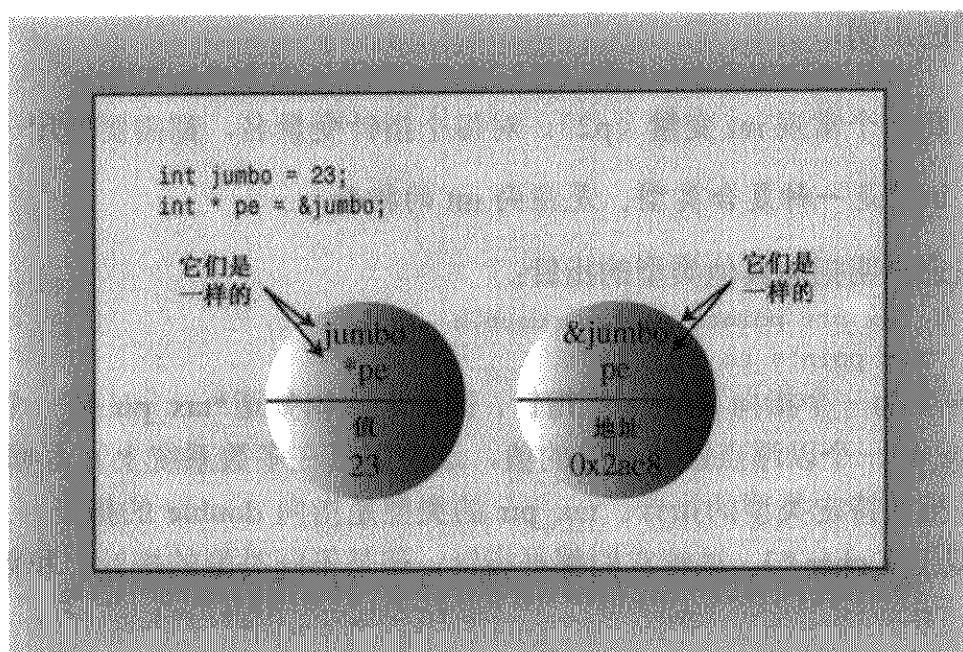
图 4.8 硬币的两面
