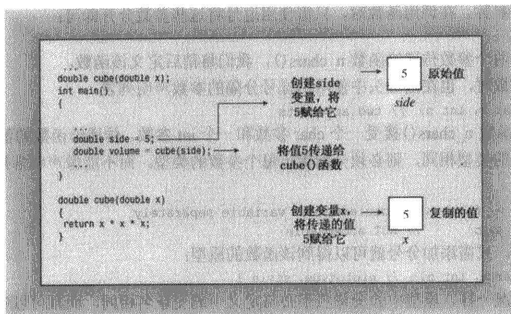
图 7.2 按值传递
