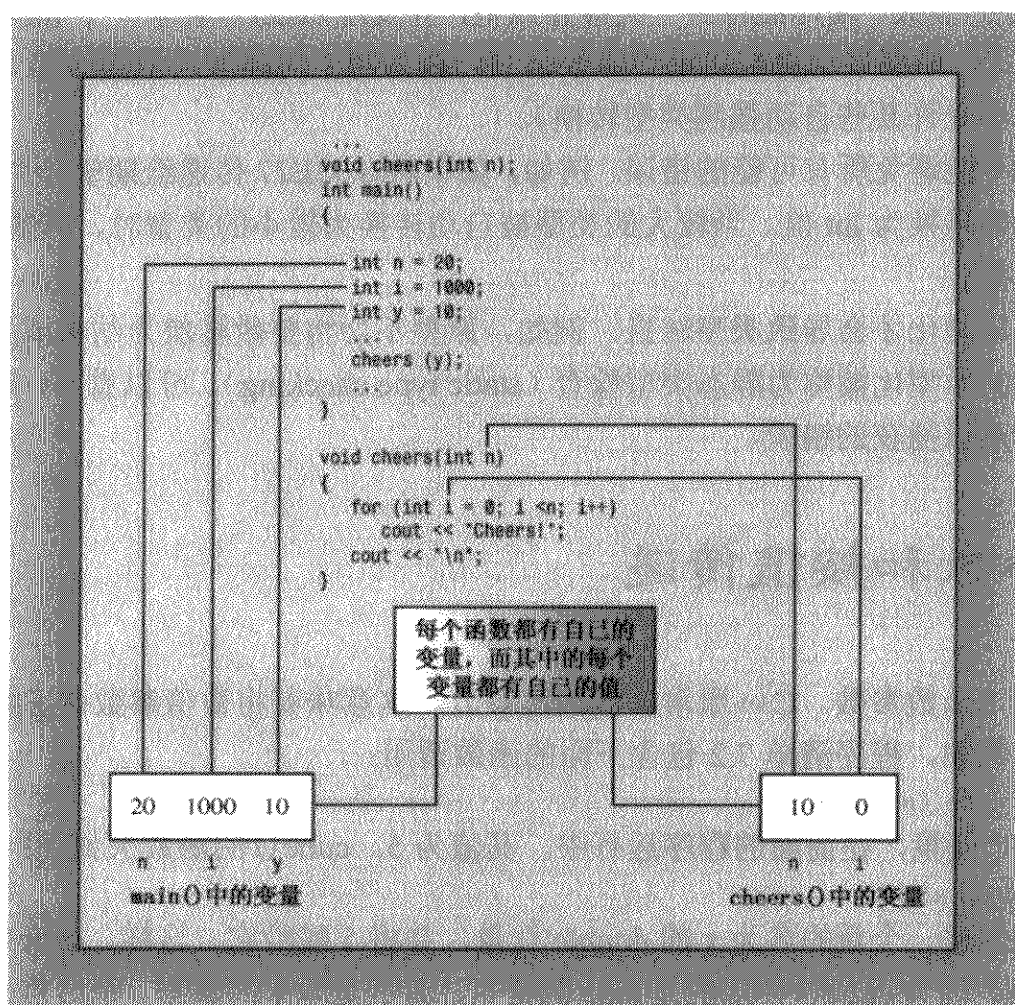
图 7.3 局部变量
