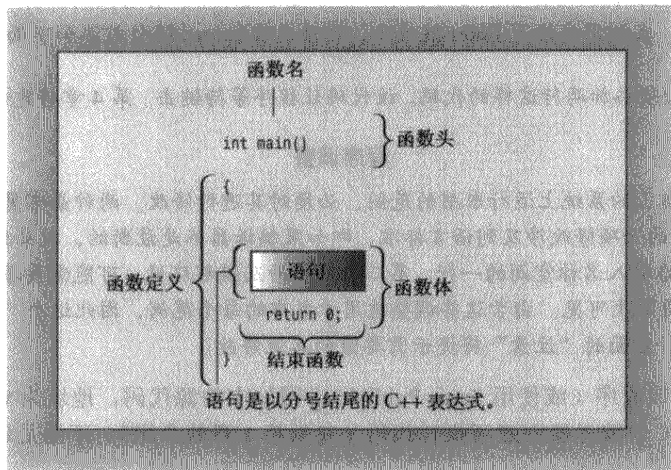
图 2.1 main() 函数
