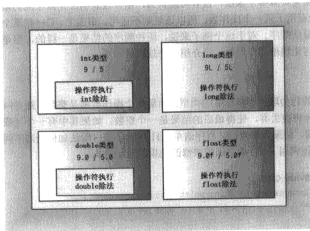
图 3.4 各种除法
