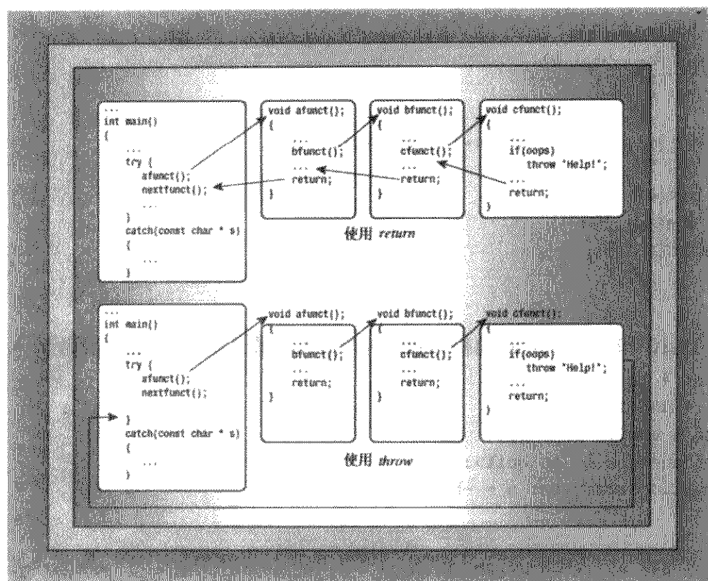
图 15.3 throw 与 return
