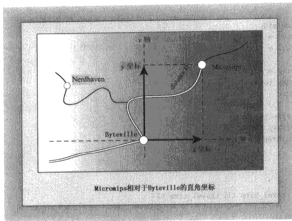
图 7.6 直角坐标
