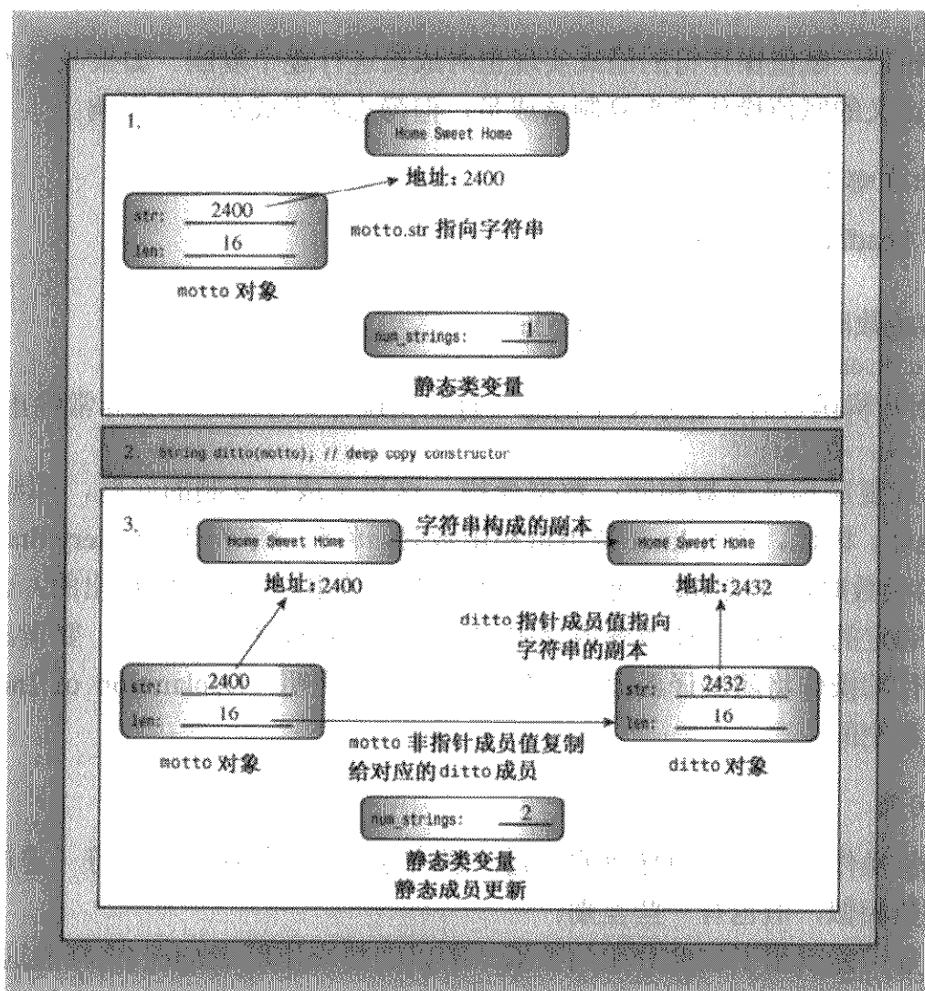
图 12.3 深度复制
