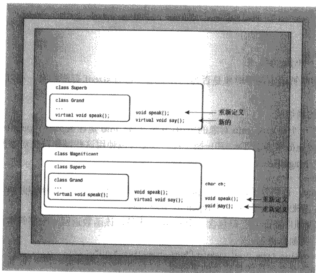
图 15.4 Grand 类系列
