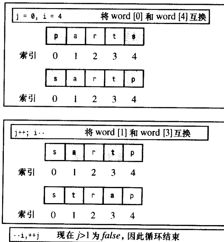
图 5.2 反转字符串
