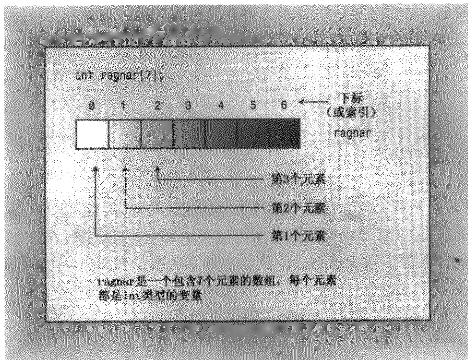
图 4.1 创建数组
