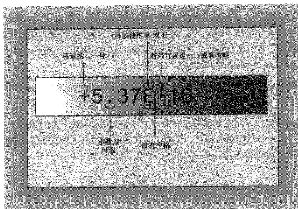
图 3.3 E 表示法
