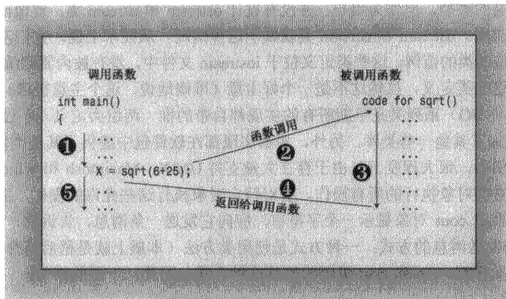
图 2.6 调用函数
