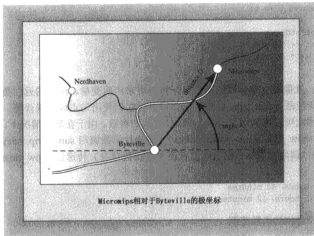
图 7.7 极坐标
