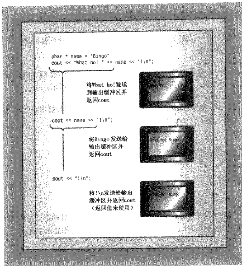
图 17.4 拼接输出
