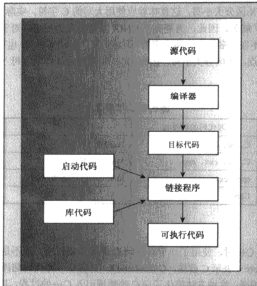
图 1.3 编程步骤
