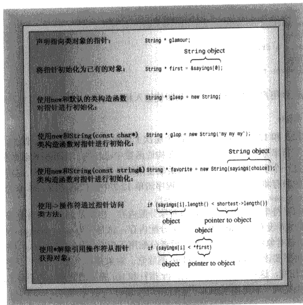
图 12.5 指针和对象
