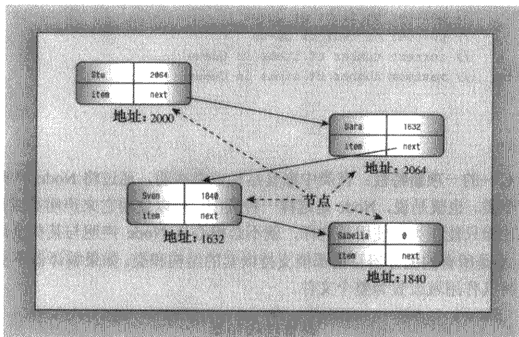
图 12.8 链表
