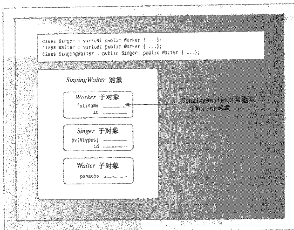
图 14.5 虚基类继承
