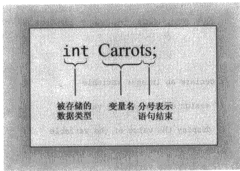
图 2.4 变量声明
