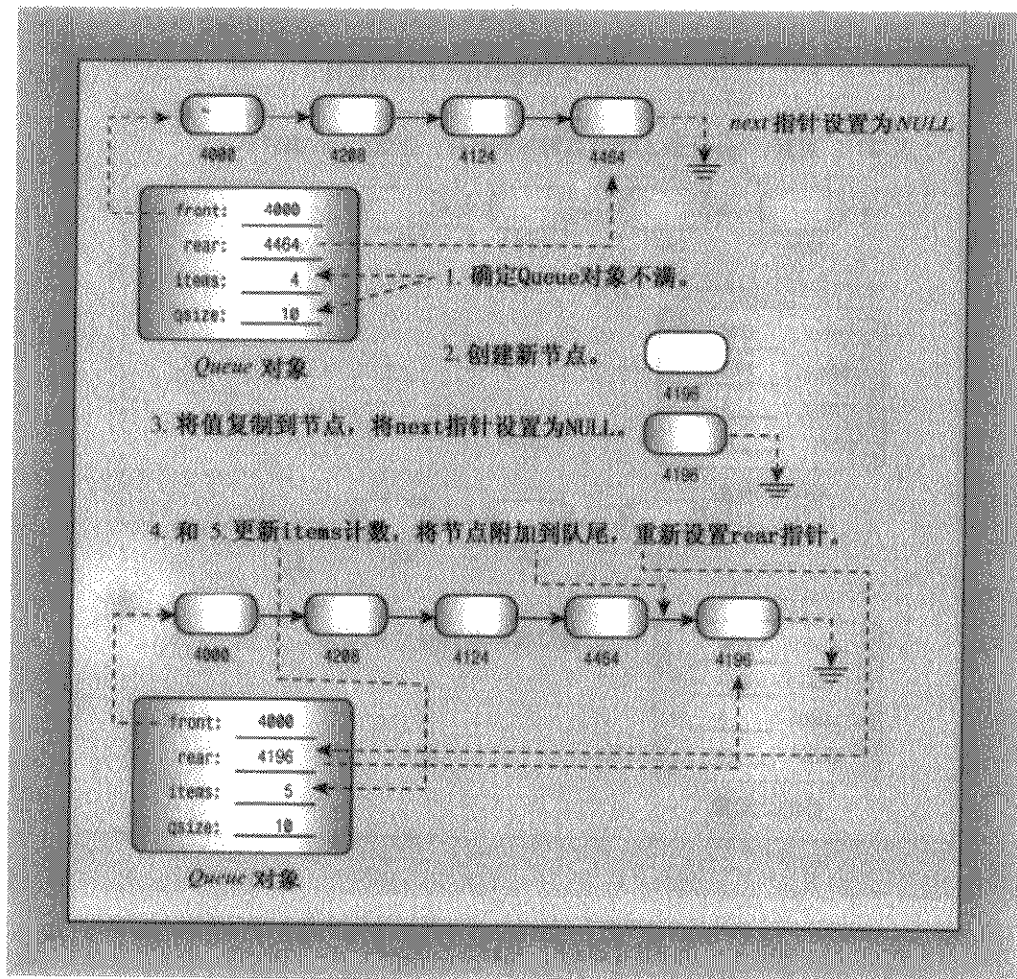
图 12.10 将项目入队
