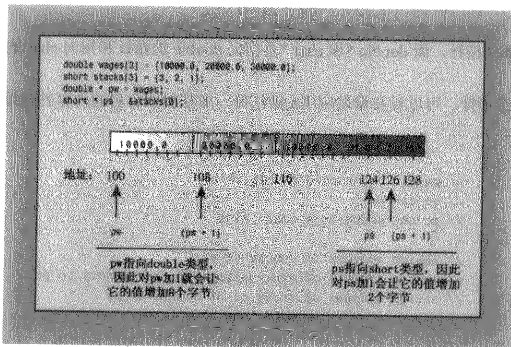
图 4.10 指针加法
