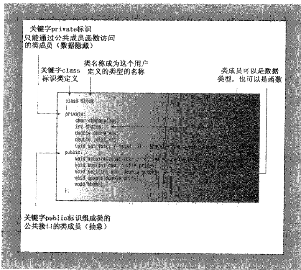
图 10.1 Stock 类
