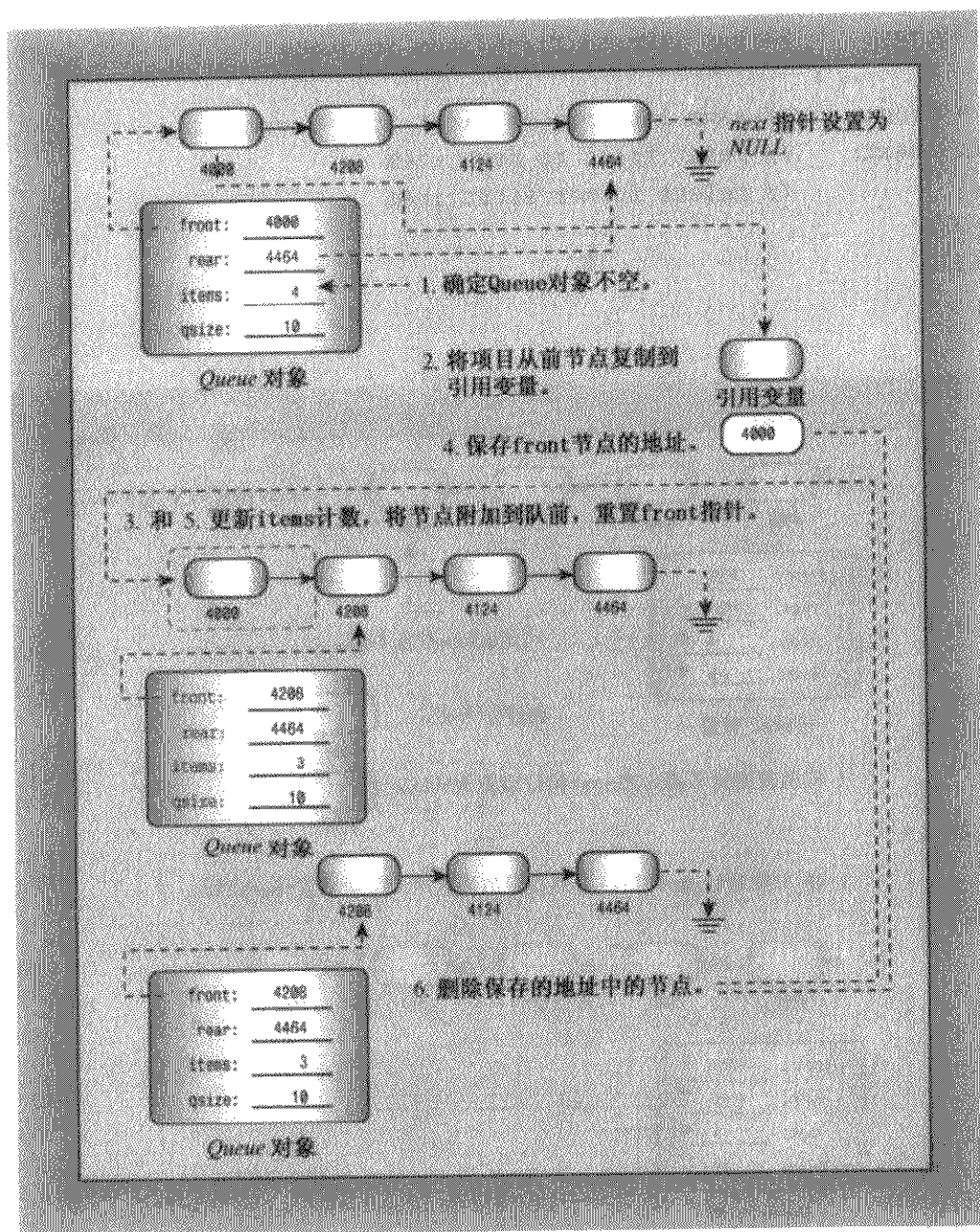
图 12.11 将项目出队
