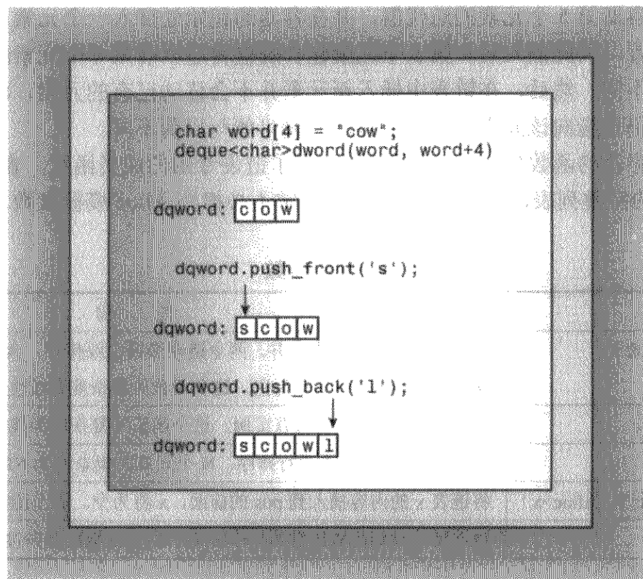
图 16.4 push_front() 和 push_back()
