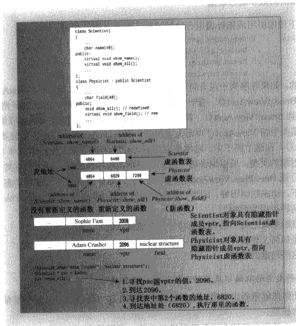
图 13.5 虚函数机制
