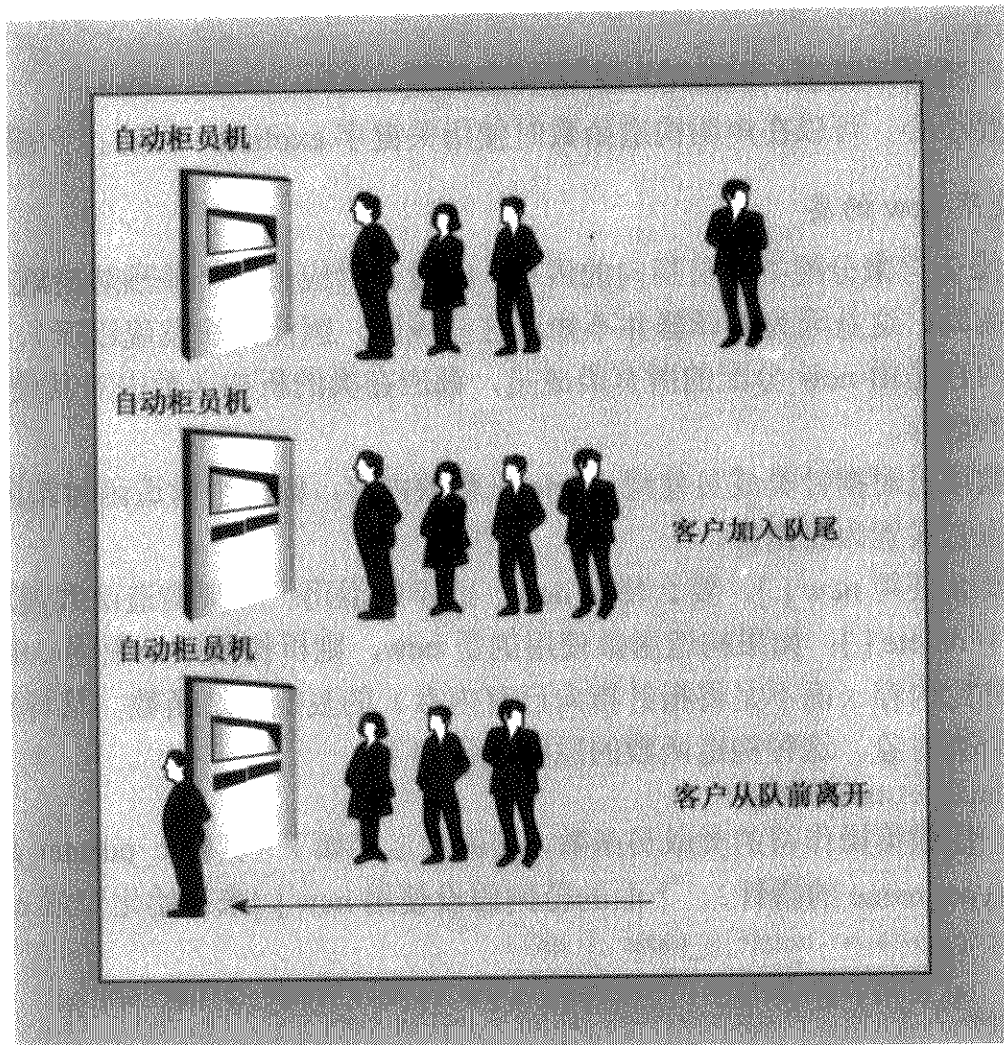
图 12.7 队列
