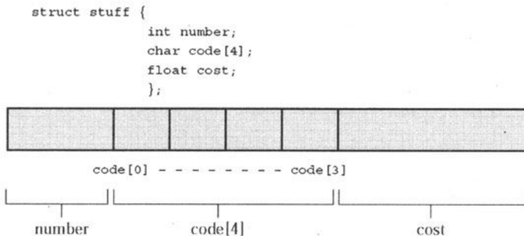
图14.1 结构的存储分配
