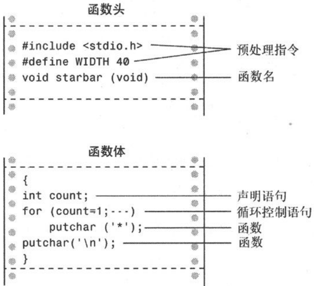
图9.2 一个简单函数的结构
