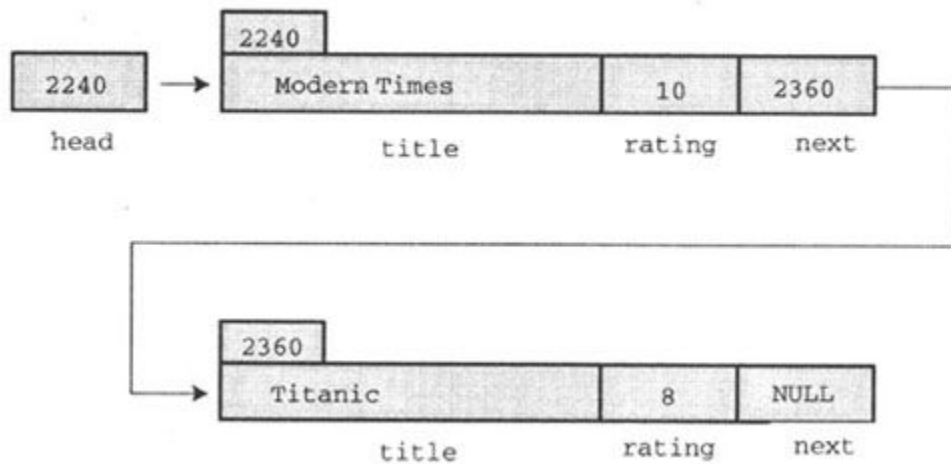
图17.3 含有两个项目的链表
