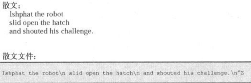
图8.2 具有文件尾标记的文件
