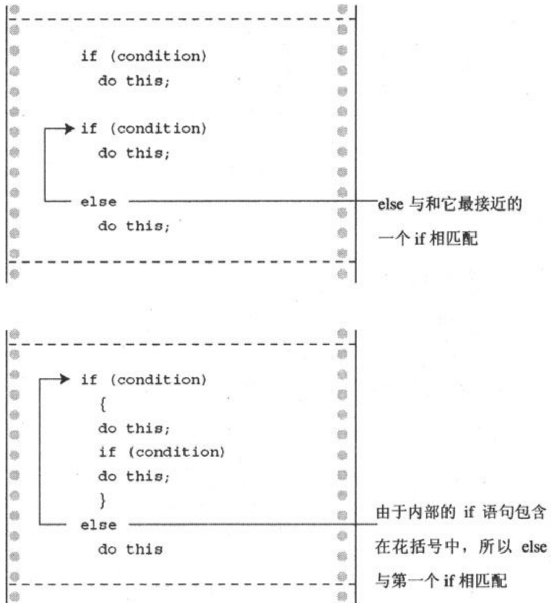
图7.3 if else的配对规则
