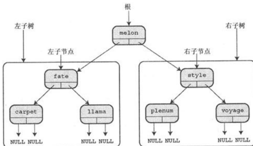
图17.12 一个存储单词的二叉搜索树
