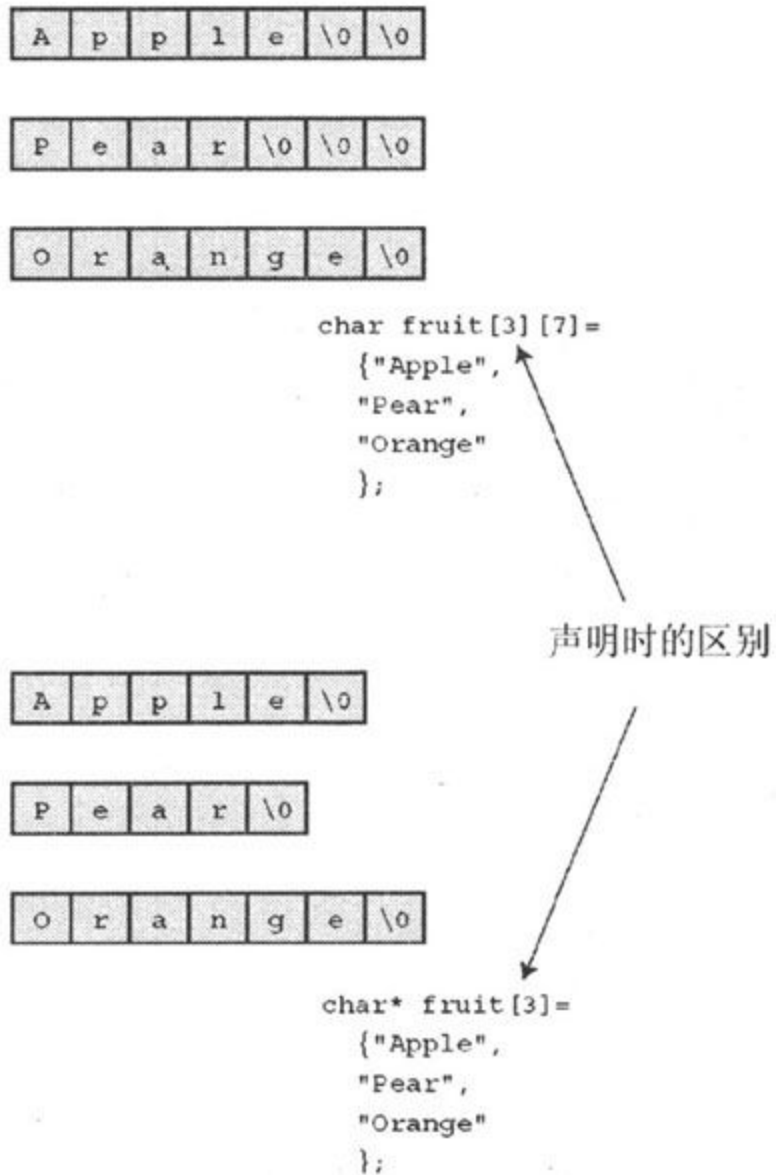
图11.2 矩形数组和不规则数组
