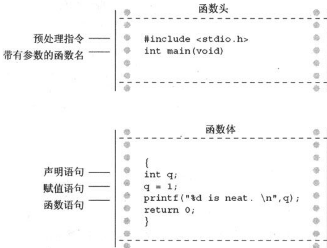
图2.4 一个包含函数头和函数体的函数
