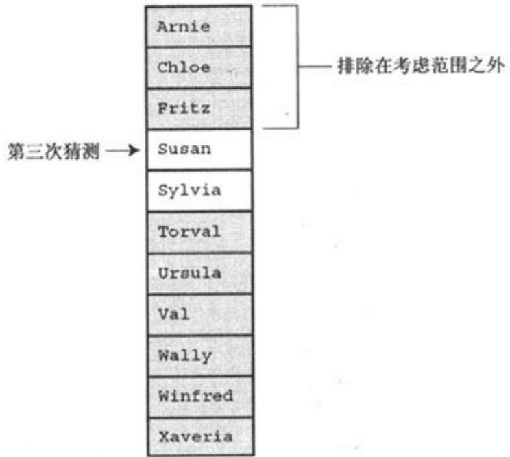
图17.11 以折半搜索法查找Susan
