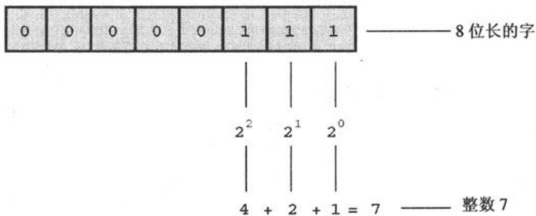
图3.2 使用二进制编码存储整数7
