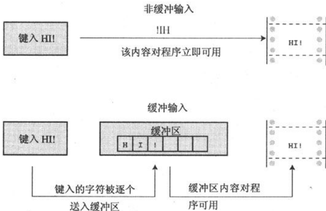
图8.1 缓冲输入与非缓冲输入
