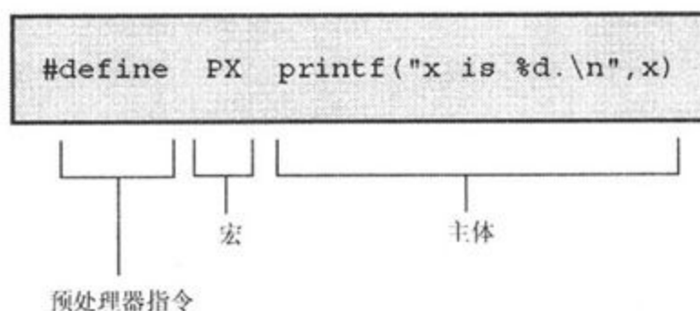
图16.1 类对象宏定义的组成
