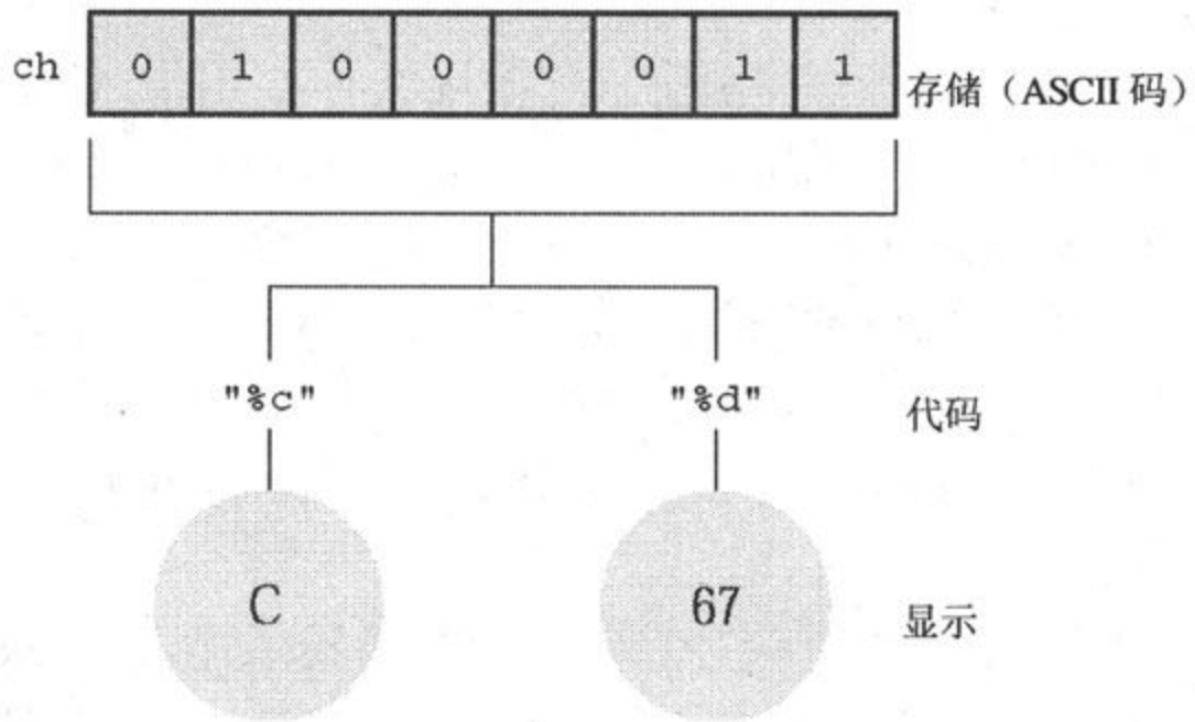
图3.6 数据显示与数据存储
