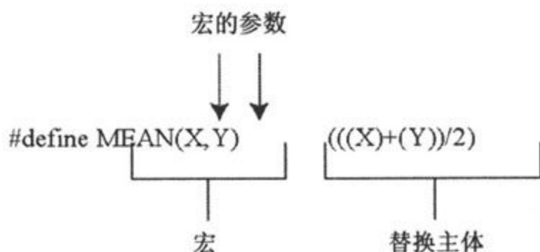
图16.2 类型函数宏定义的组成
