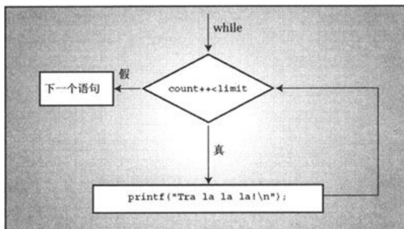
图6.1 while循环的结构
