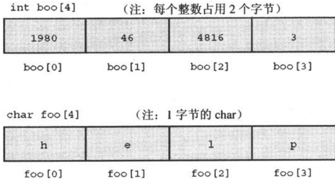
图6.7 内存中的char和int数组
