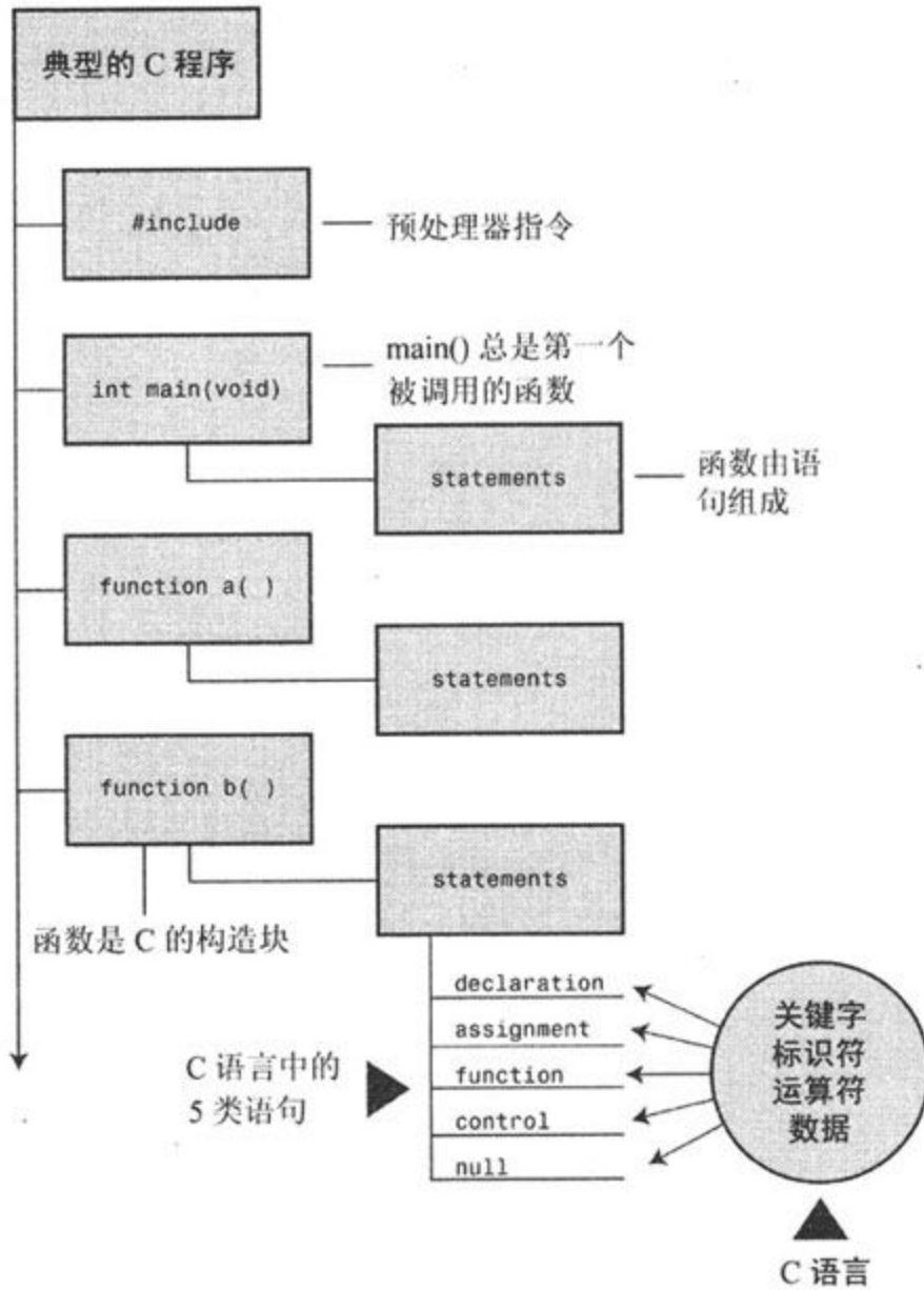
图2.1 C程序剖析
