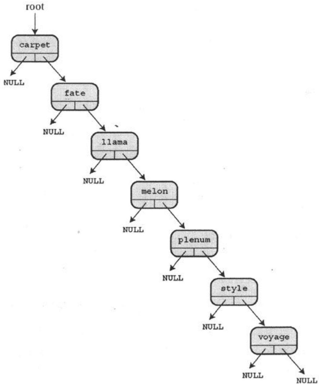
图17.16 不平衡的二叉搜索树
