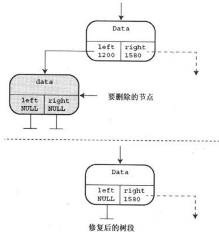
图17.13 删除一个叶节点
