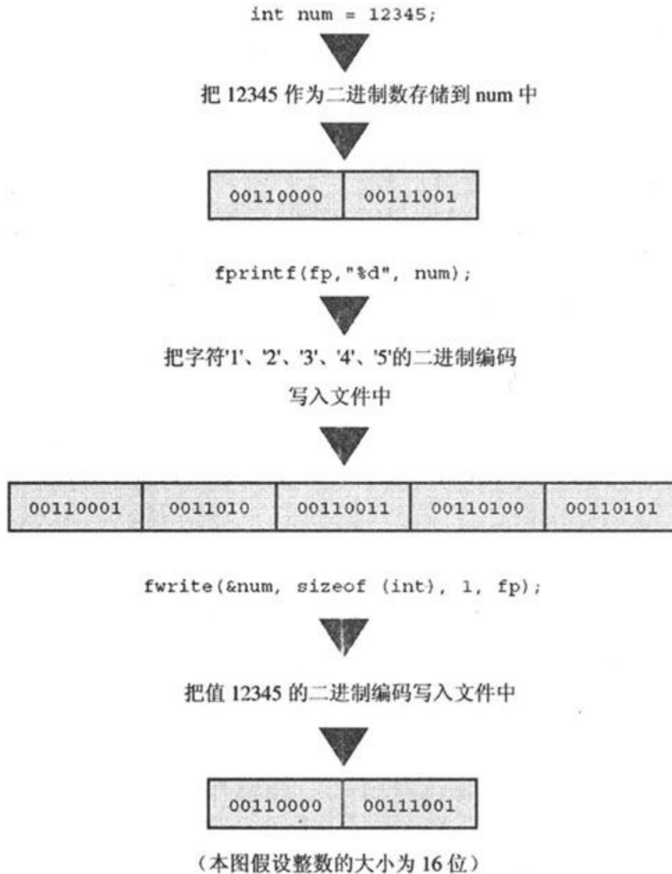
图13.3 二进制输出和文本输出
