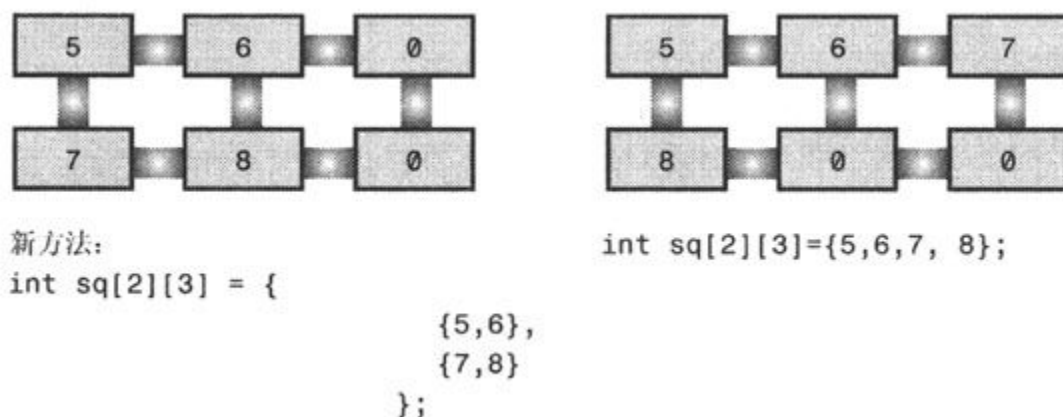
图10.2 初始化数组的两种方法
