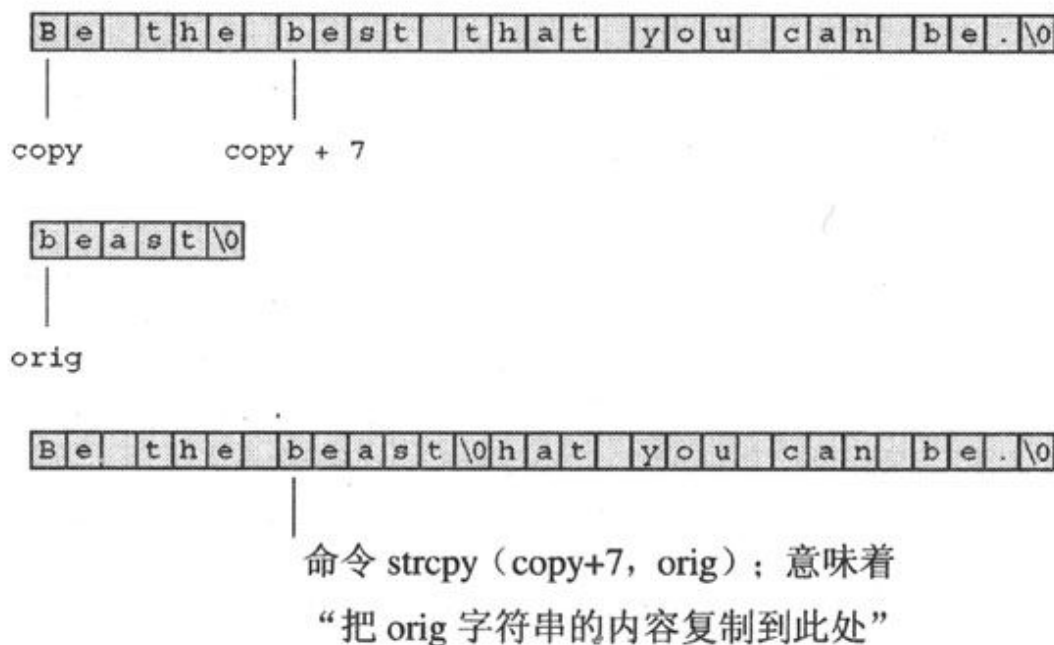
图11.5 strcpy() 使用指针
