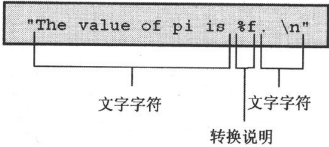
图4.7 一个控制字符串的结构
