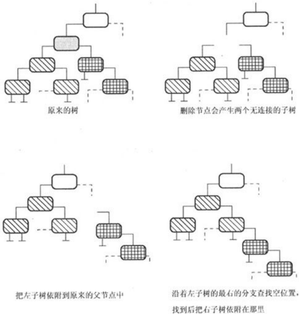
图17.15 删除有两个子节点的节点
