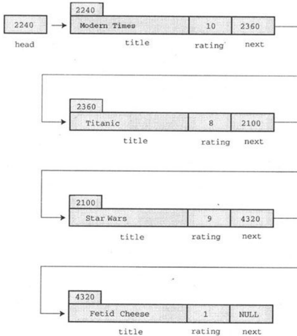
图17.4 含有多个项目的链表
