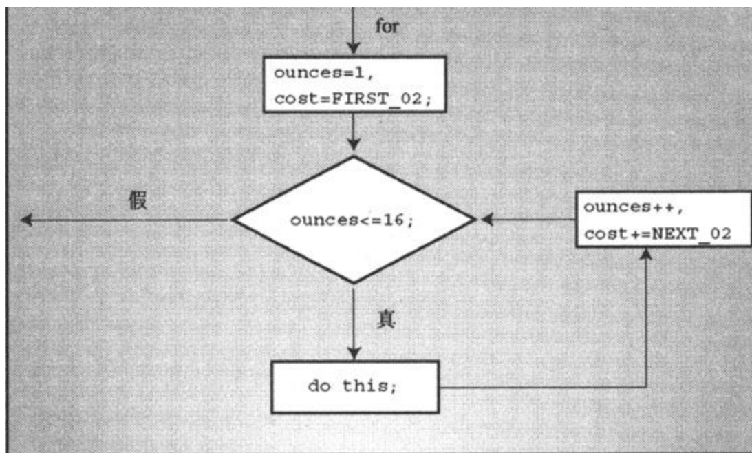
图6.4 逗号运算符和for循环
