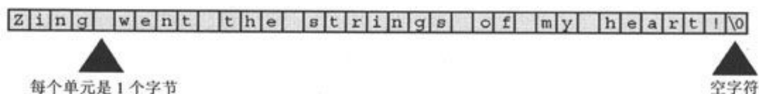
图4.1 字符串在数组中的存储
