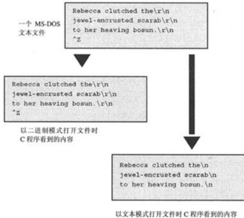
图13.1 二进制视图和文本视图
