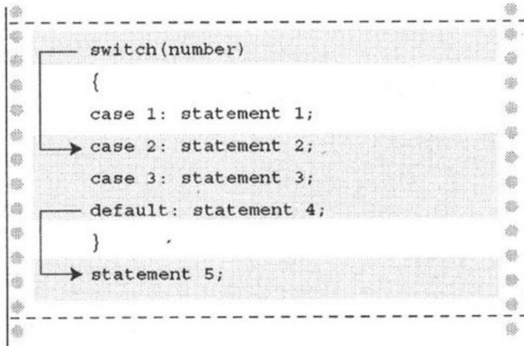
图7.5 switch语句中有和没有break时的程序流程
