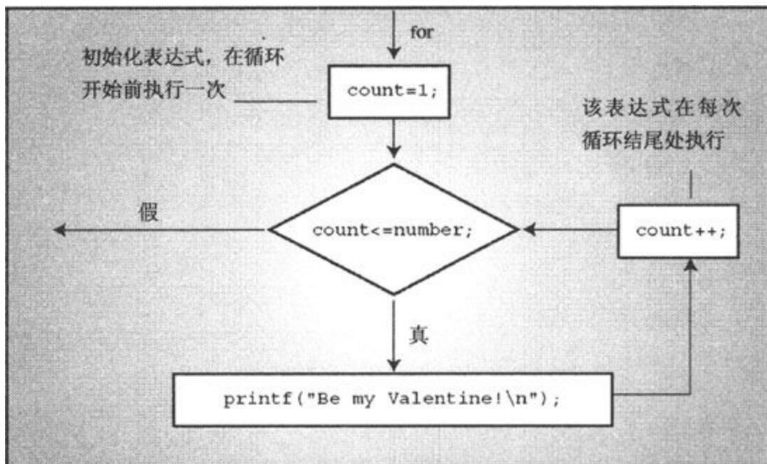
图6.3 for循环的结构
