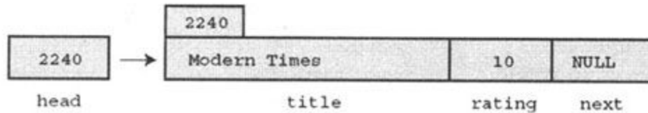
图17.2 链表中的第一项
