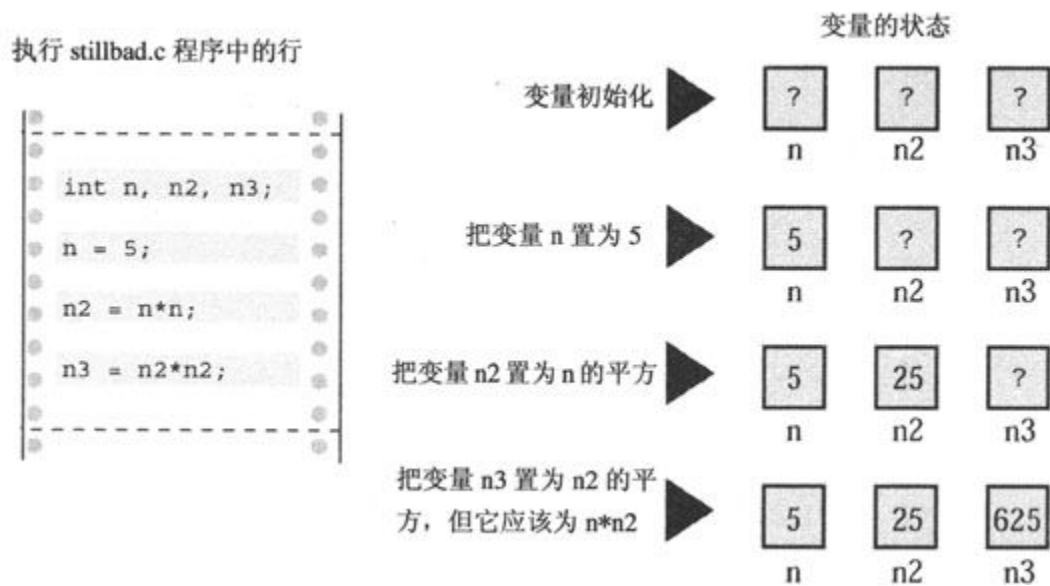
图2.6 跟踪一个程序
