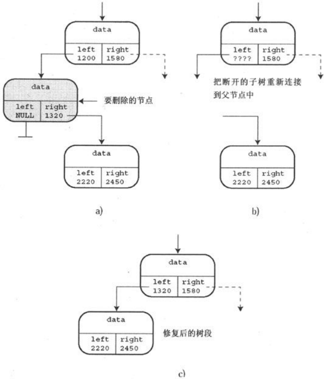
图17.14 删除有一个子节点的节点
