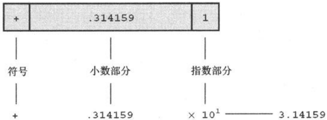
图3.3 以浮点格式存储实数（十进制版本）
