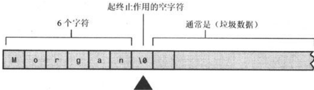
图4.4 strlen（）函数知道在哪里停止
