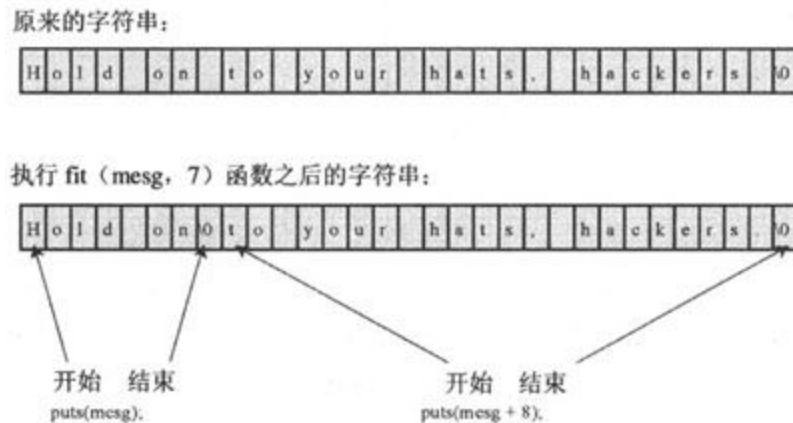
图 11.4 puts ( ) 和空字符
