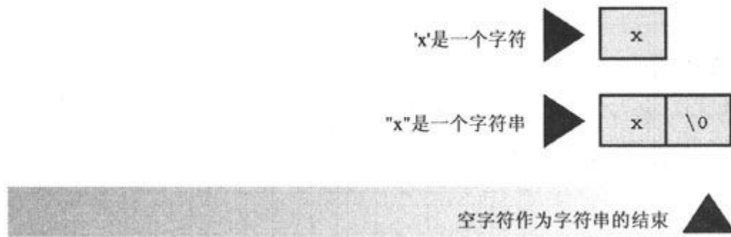
图4.3 字符‘x’和字符串“x”
