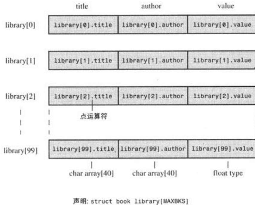
图14.2 一个结构数组
