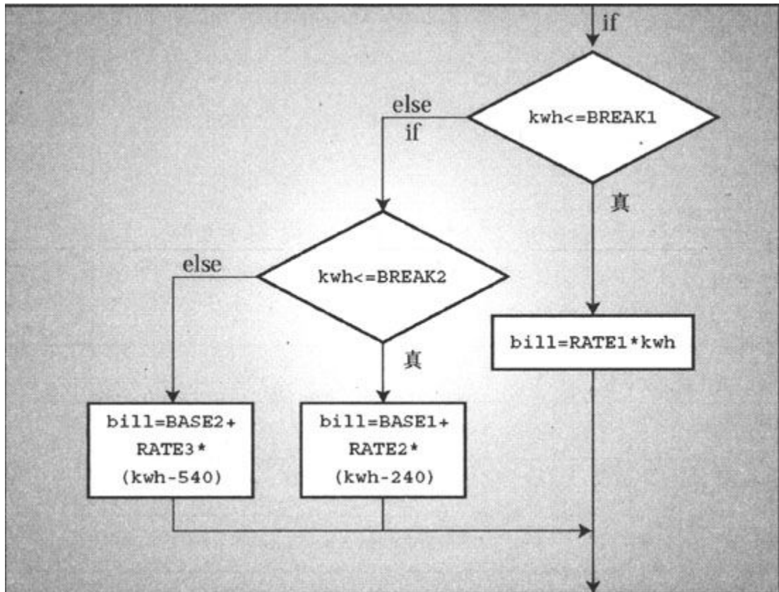
图7.2 程序清单7.4 (electric.c) 的程序流程
