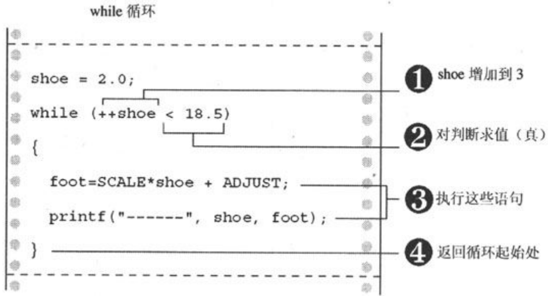
图5.4 通过循环一次
