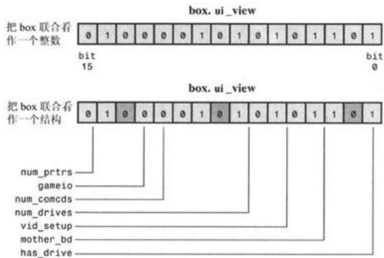
图15.3 整数和结构的联合
