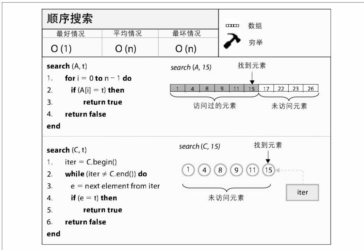
图 5-1 顺序查找详解
