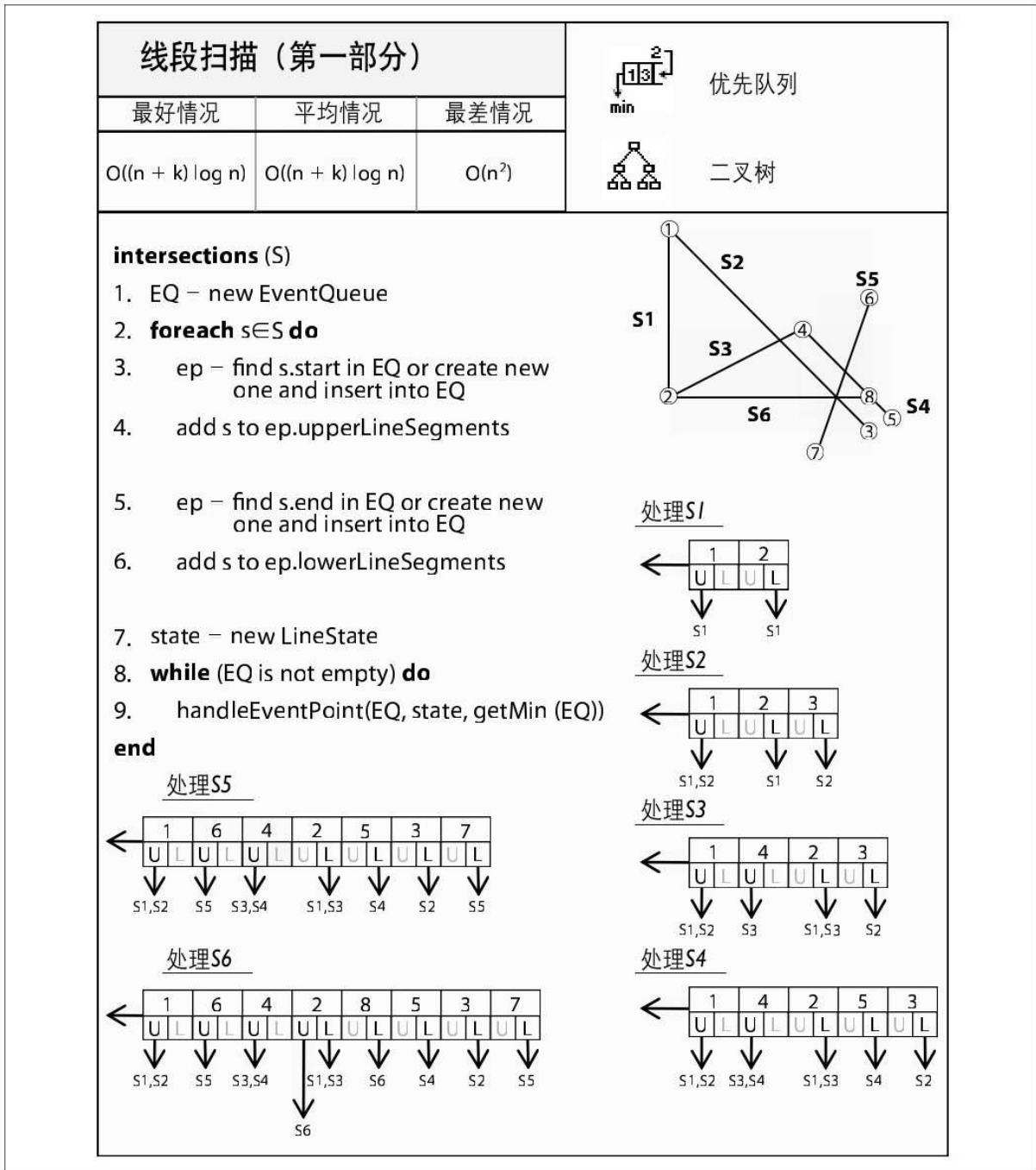
图 9-14 线段扫描算法详解 (第一部分)
