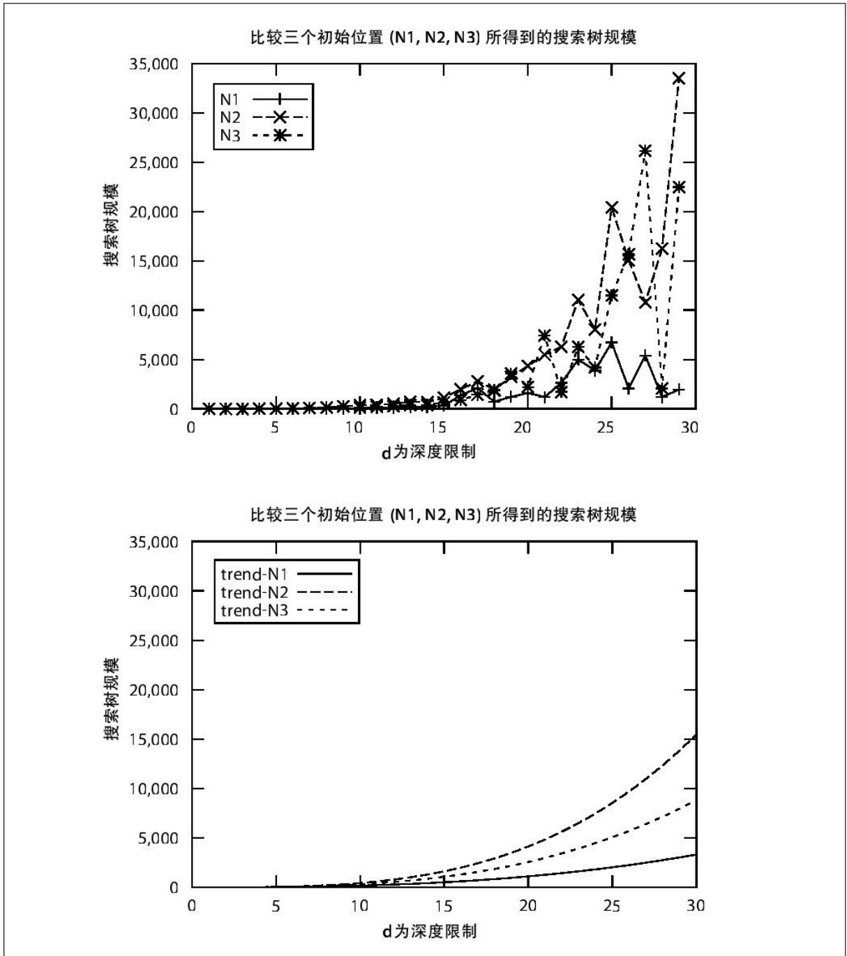
图 7-7 随着深度增加，深度优先搜索搜索树的规模
