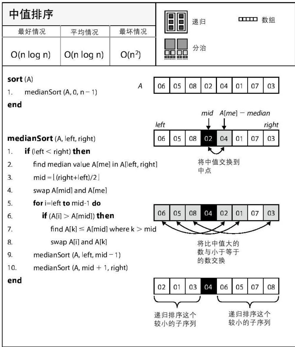
图 4-8 中值排序详解
