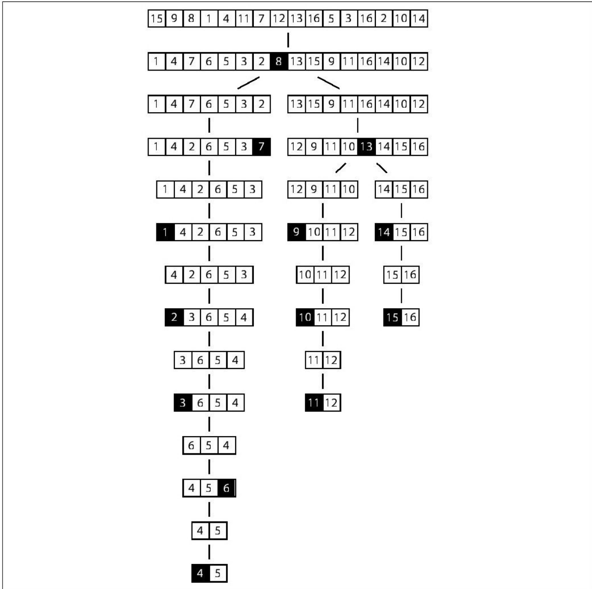
图 4-13 快速排序的不同行为
