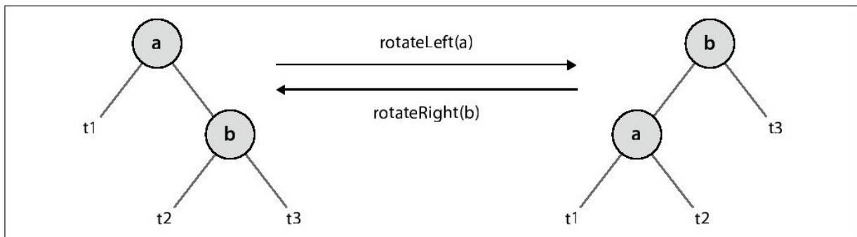
图 5-12 红黑节点旋转
