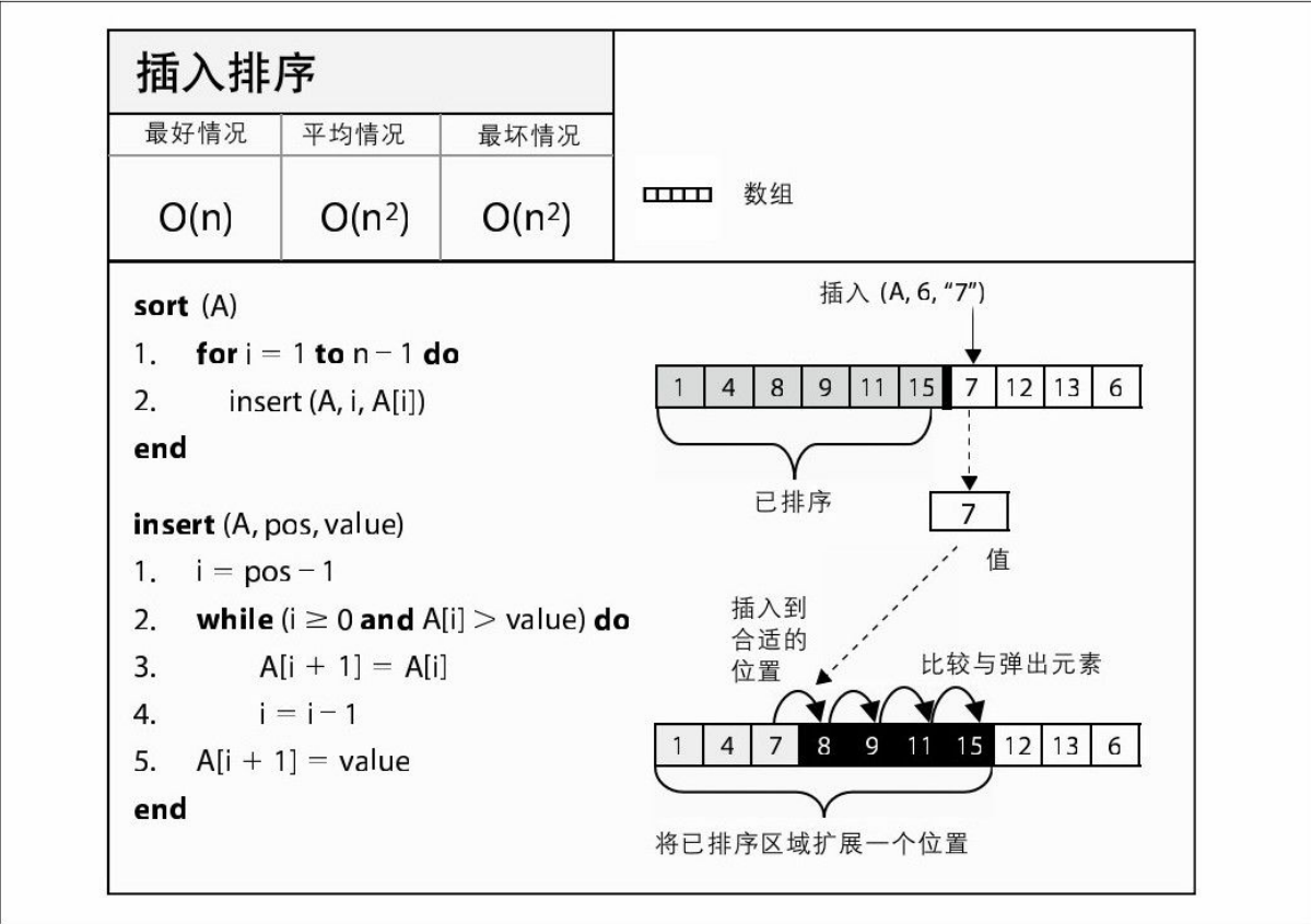
图 4-6 插入排序详解
