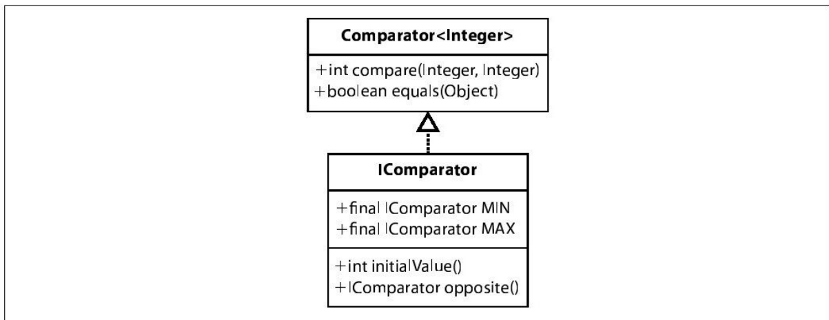
图 7-16 IComparator接口重载了MAX和MIN操作符
