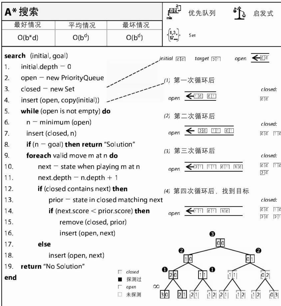
图 7-10 A*搜索详解
