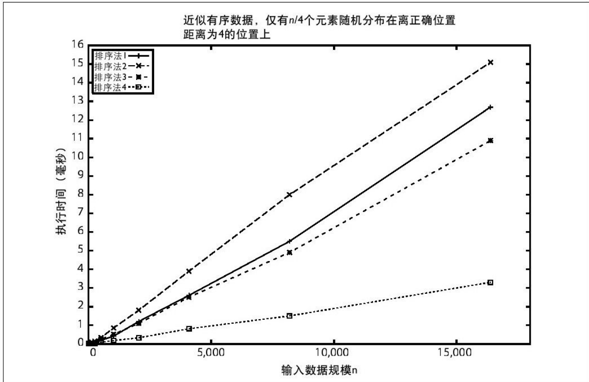
图 2-4 处理几乎有序数据时，第四种排序法胜出
