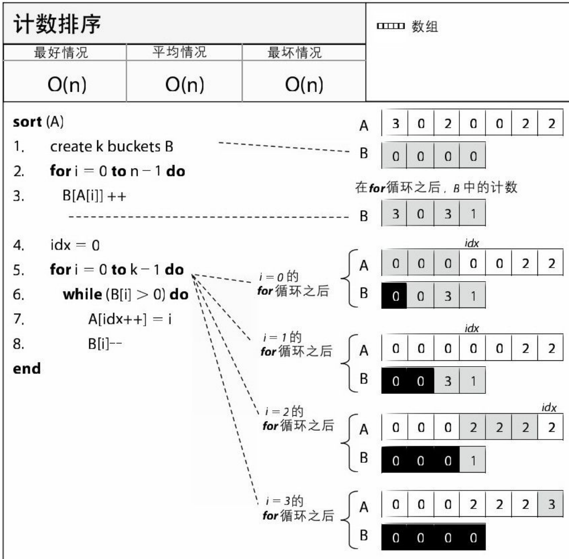
图 4-17 计数排序详解
