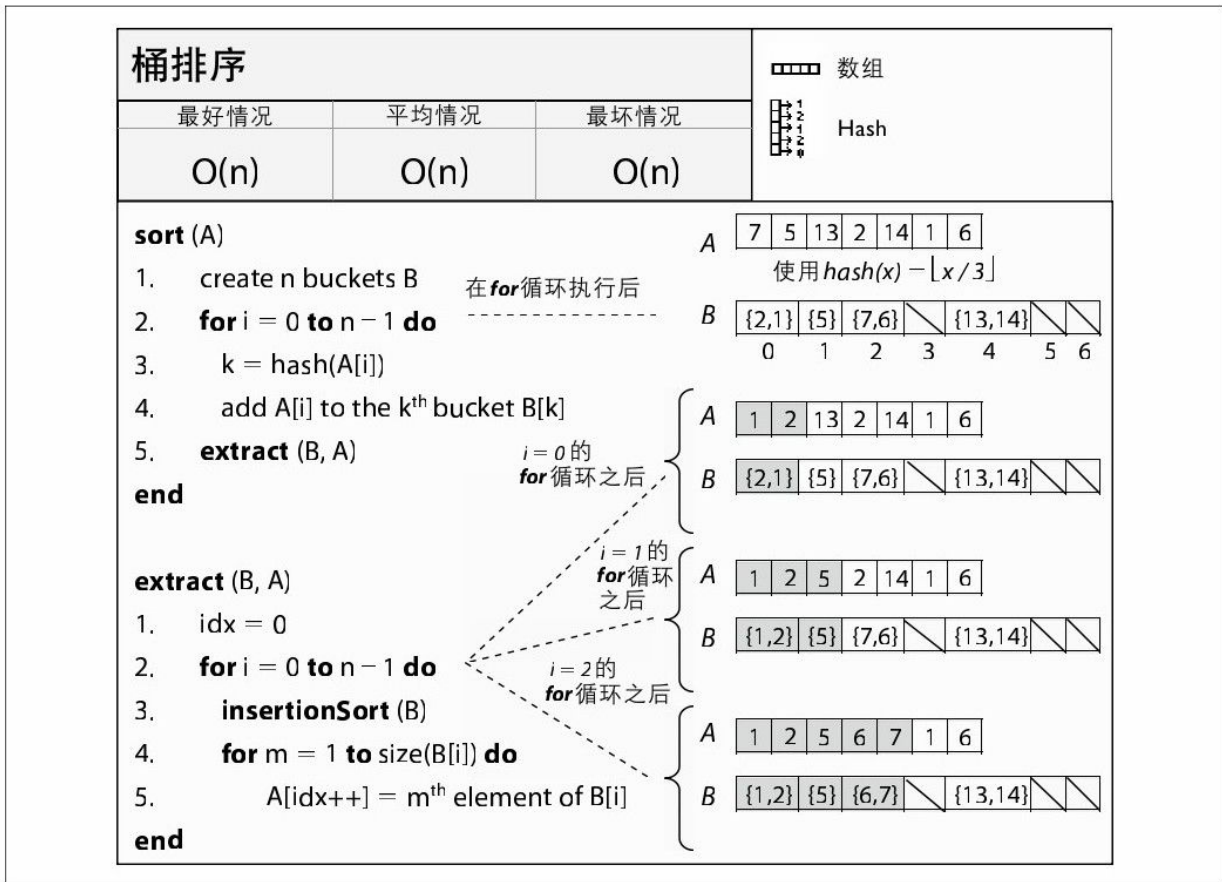
图 4-18 桶排序详细介绍
