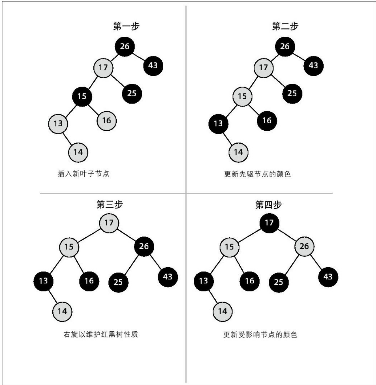
图 5-11 添加键值14的元素到红黑树所需要的4步
