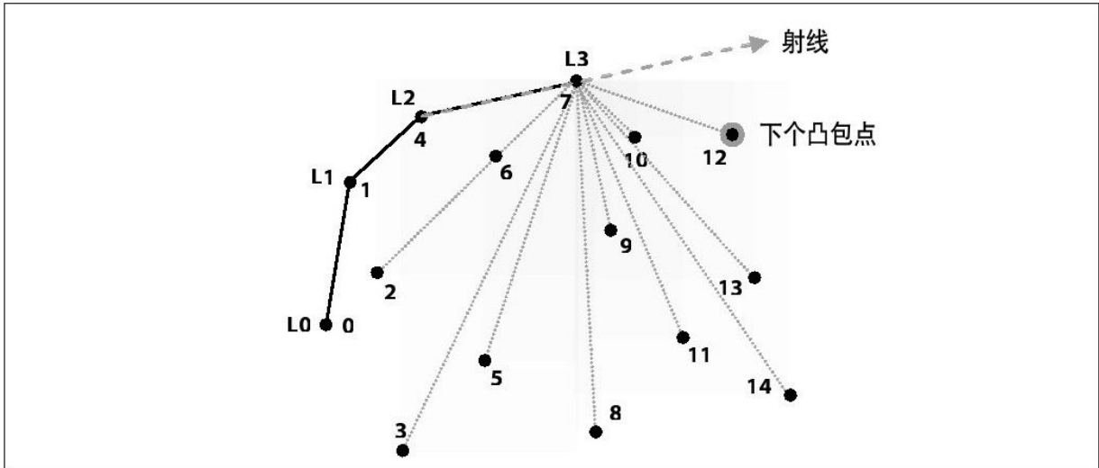
图 9-8 凸包的增量式构建
