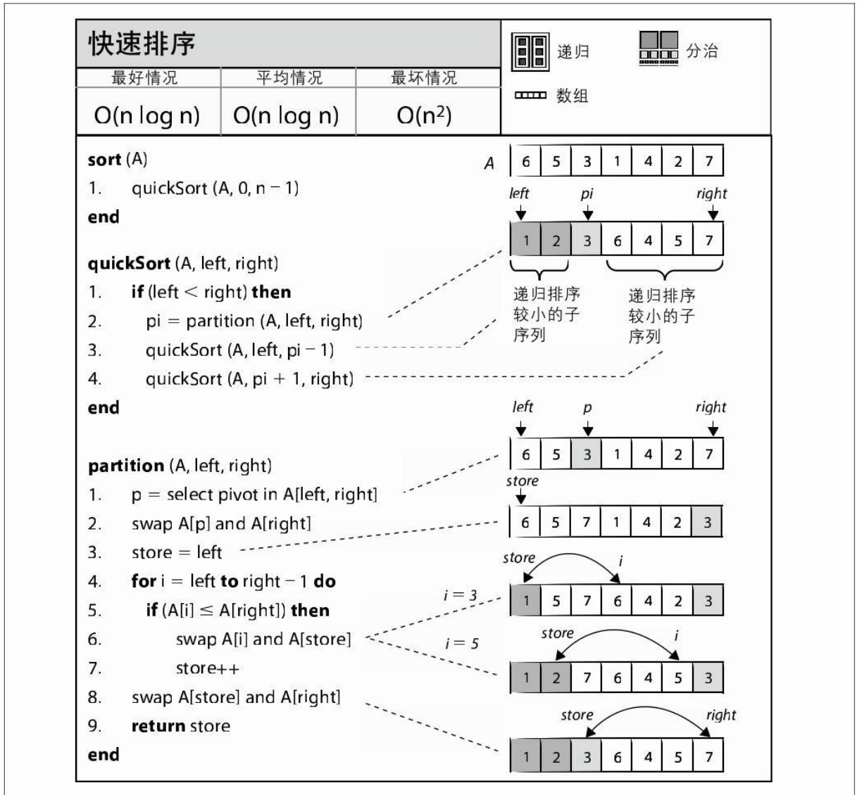
图 4-11 快速排序详解
