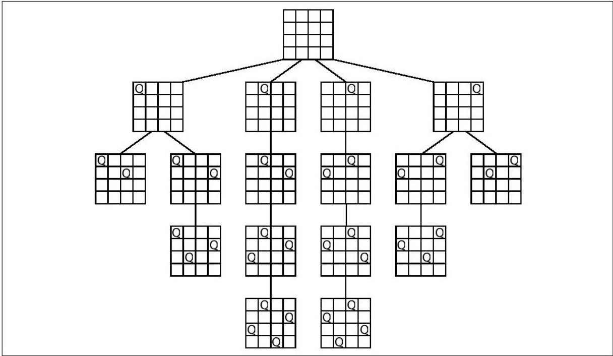
图 10-3 4皇后问题的最终解
