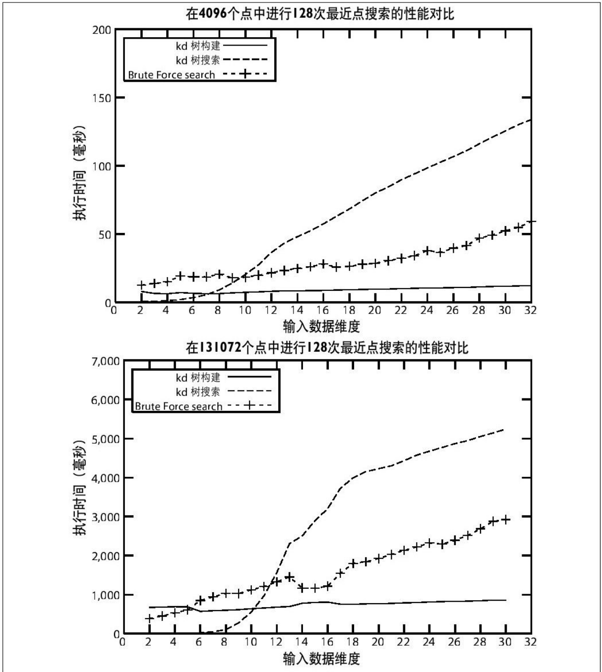
图 9-23 比较kd树和穷举实现
