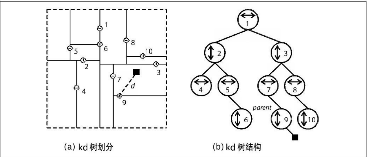
图 9-19 使用kd树切分二维平面
