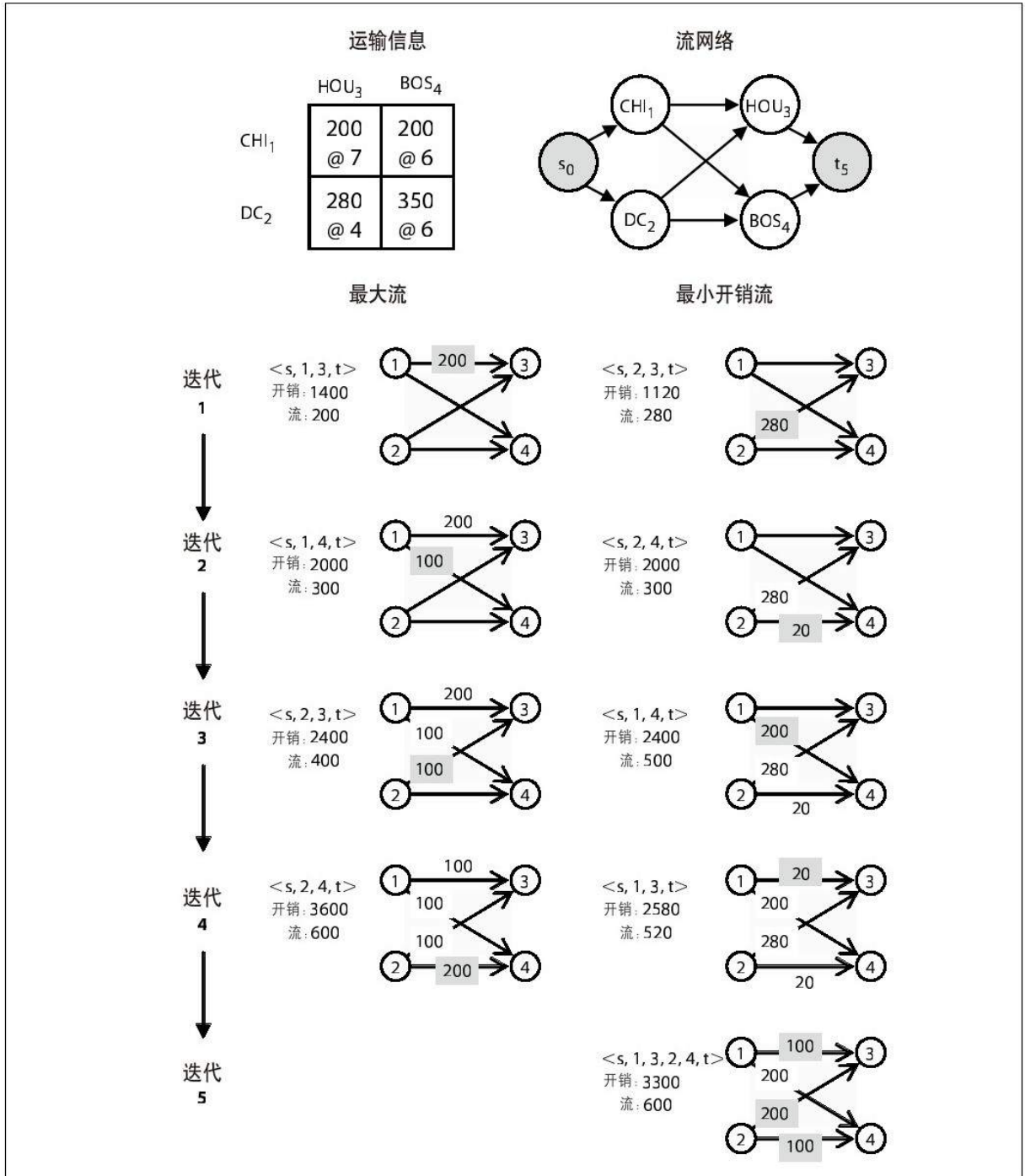
图 8-7 揭示最小开销搜索策略的高效
