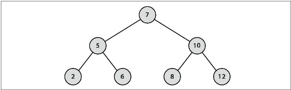
图 5-8 一棵简单的二叉查找树
