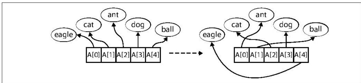
图 4-2 使用指针排序
