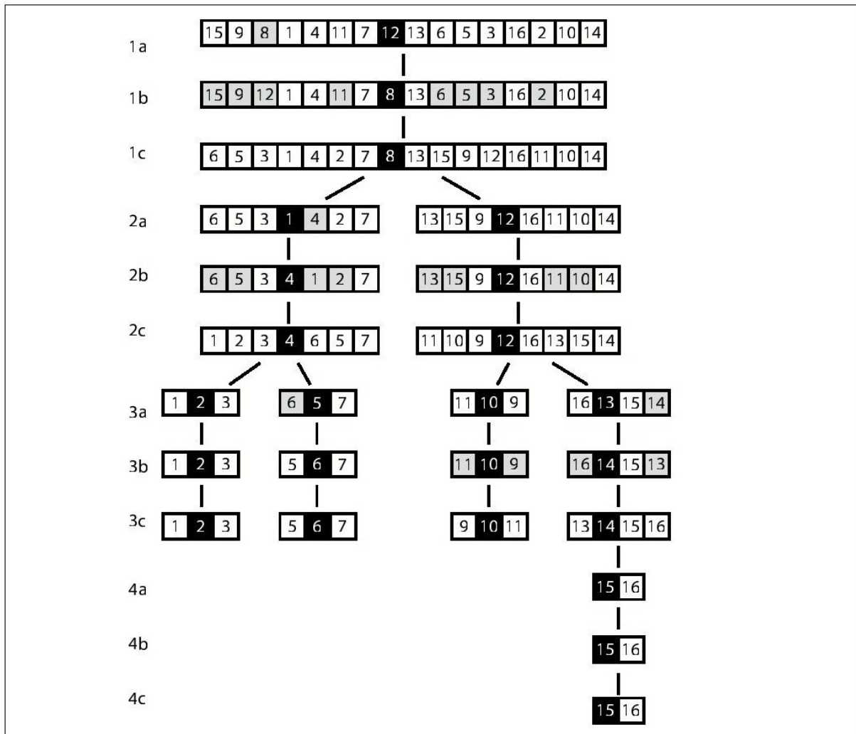
图 4-9 在一个小数组上进行中值排序
