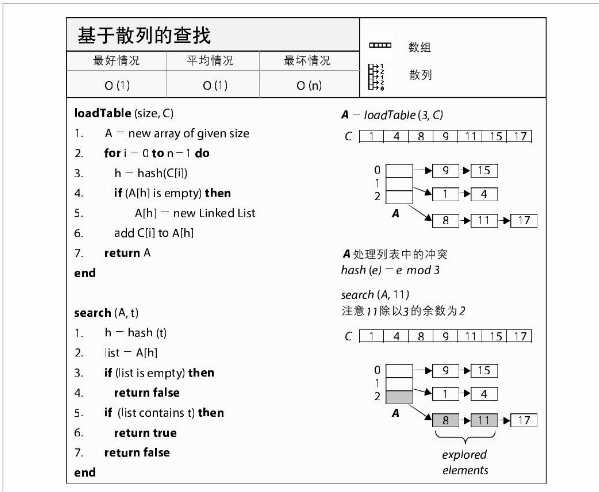
图 5-3 基于散列查找详解
