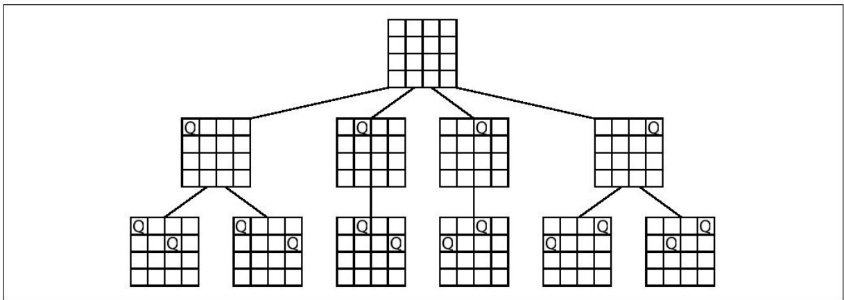
图 10-2 放置了第二个皇后的4皇后搜索树
