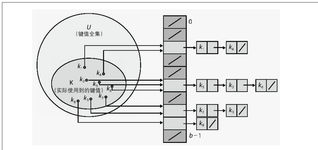
图 5-6 使用表结构来处理冲突
