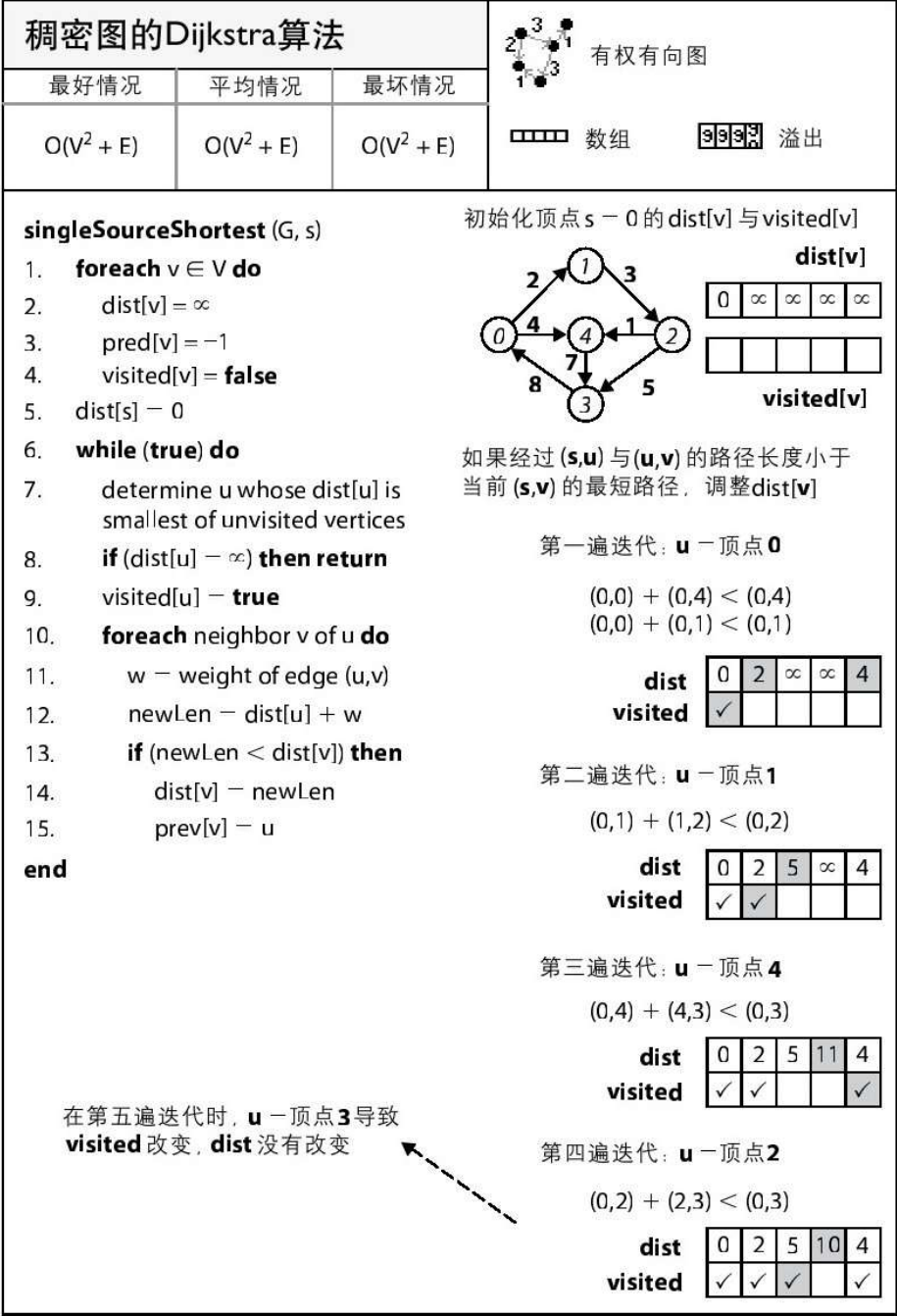
图 6-15 稠密图的Dijkstra算法详解
