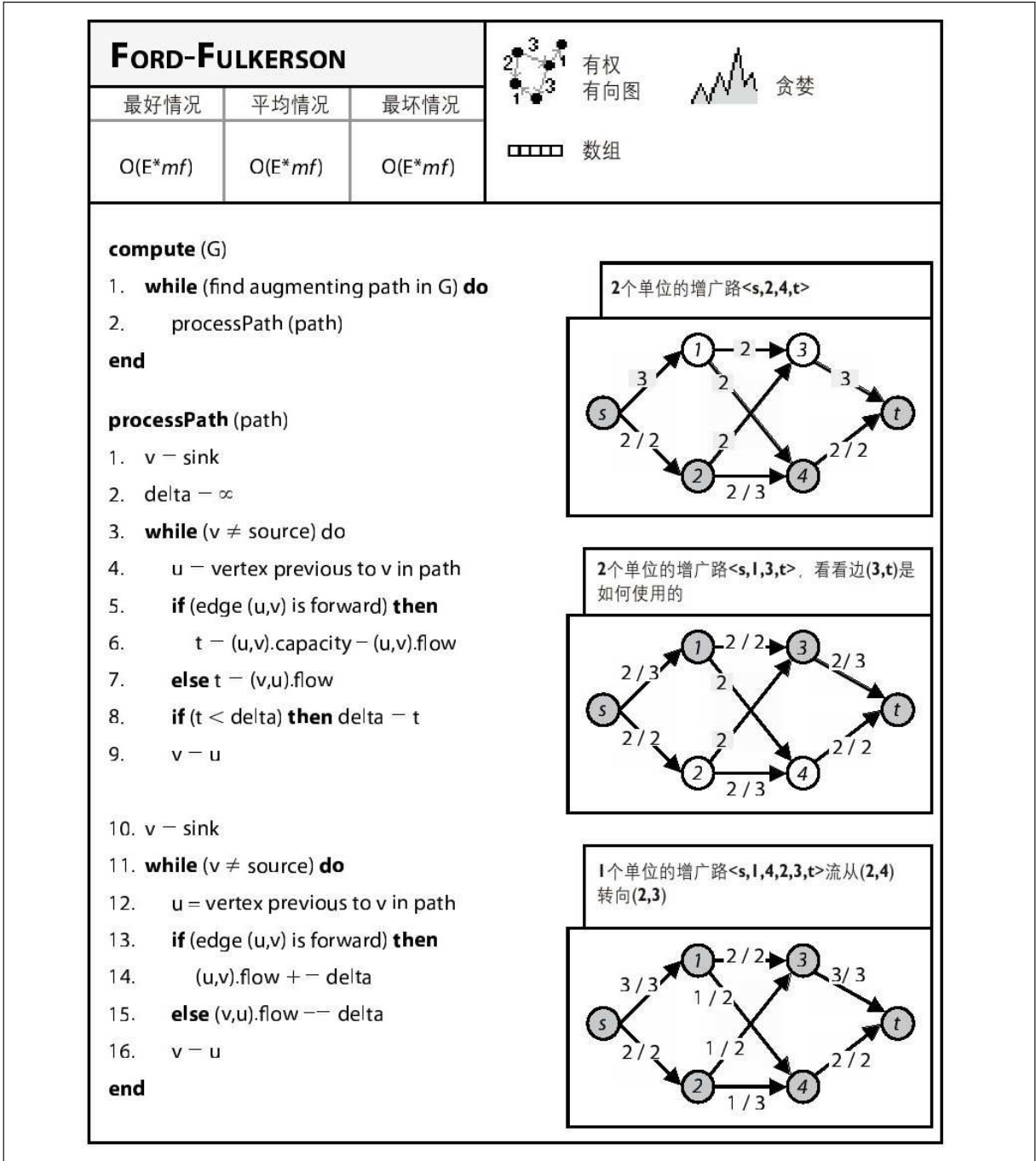
图 8-3 Ford-Fulkerson详解
