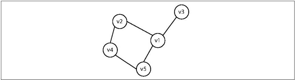
图 6-5 无向图样例
