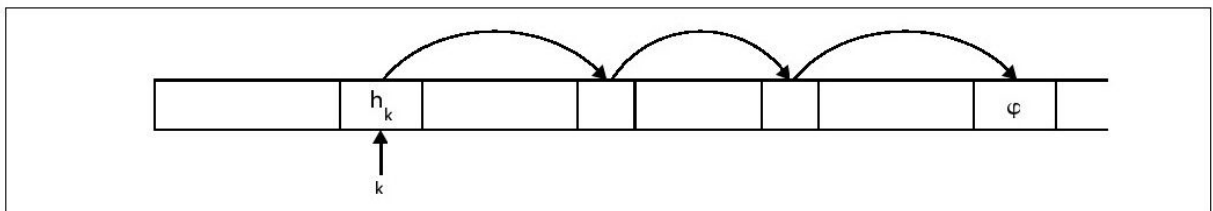
图 5-7 开放定址
