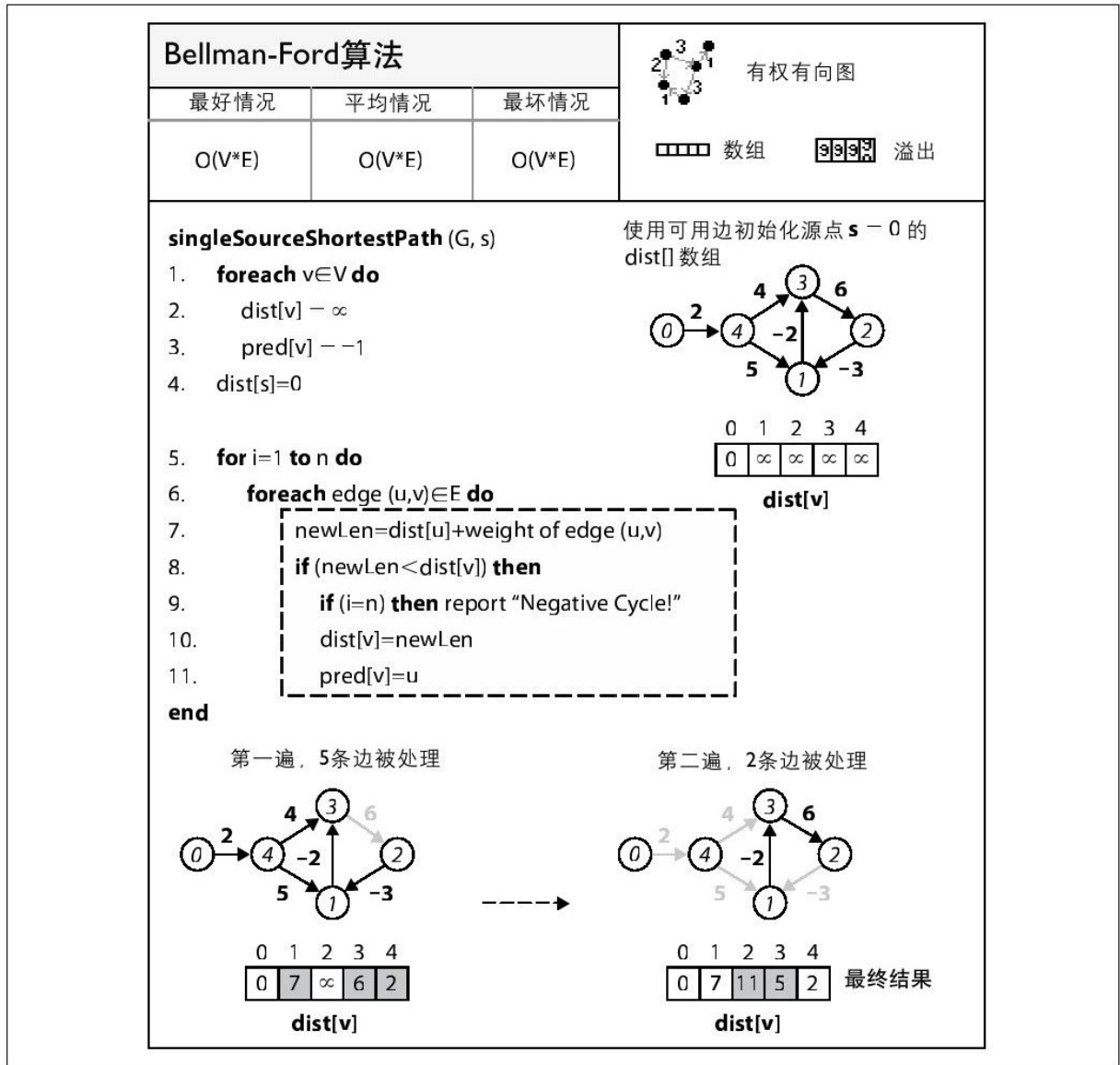
图 6-16 Bellman-Ford详解
