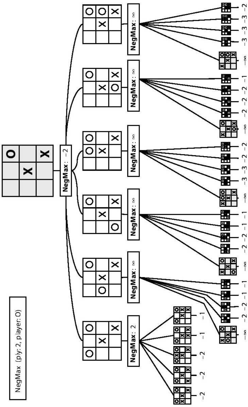
图 7-19 NegMax探测
