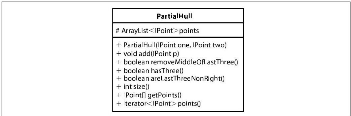
图 9-11 PartialHull类
