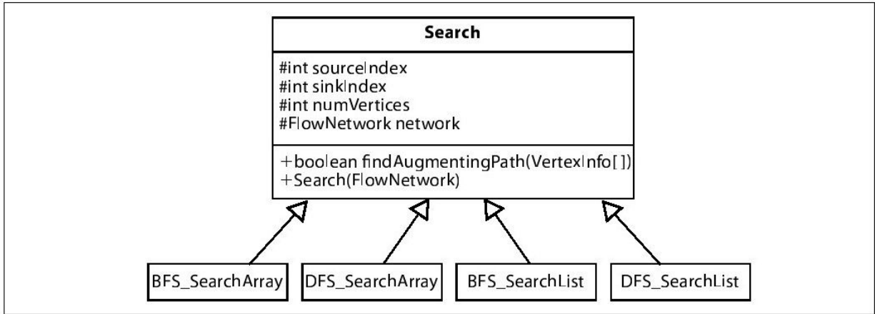
图 8-5 Search的功能
