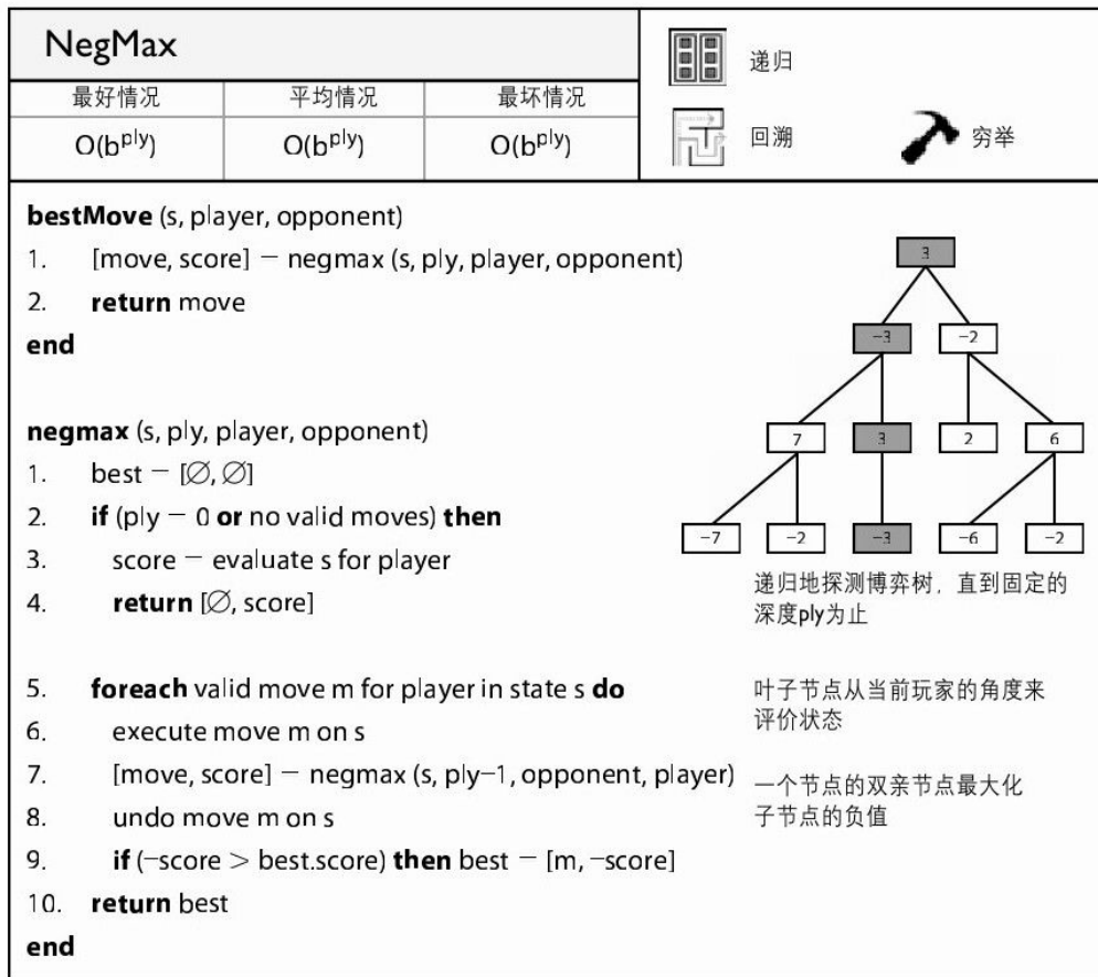
图 7-18 NegMax详解
