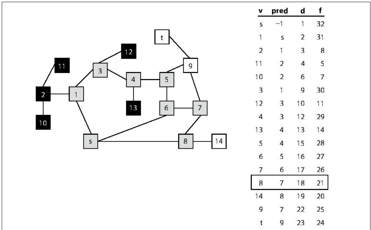
图 6-10 在一个例图上计算d、f、pred，计数器为18时顶点的着色情况
