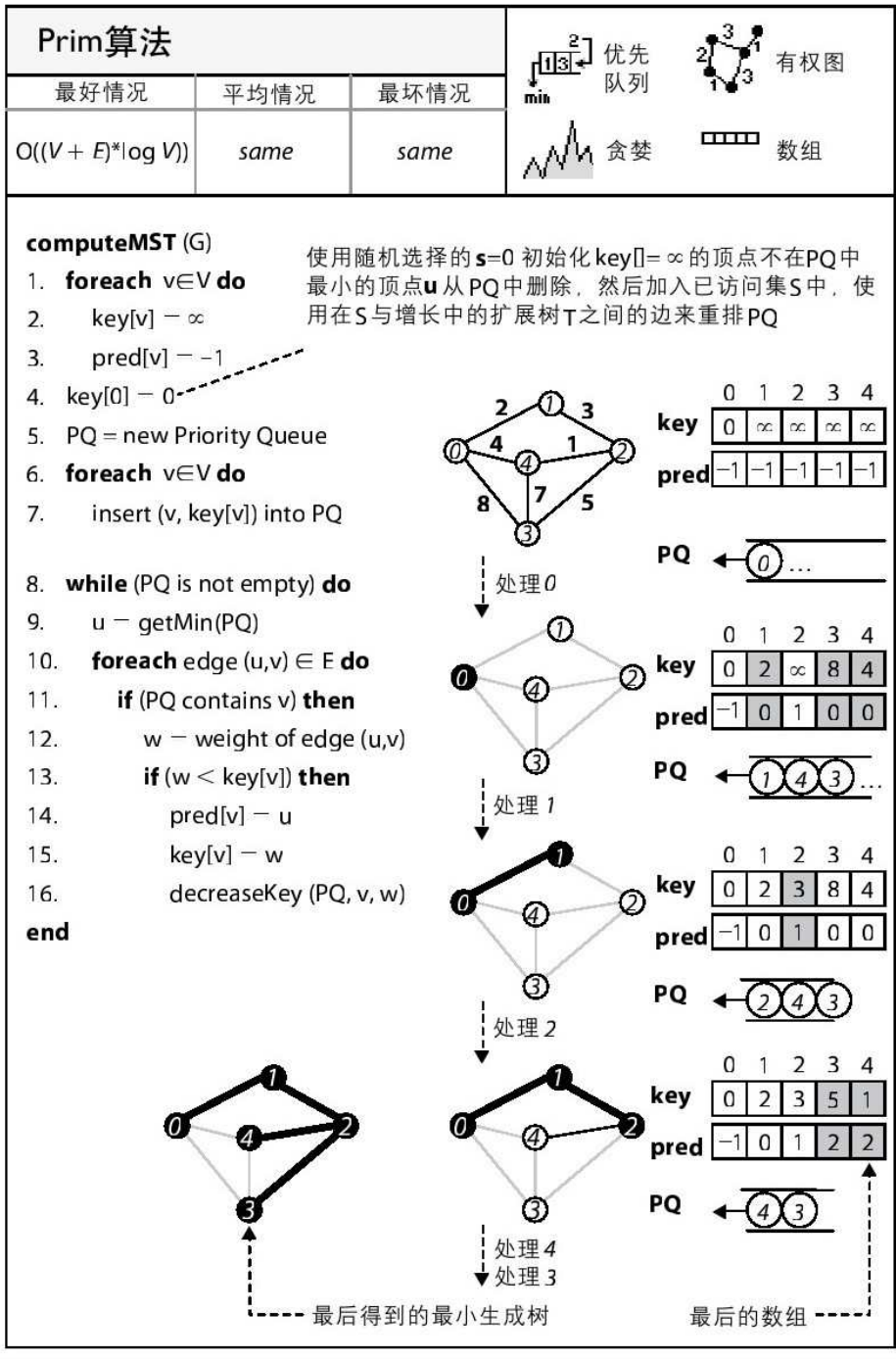
图 6-19 Prim算法详解
