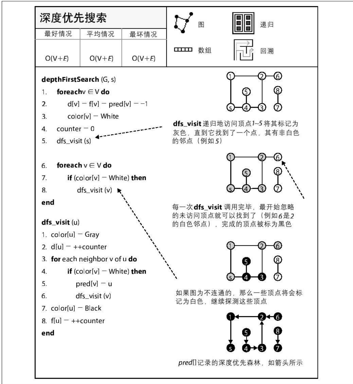
图 6-9 深度优先搜索详解
