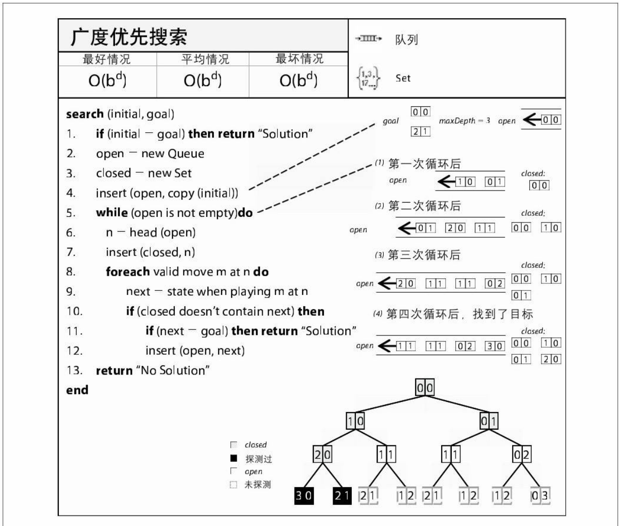
图 7-8 广度优先搜索详解
