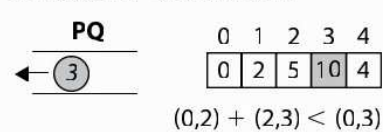
图 6-13 使用优先队列的Dijkstra算法详解
