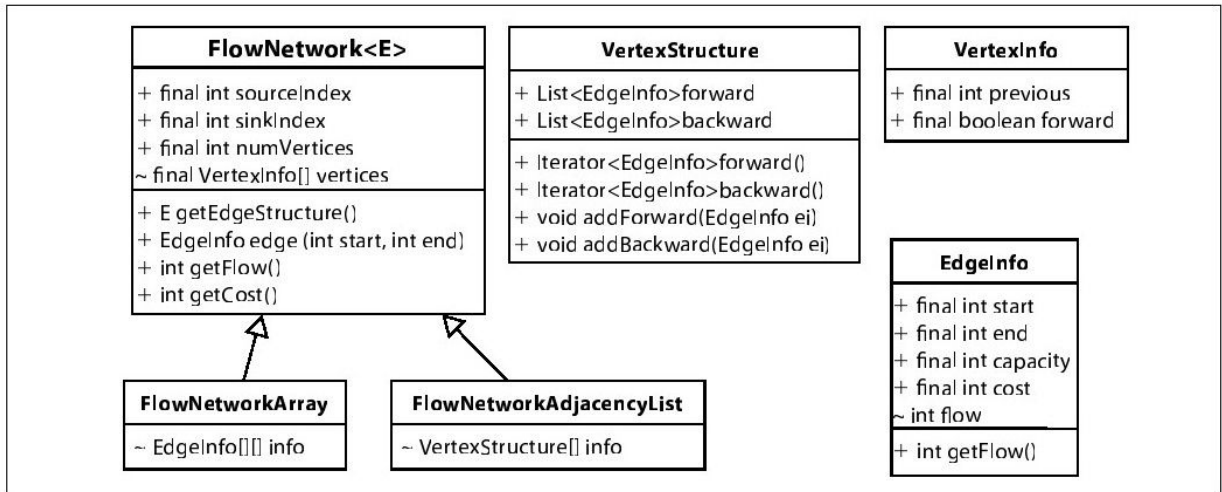
图 8-4 Ford-Fulkerson 的建模信息
