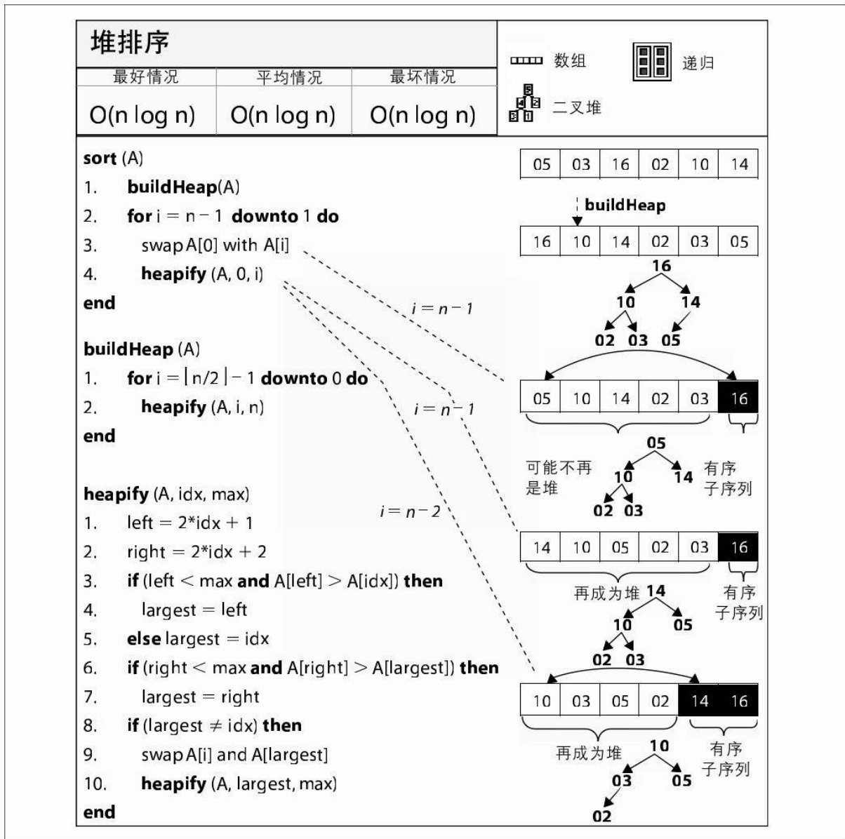
图 4-14 堆排序详解
