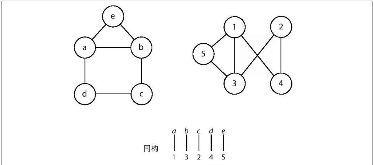
图 10-6 同构图示例
