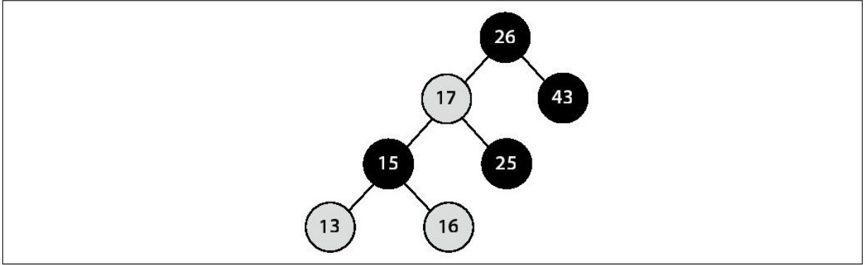
图 5-10 红黑树样例
