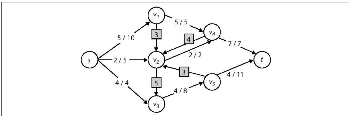
图 8-2 网络流图
