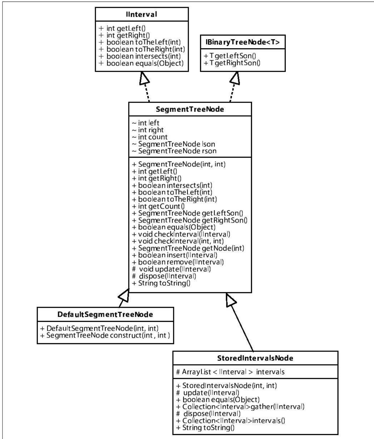
图 3-3 UML图样例
