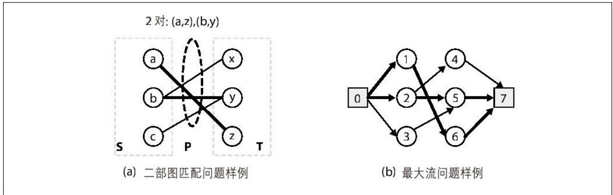
图 8-6 小规模的二部图匹配归约成最大流问题
