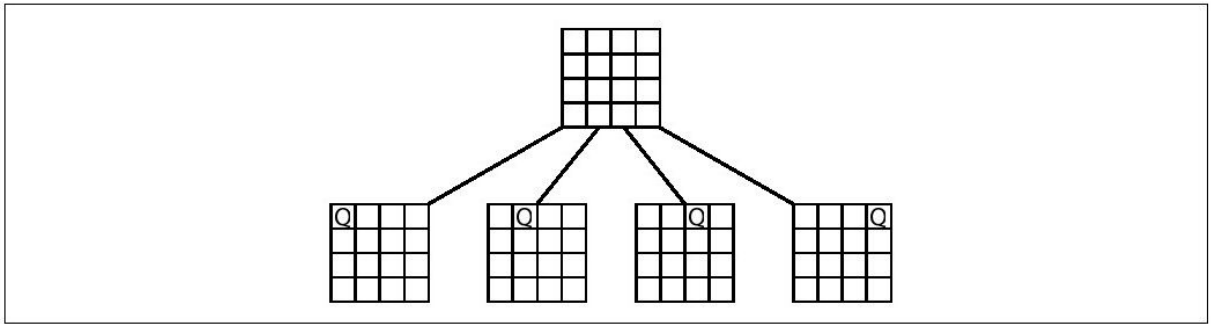
图 10-1 4皇后问题的初始搜索树
