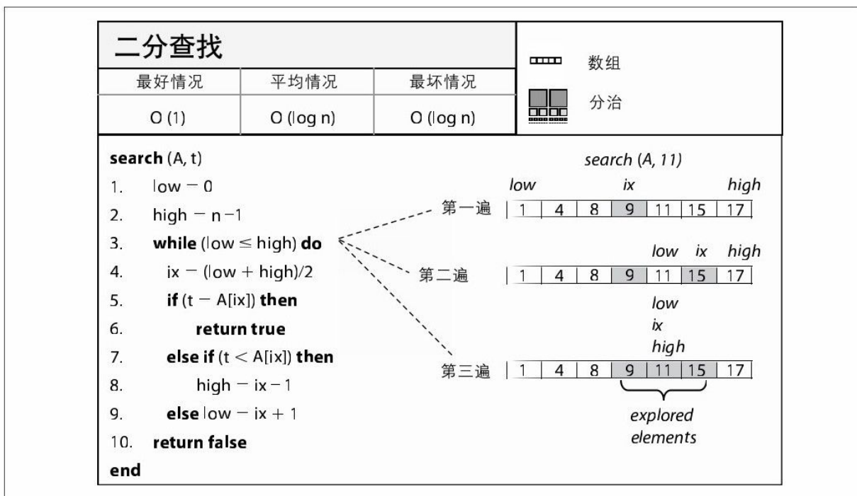
图 5-2 二分查找详解
