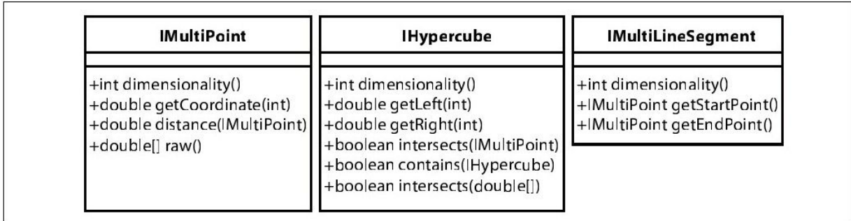
图 9-2 多维数据的接口
