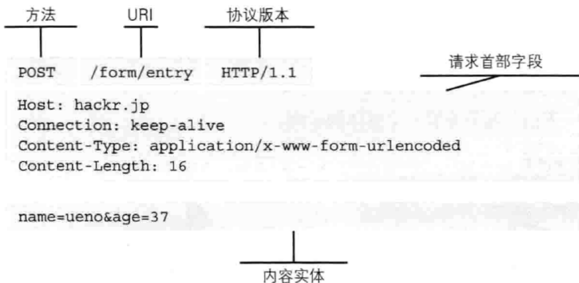
图：请求报文的构成
