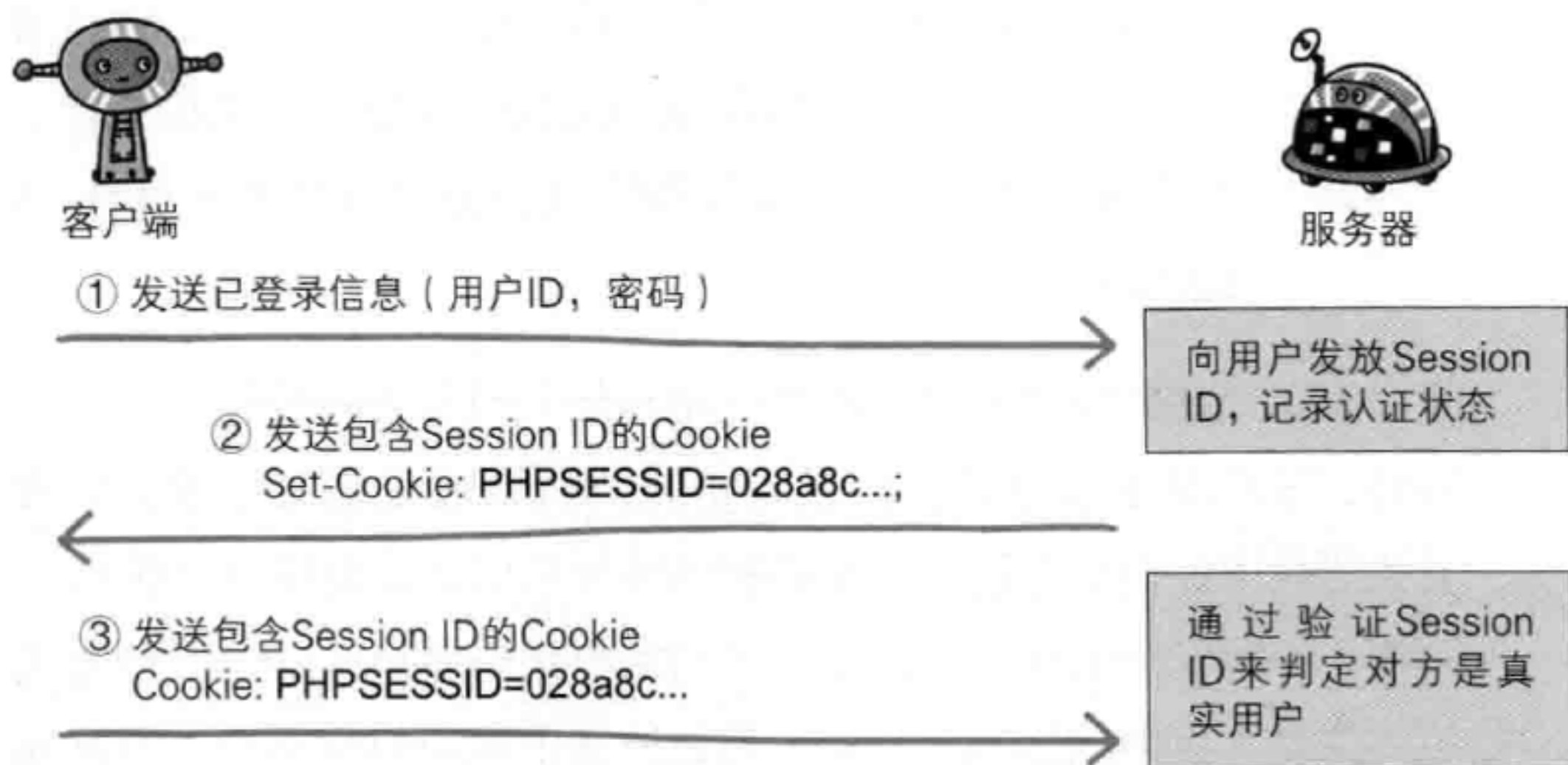
图：Session 管理及 Cookie 状态管理
