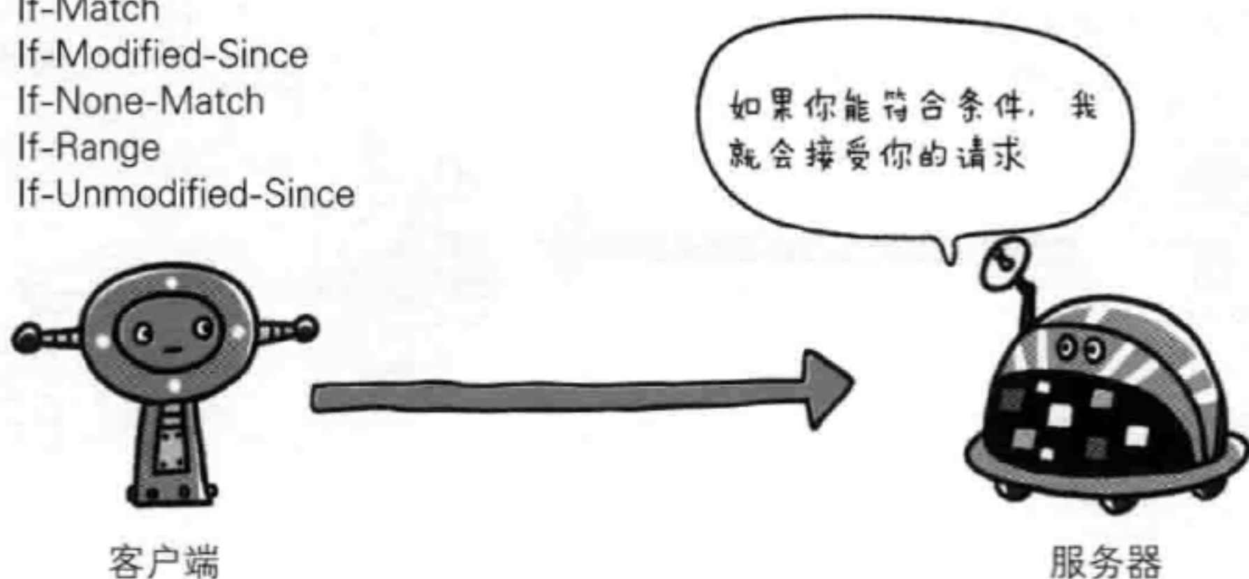
图：附带条件请求
