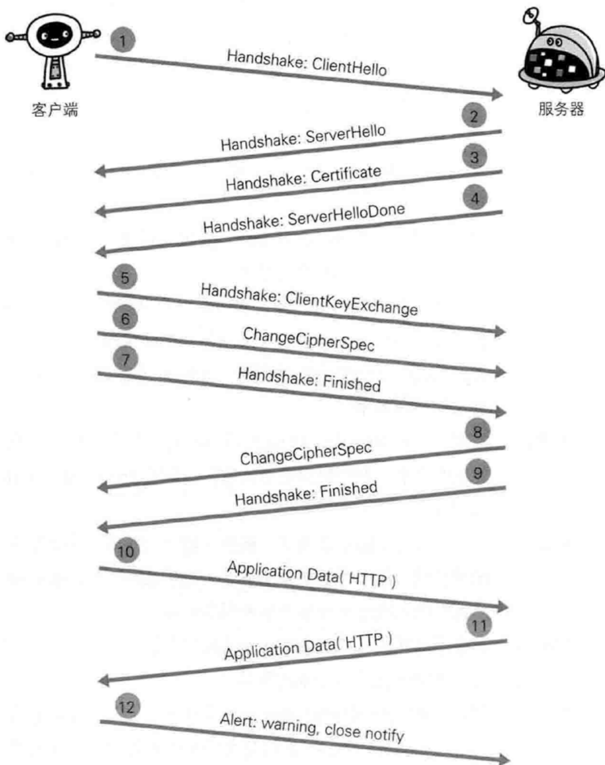
图：HTTPS 通信
