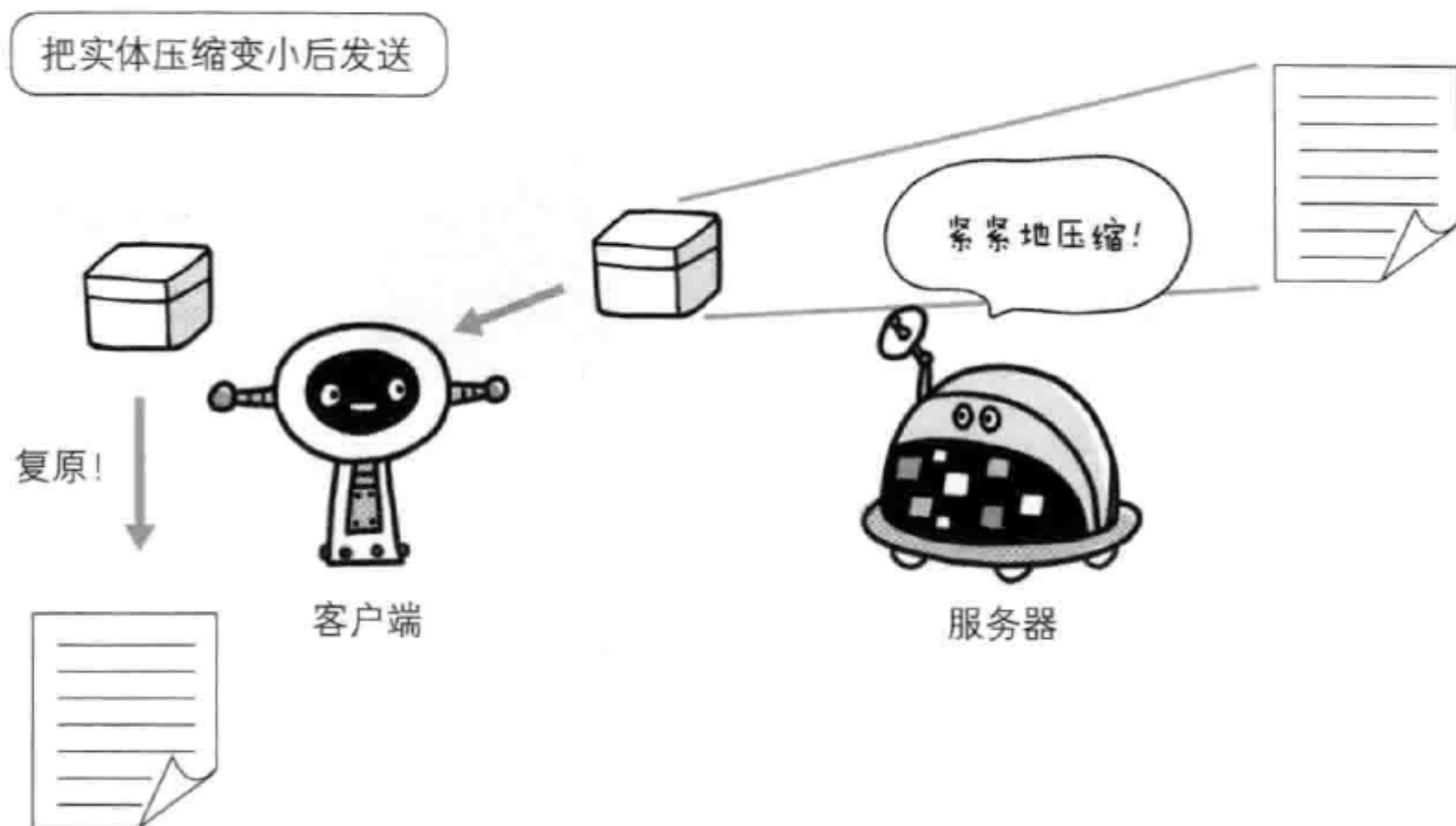
图：内容编码
