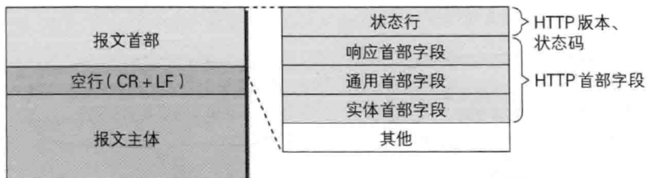
图：响应报文
