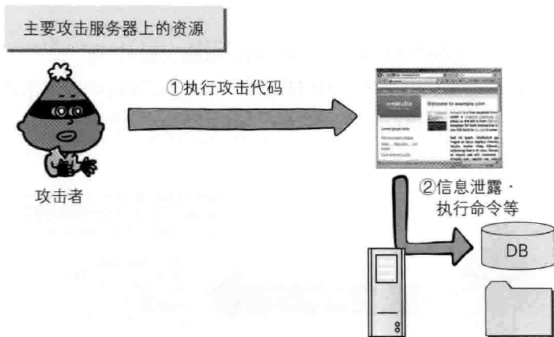
图：主动攻击
