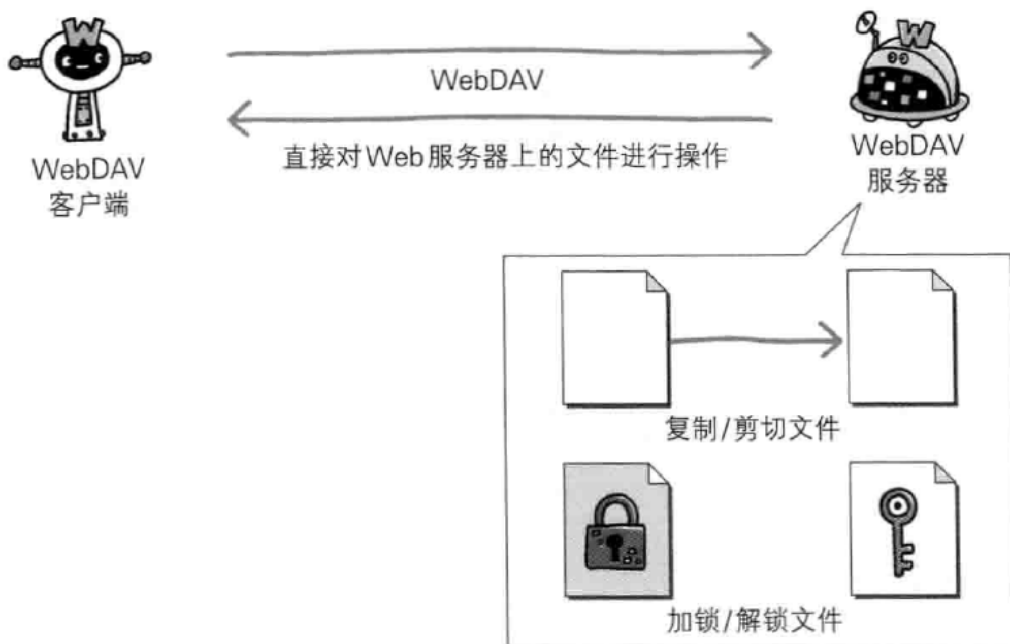
图: WebDAV
