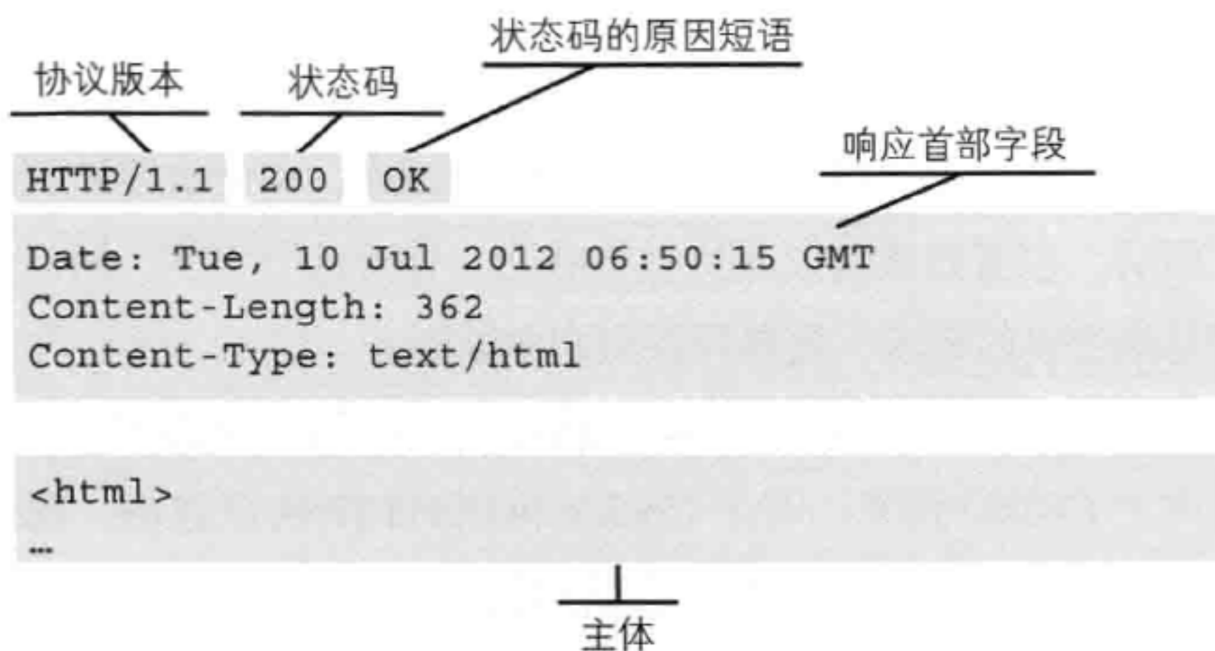
图：响应报文的构成
