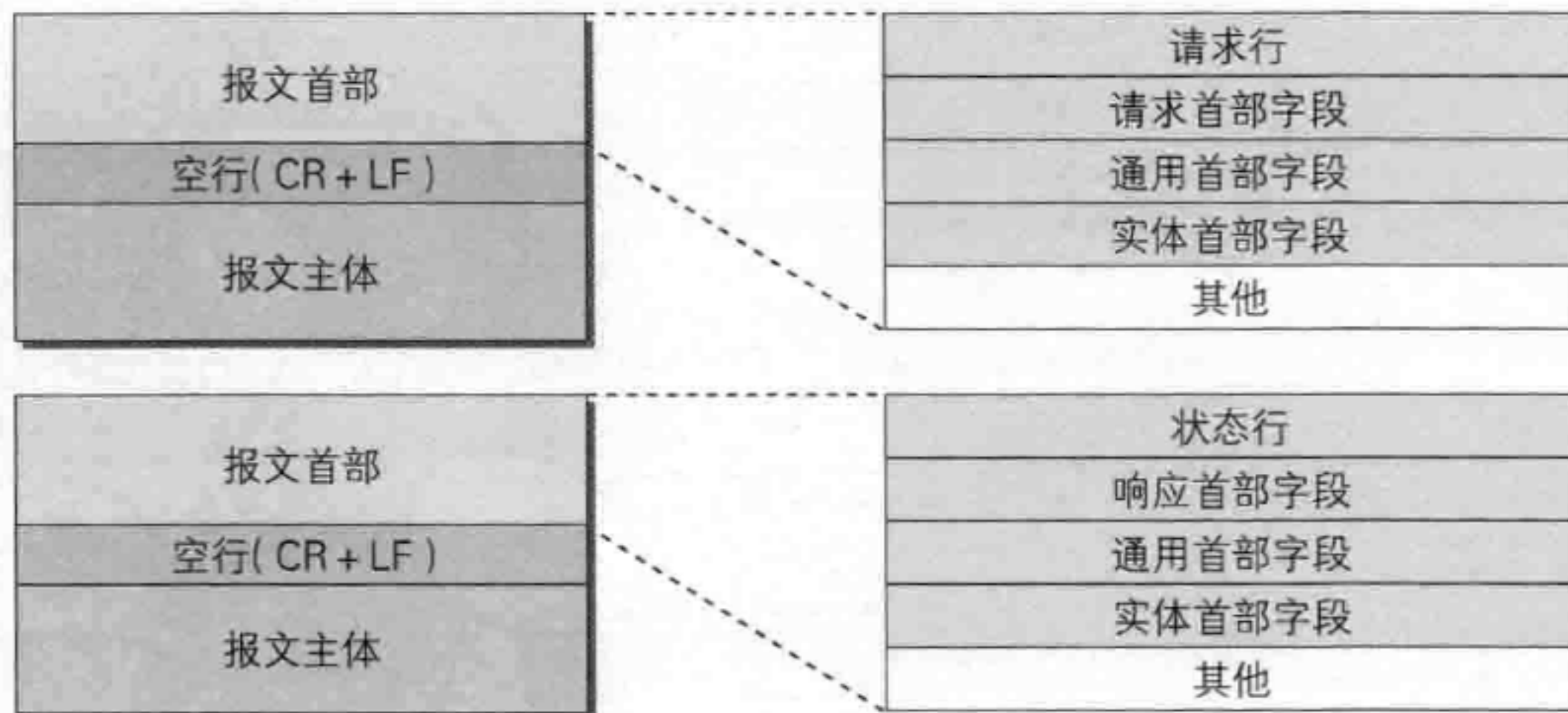
图: 请求报文（上）和响应报文（下）的结构
