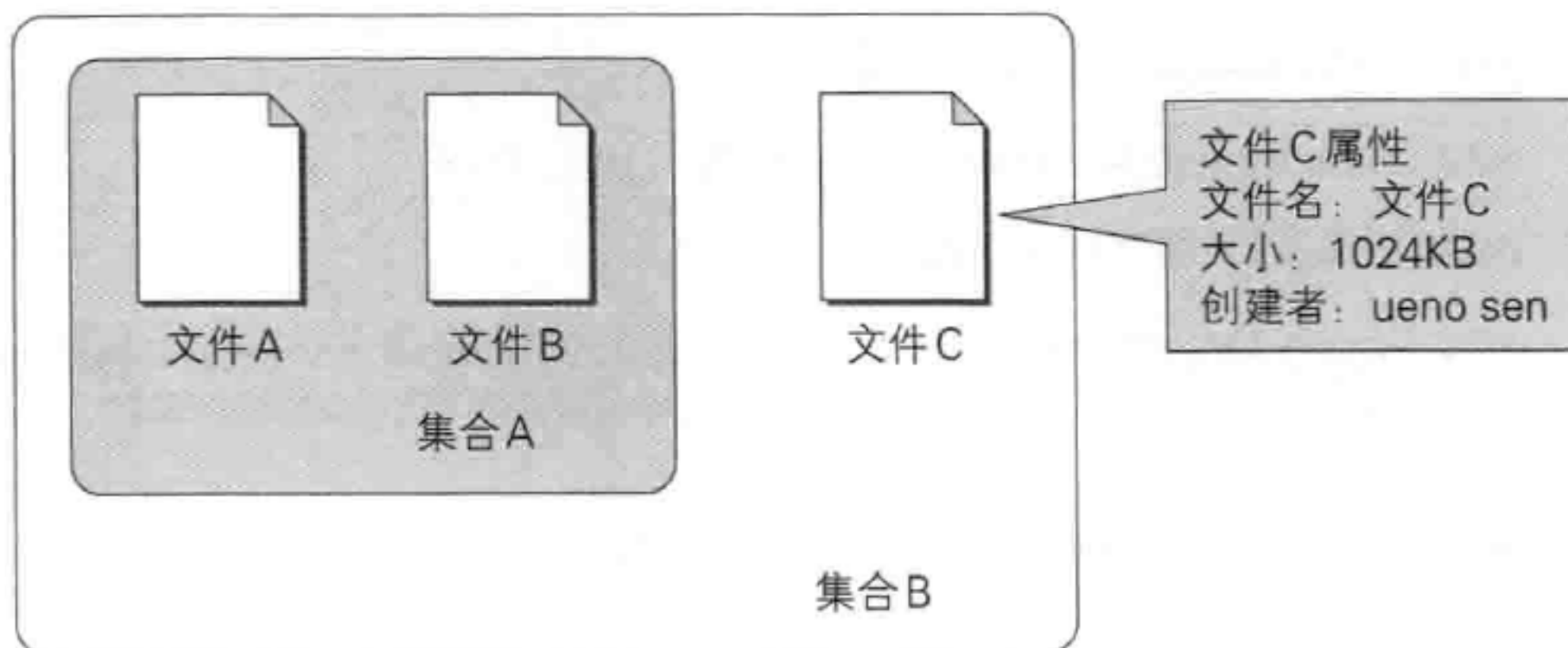
图: WebDAV 扩展的概念
