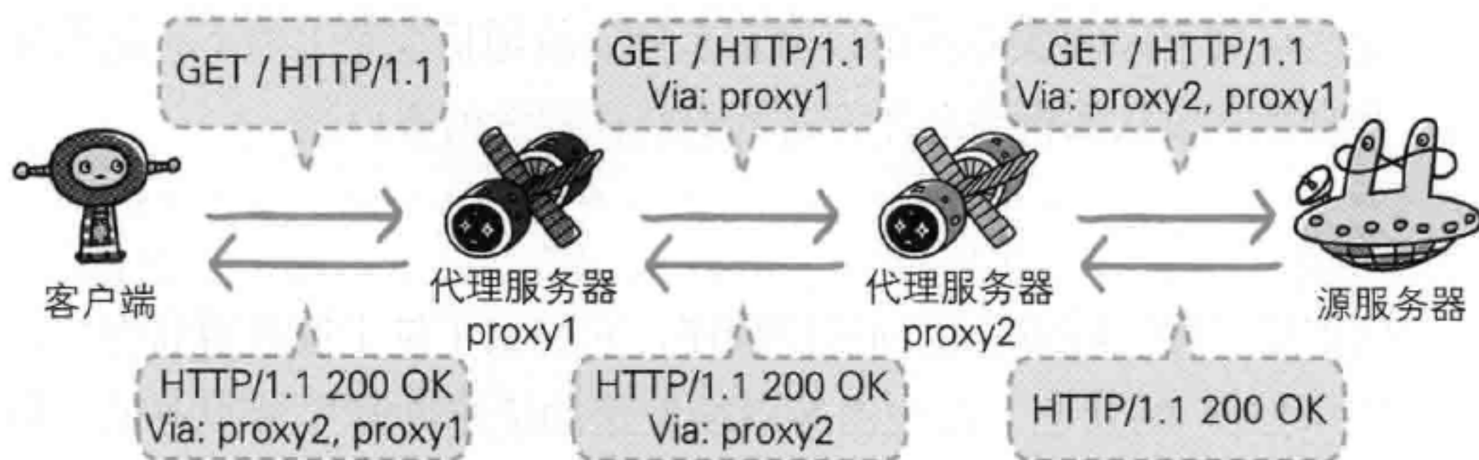
图：每次通过代理服务器转发请求或响应时，会追加写入 Via 首部信息
