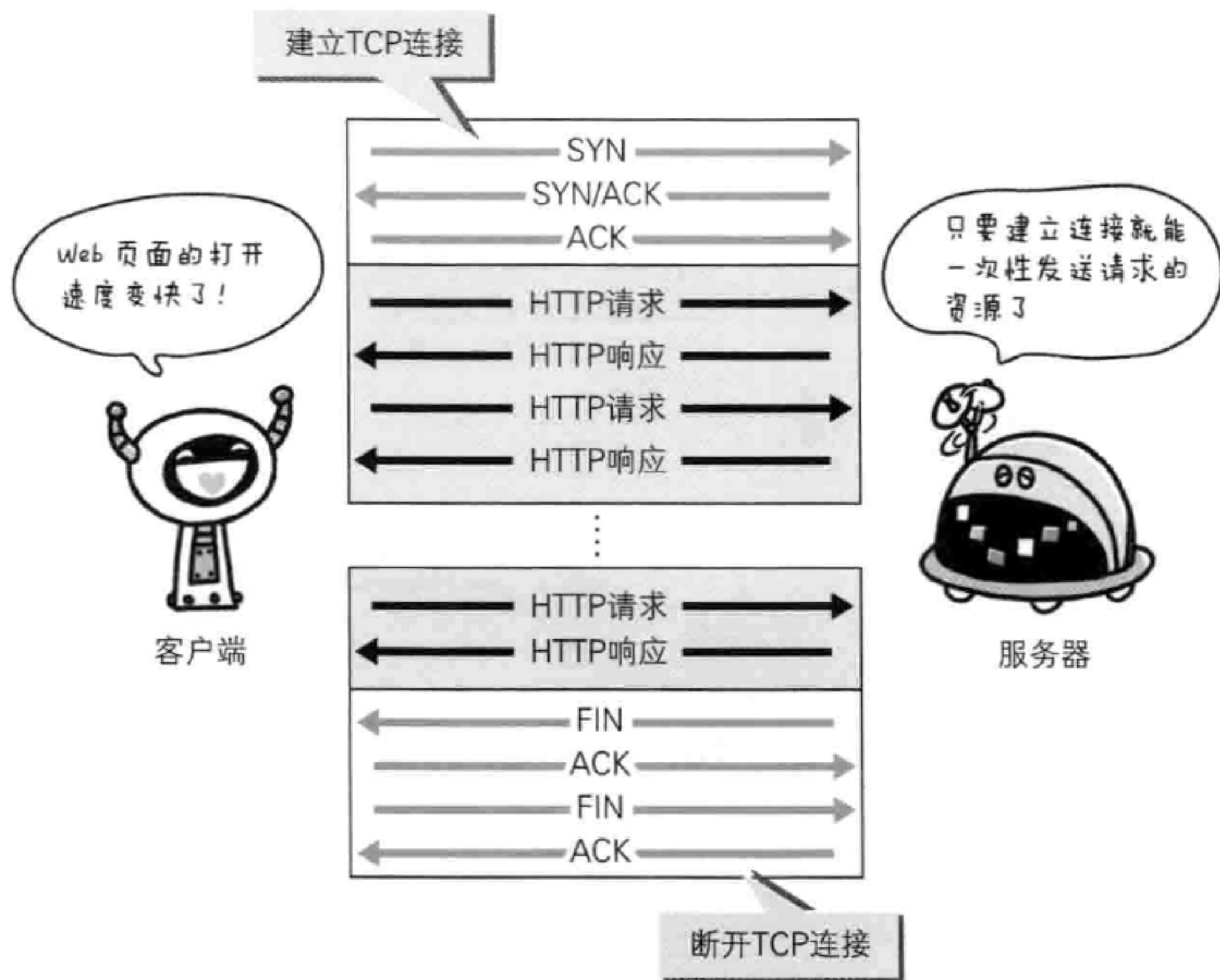
图：持久连接旨在建立 1 次 TCP 连接后进行多次请求和响应的交互
