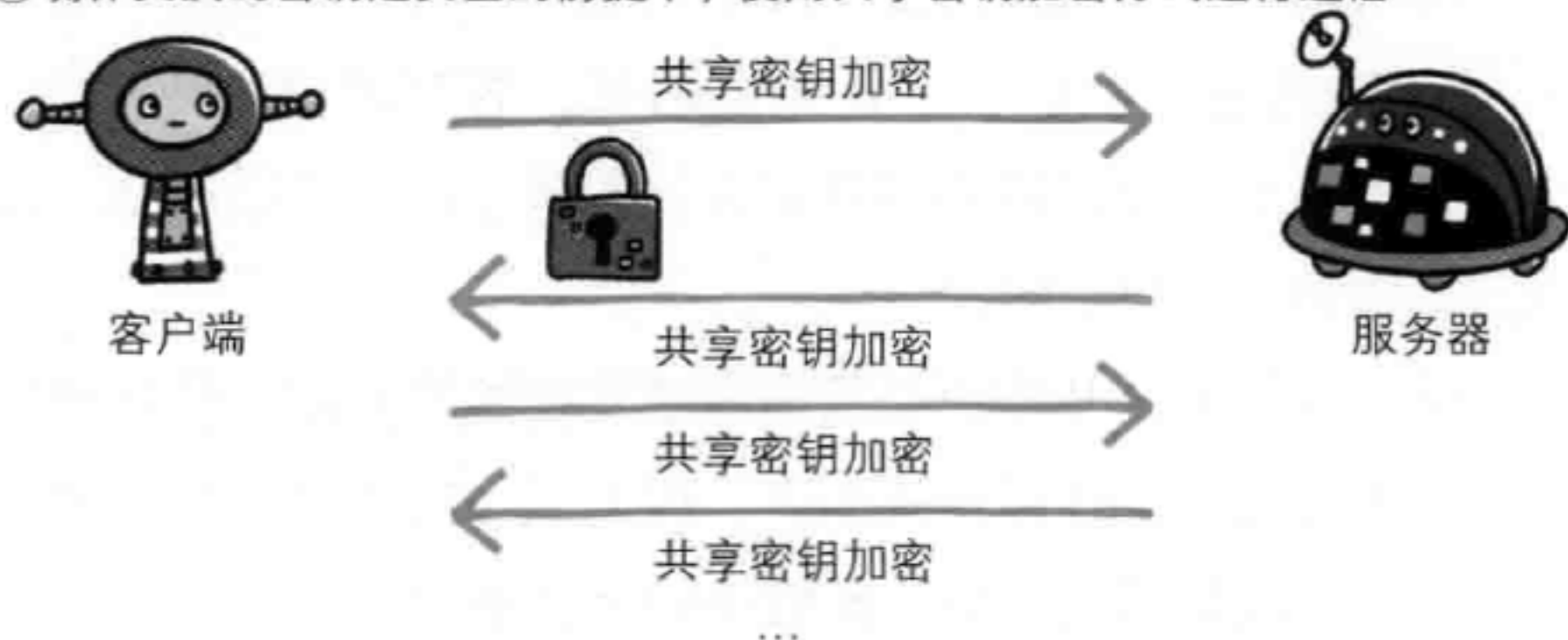
图：混合加密机制
