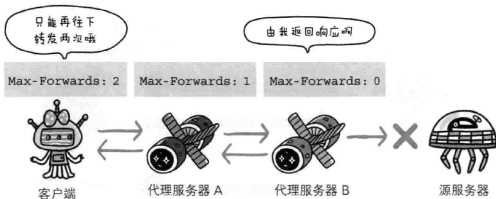
图：每次转发数值减 1。当数值变 0 时返回响应
