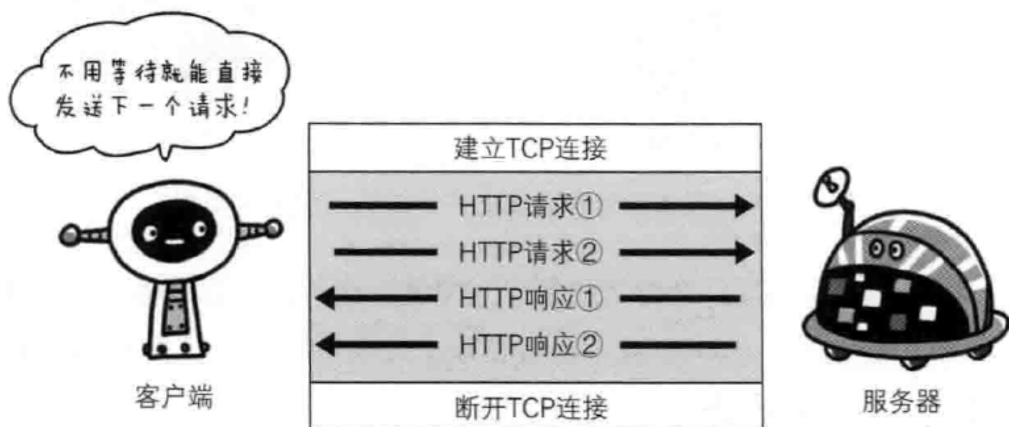
图：不等待响应，直接发送下一个请求
