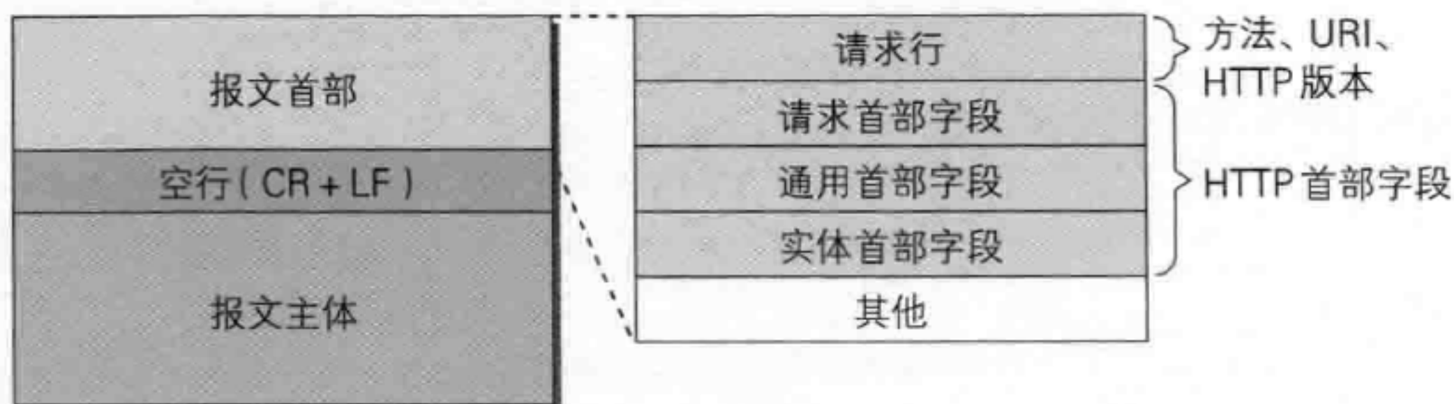
图：请求报文
