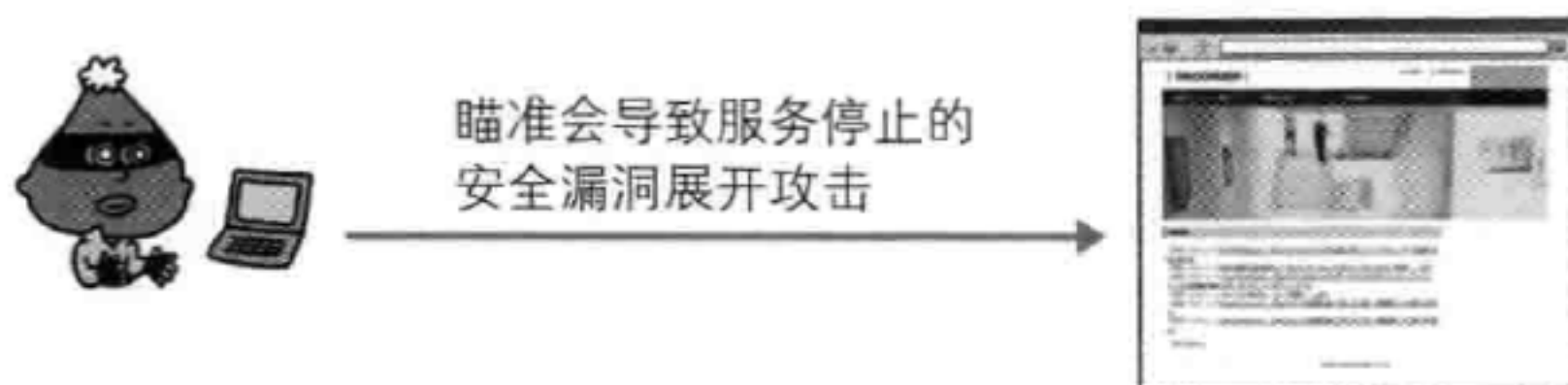
图：DoS 攻击
