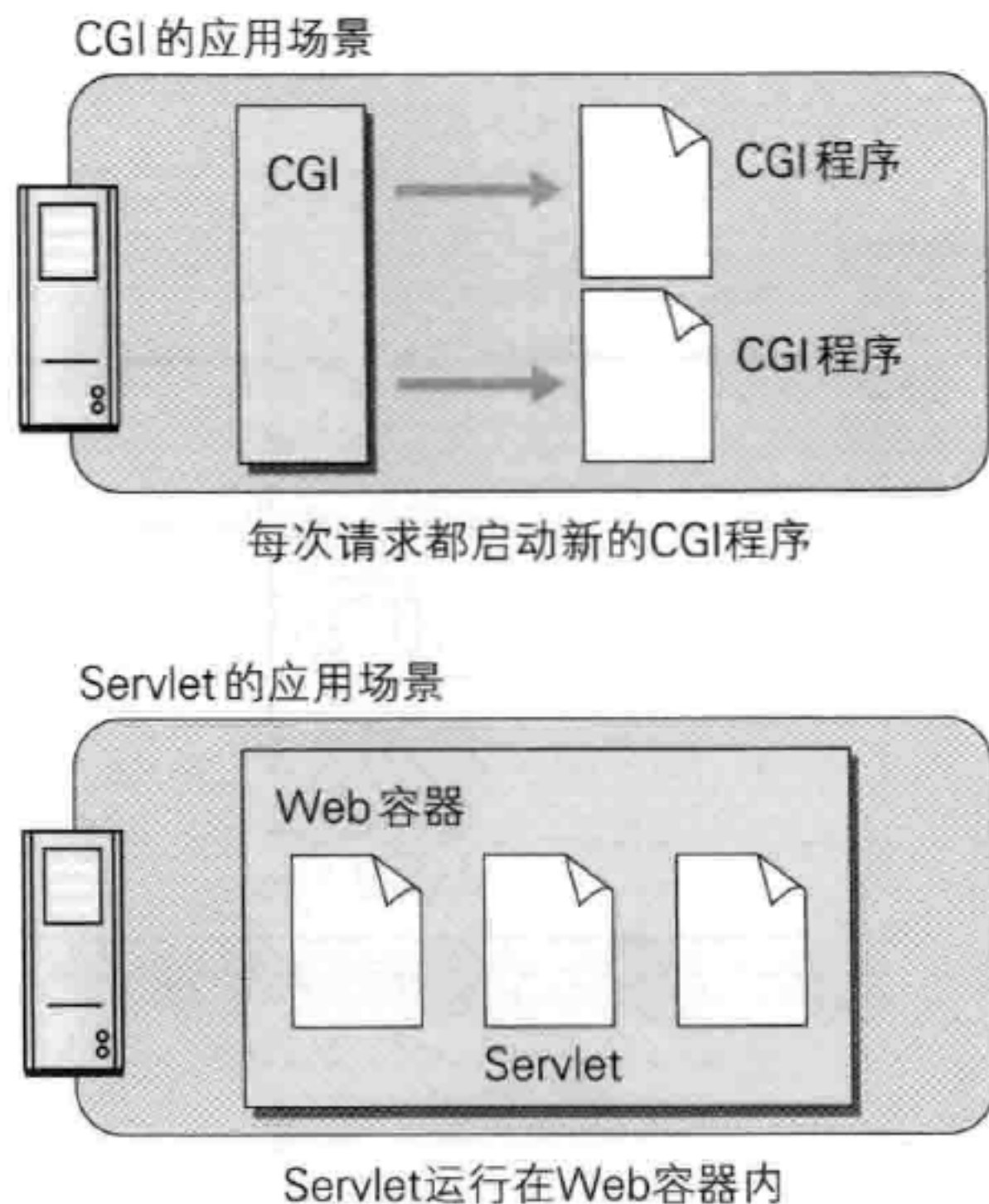
图：Servlet
