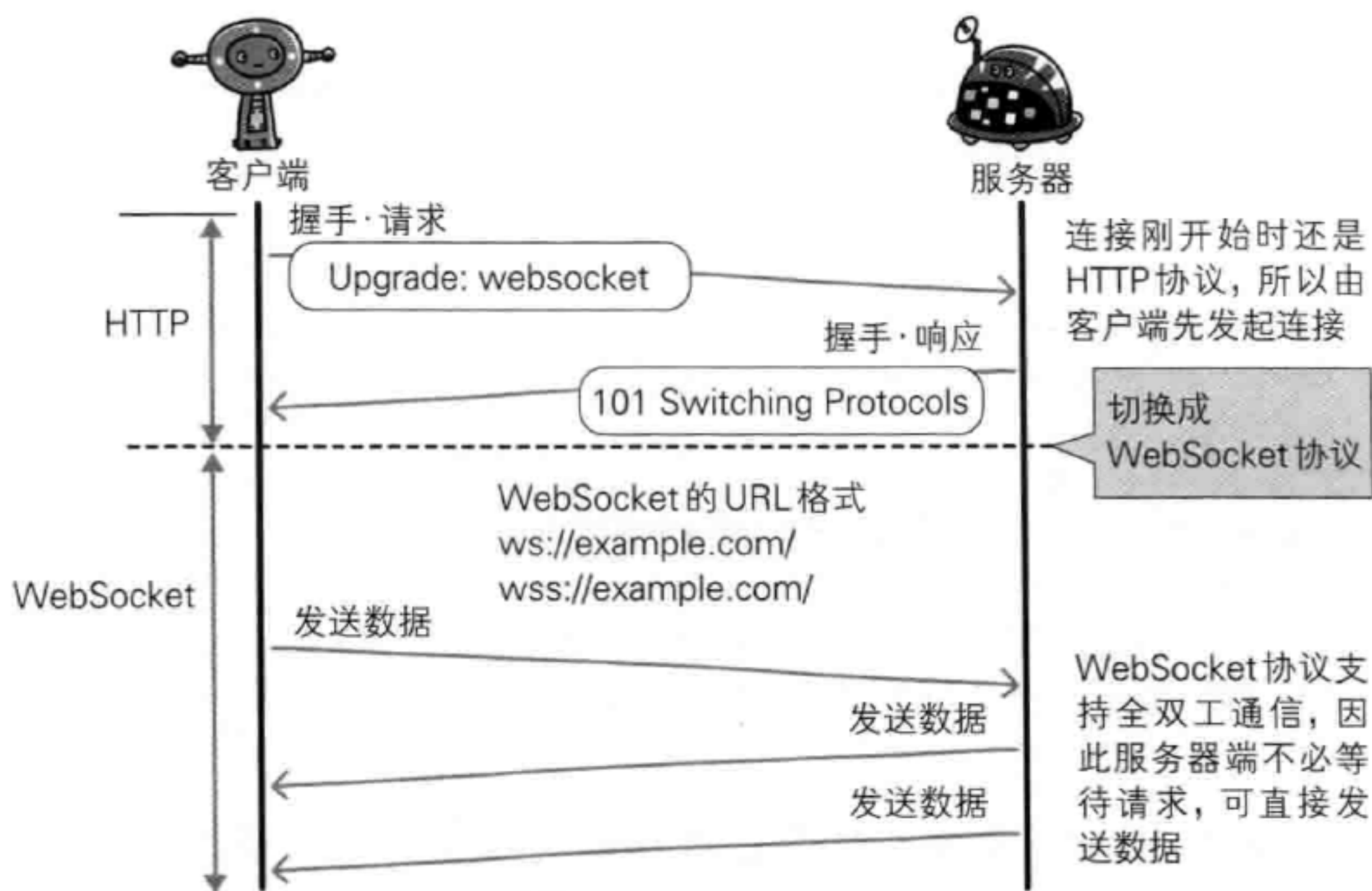
图：WebSocket 通信
