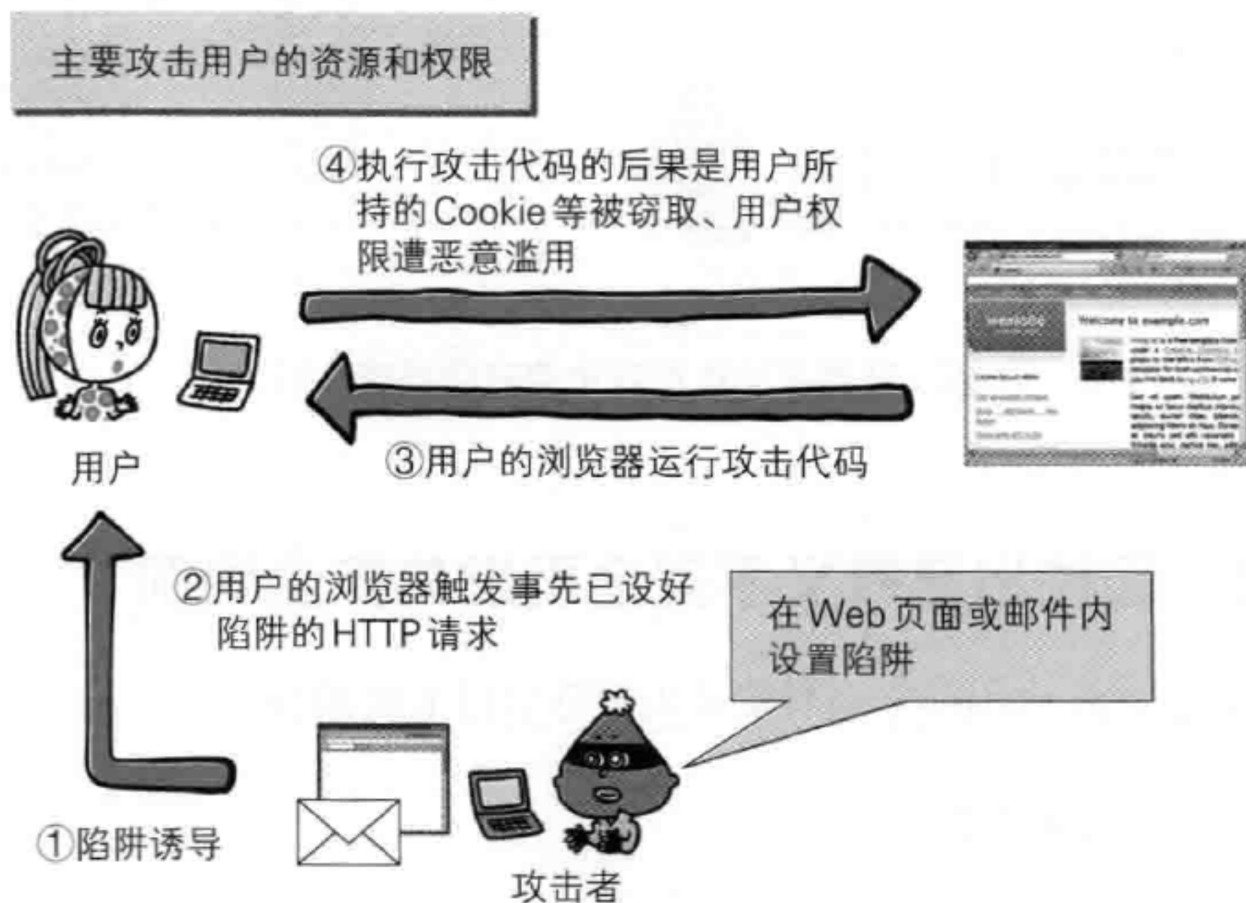
图：被动攻击
