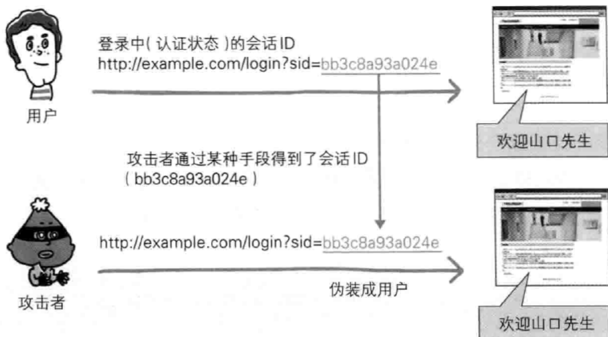
图：会话劫持
