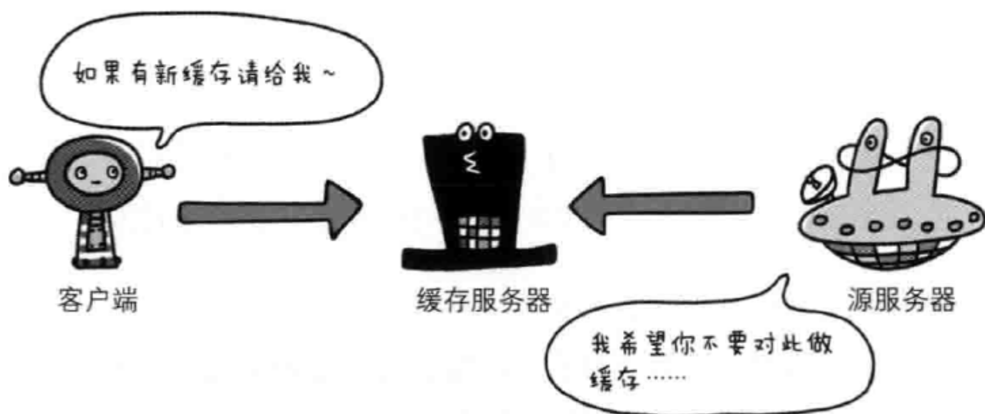
图：首部字段 Cache-Control 能够控制缓存的行为
