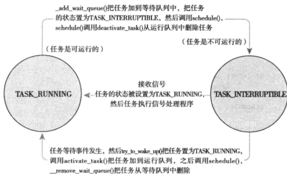
图 4-1 休眠和唤醒
