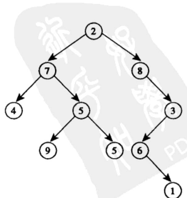
图 6-6 二叉树
