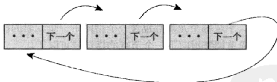
图 6-3 环形单向链表
