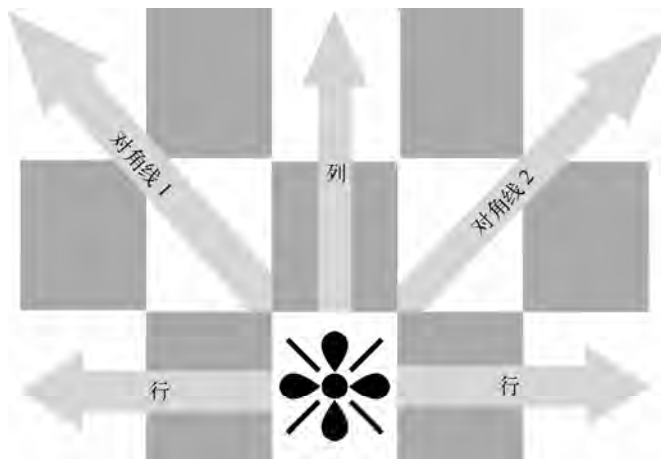
图4-2 八皇后规则
