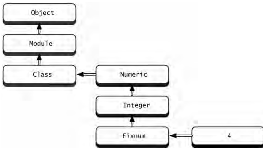
图2-1 Ruby元模型
