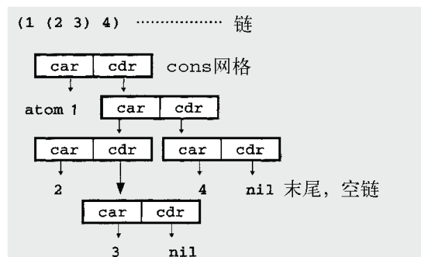
图 14-2 Lisp 的链
