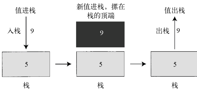
图 2-8 栈的构造
