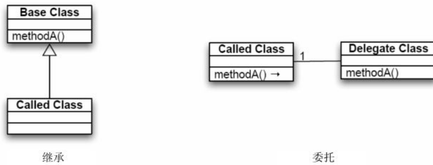
图6-3 委托与继承
