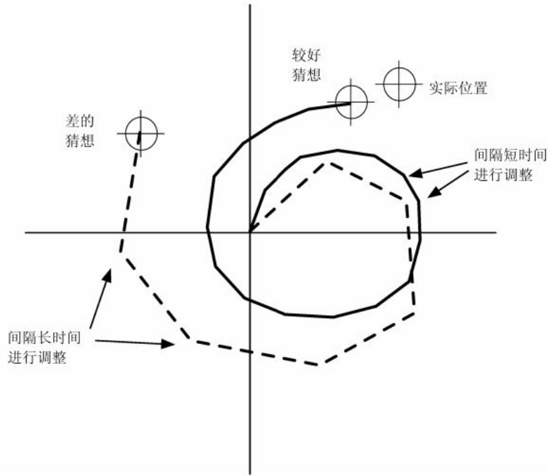
图4-1 计算宇宙飞船的运行轨线
