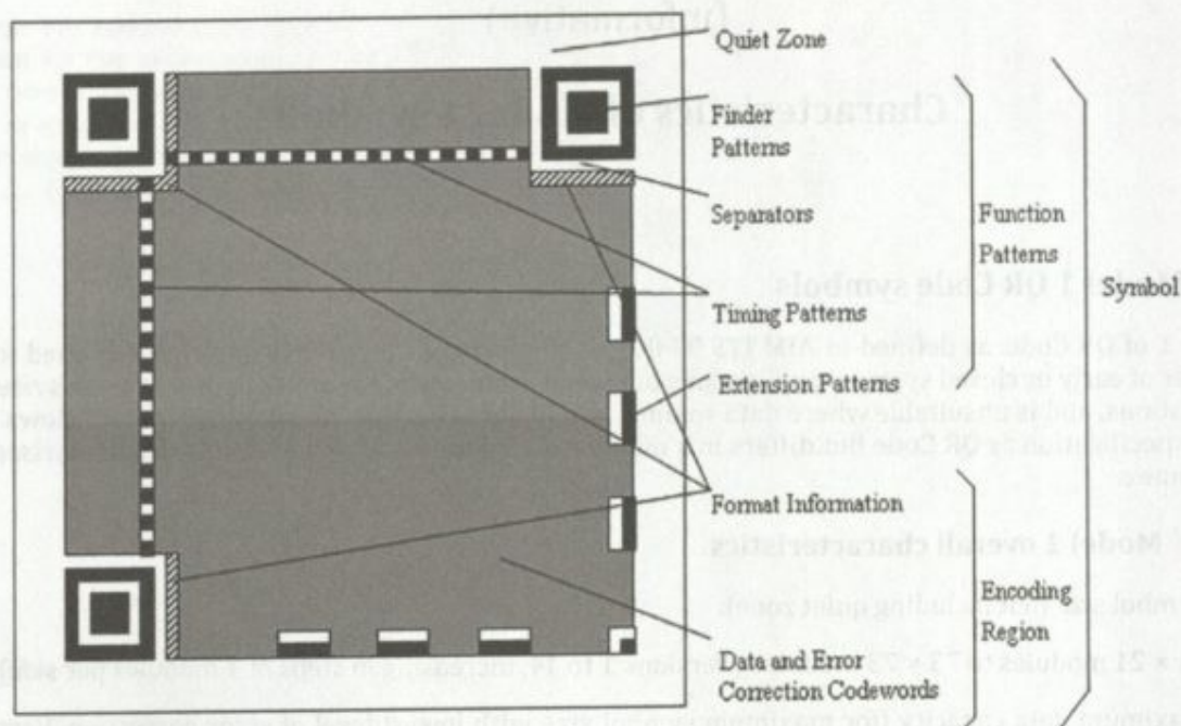
Figure N.1 — Structure of a QR Code Model 1 symbol
