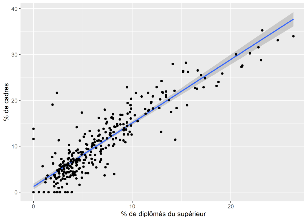
Figure 20. Nuage de points avec droite de régression linéaire
