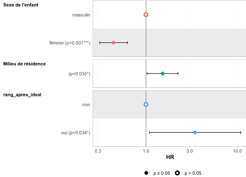
Figure 4. Coefficients du modèle avec ggcoef_model
