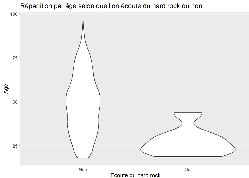
Figure 10. Graphiques en violon ou violin plot
