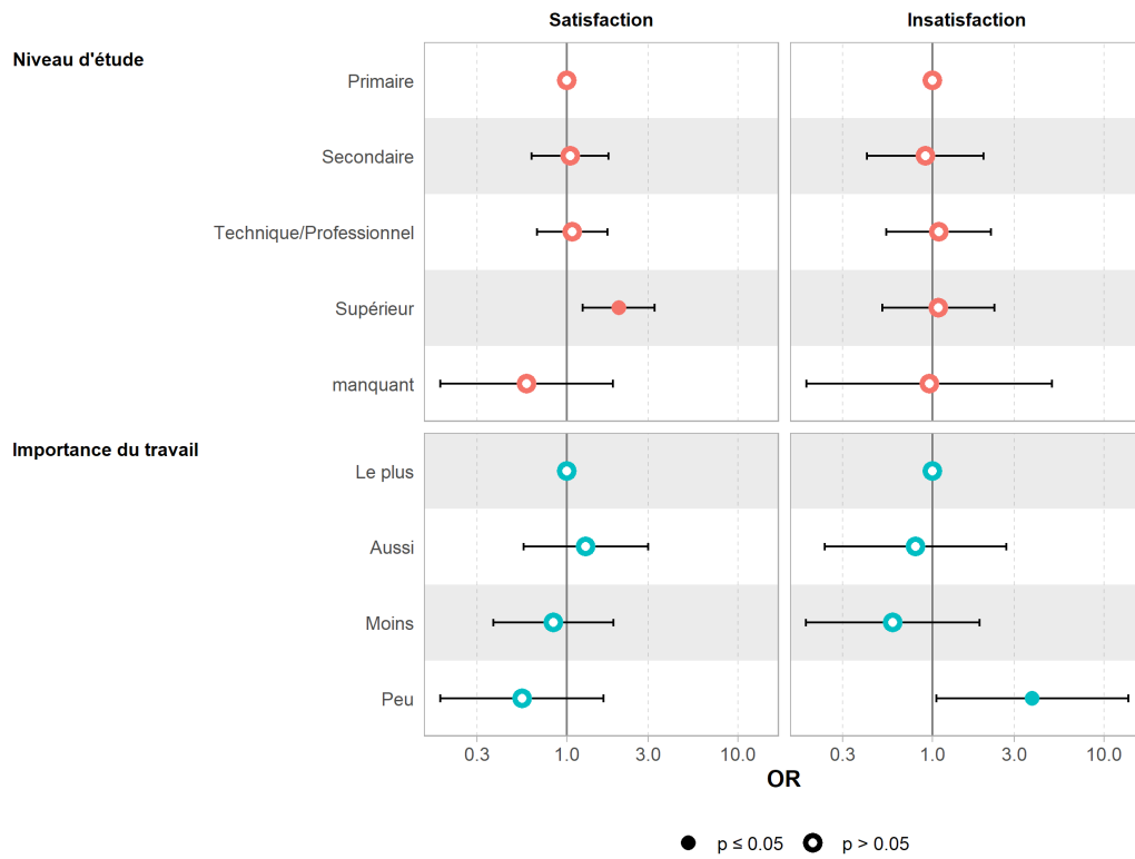
Figure 8. La fonction ggcoef_multinom
