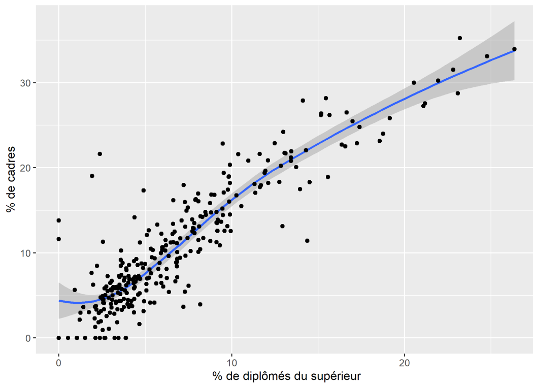
Figure 19. Nuage de points avec moyenne mobile
