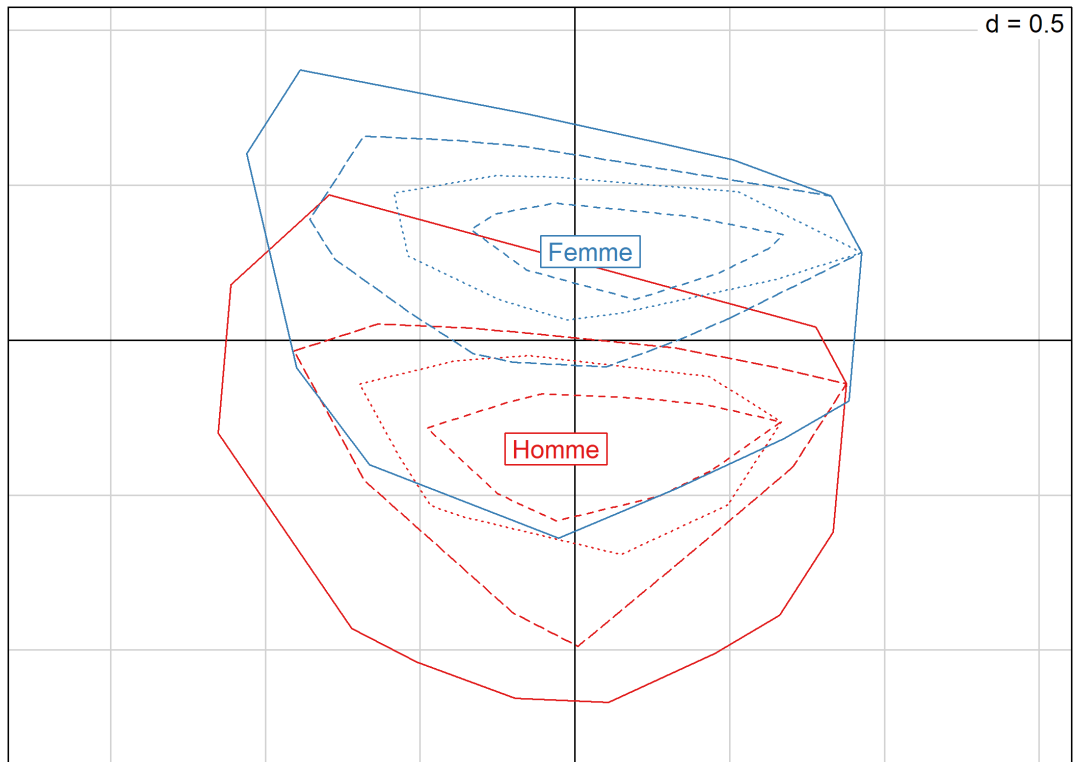
Figure 18. Individus dans le plan factoriel selon le sexe (s.chull)
