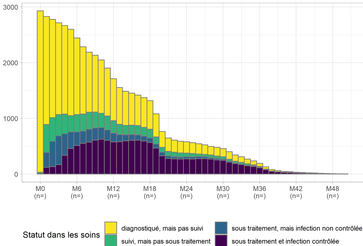
Distribution du statut dans les soins chaque mois
