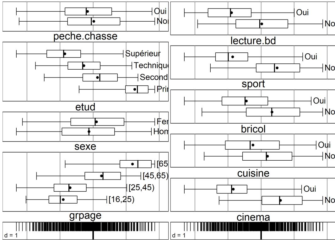
Figure 6. Répartition des modalités selon le premier axe
