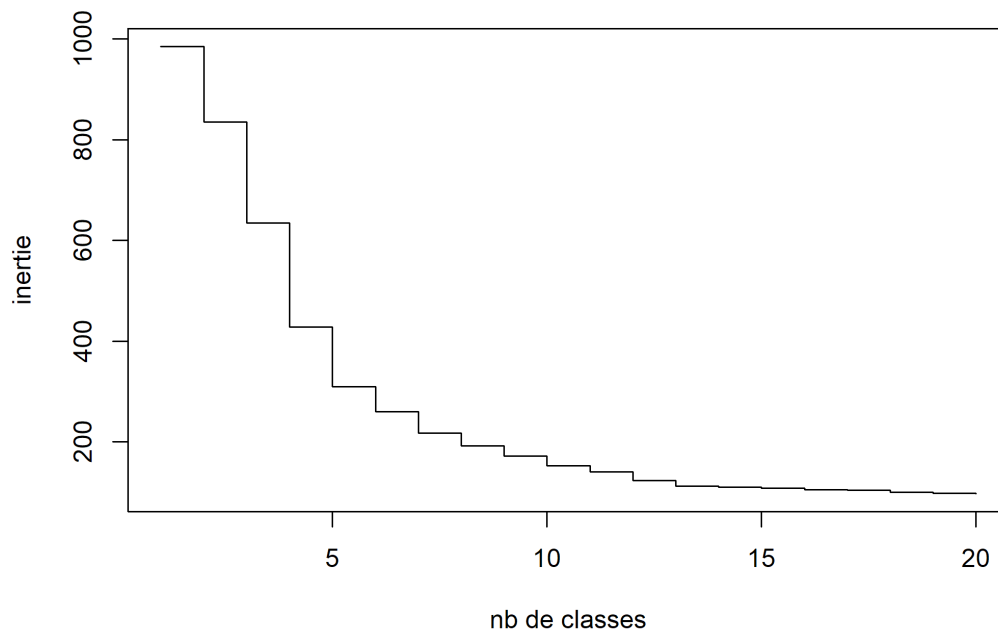
Figure 2. Sauts d'inertie de la classification des séquences
