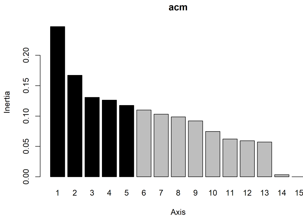
Figure 1. Valeurs propres ou inertie de chaque axe avec screeplot()
