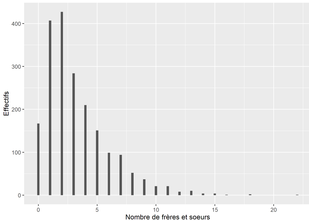
Figure 14. Diagramme en bâtons avec ajustement de la largeur des barres
