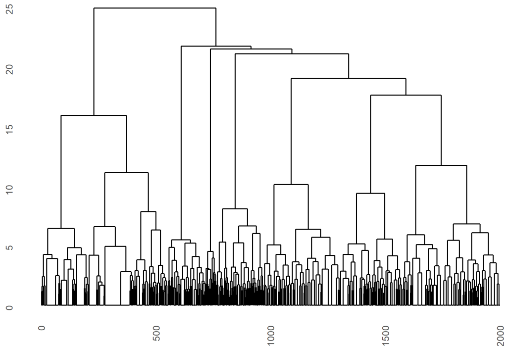
Figure 2. Dendrogramme obtenu avec ggdendrogram
