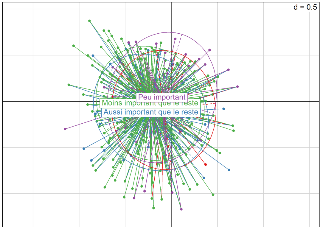
Figure 20. Individus dans le plan factoriel selon l'importance donnée au travail
