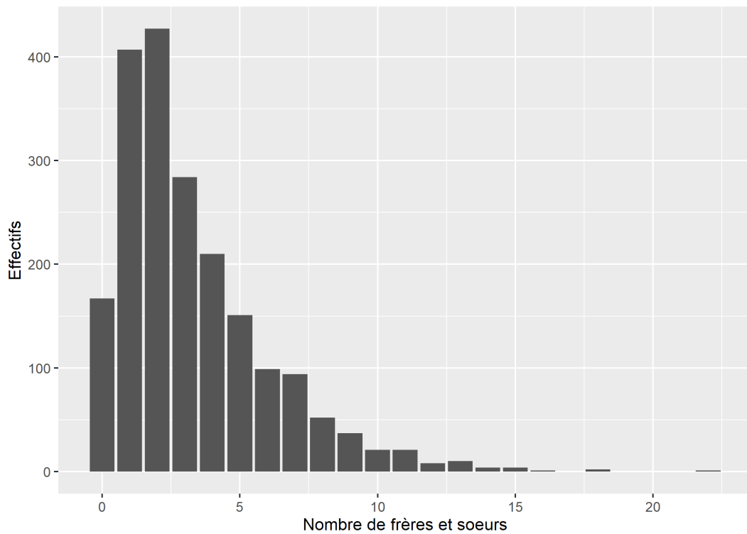
Figure 13. Diagramme en bâtons
