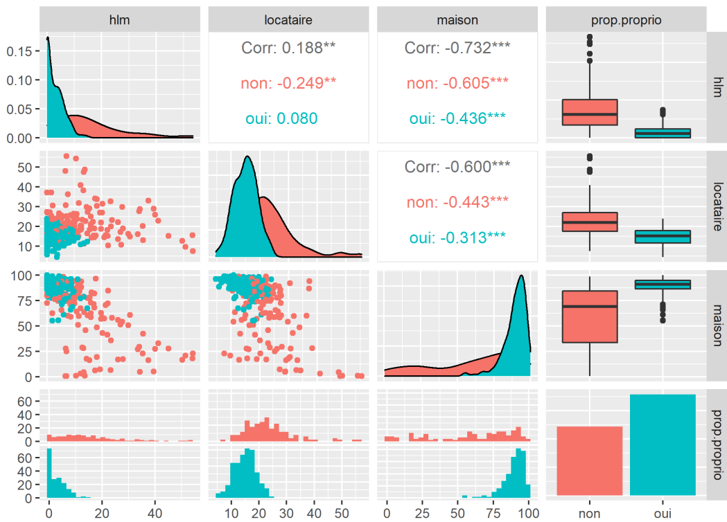
Figure 22. Matrice de nuages de points avec variables catégorielles
