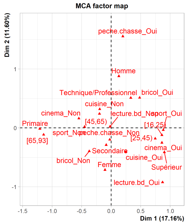
Figure 25. Plan factoriel (seulement les catégories)
