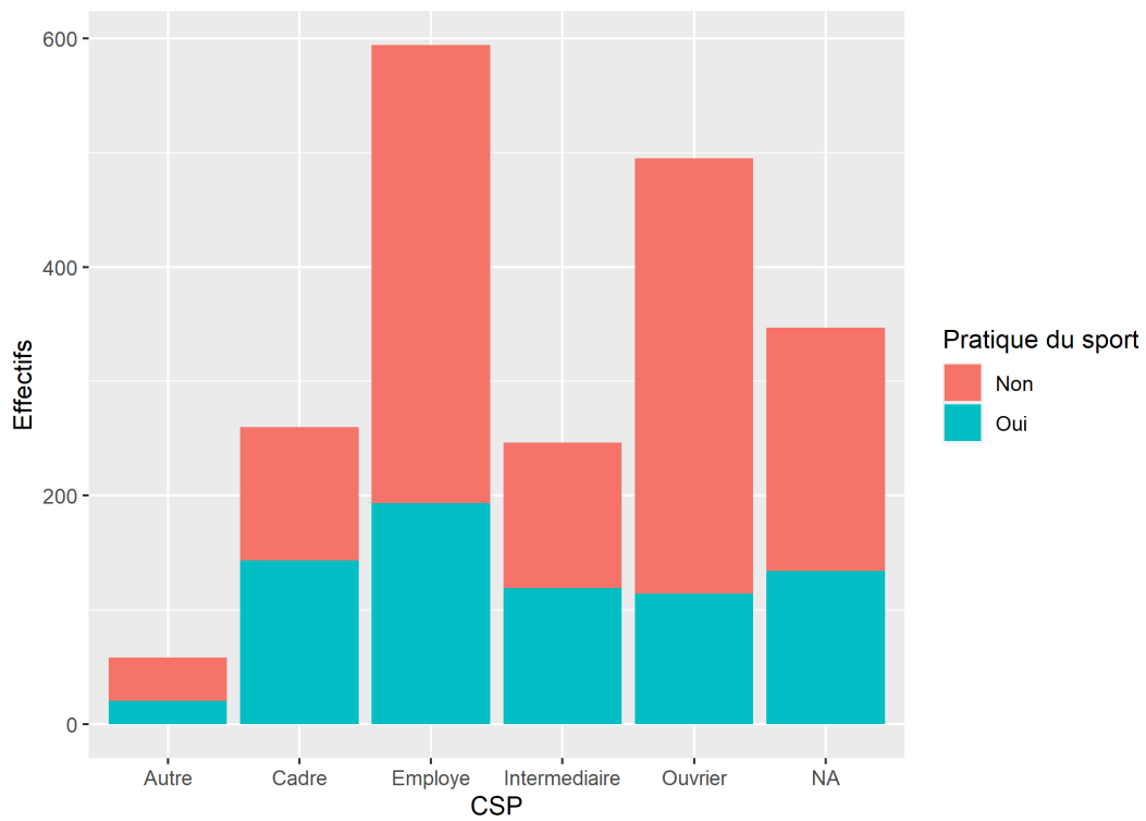
Figure 29. Diagramme en barres
