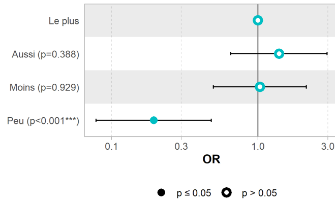
Figure 11. Coefficients du modèle ordinal
