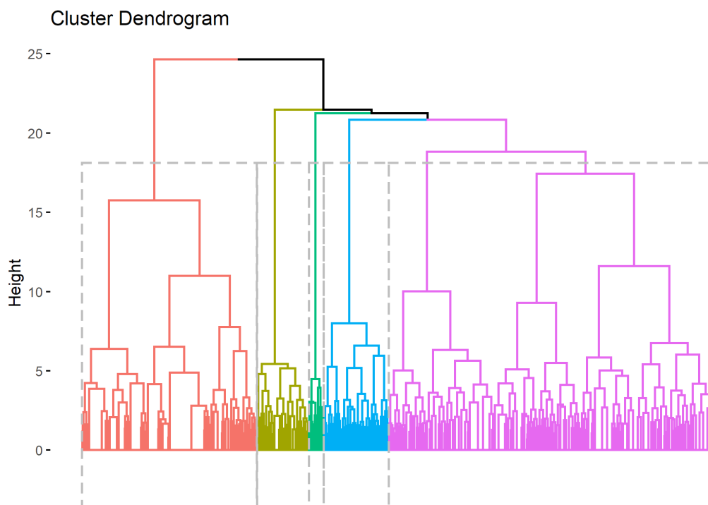
Figure 7. Un dendrogramme coloré avec factoextra
