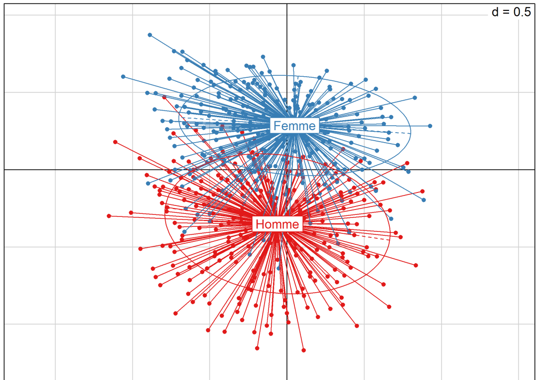
Figure 17. Individus dans le plan factoriel selon le sexe (s.class)
