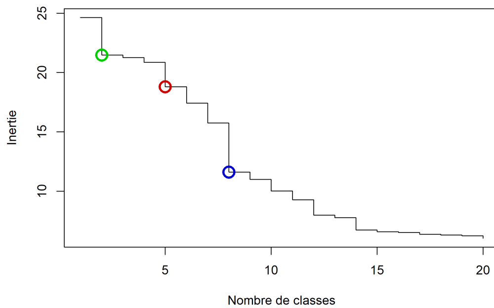
Figure 4. Sauts d'inertie du dendrogramme
