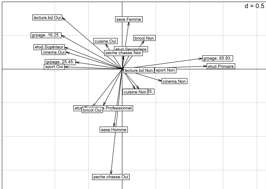
Figure 15. Vecteurs des modalités selon les deux premiers axes
