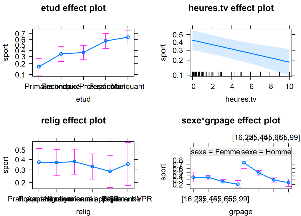
Figure 7. Représentation graphique des effets du modèle avec interaction simple entre le sexe et le groupe d'âge
