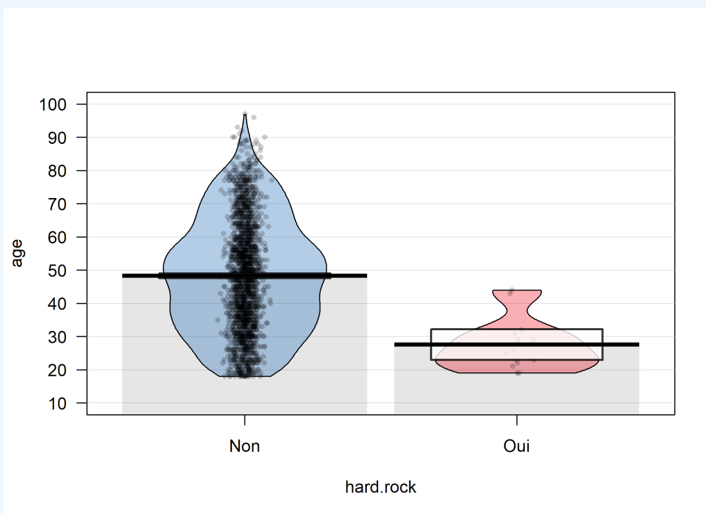
Figure 11. Graphique de «pirates»
