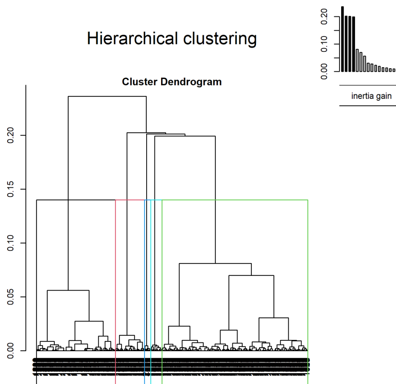
Figure 12. Dendrogramme obtenu avec HCPC (tous les axes)
