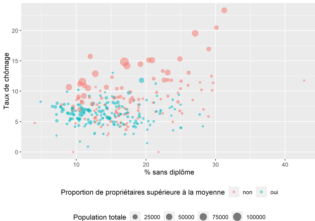
Figure 18. Nuage de points proportionnels
