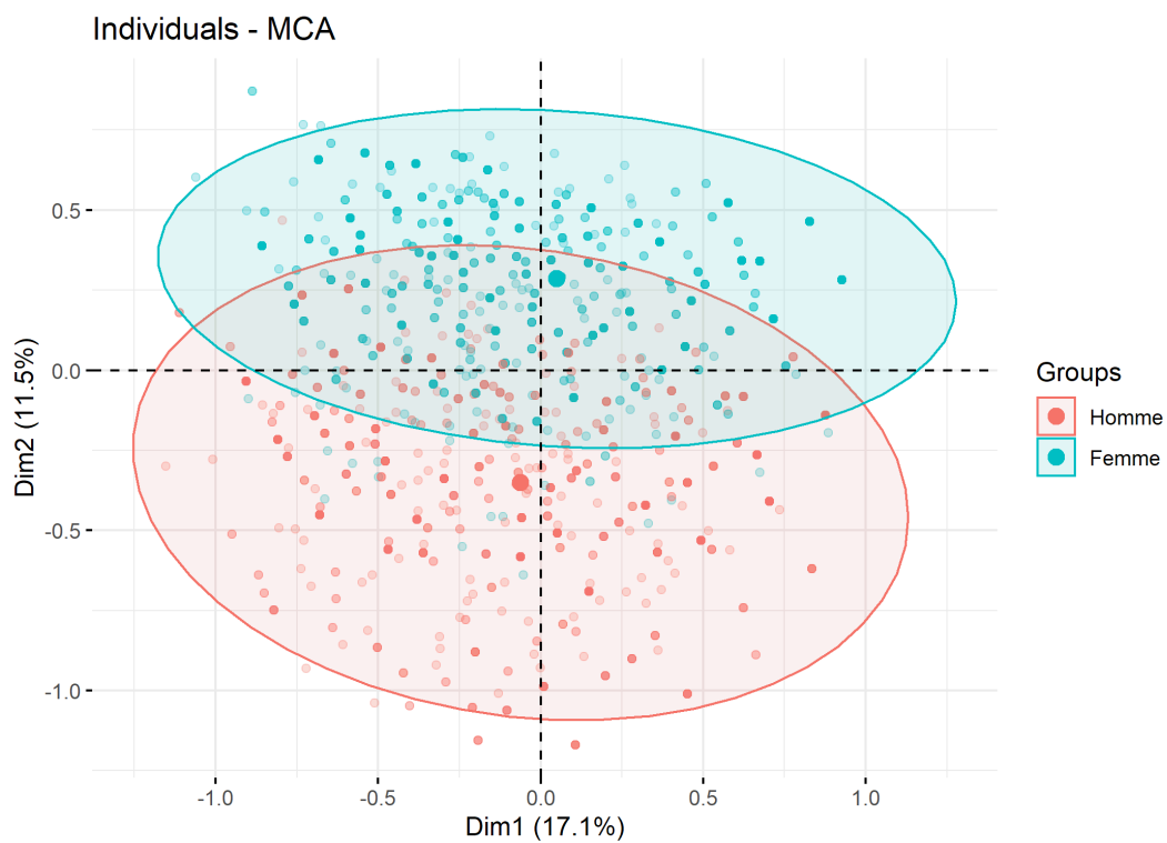
Figure 19. Individus dans le plan factoriel selon le sexe ( fviz_mca_ind )
