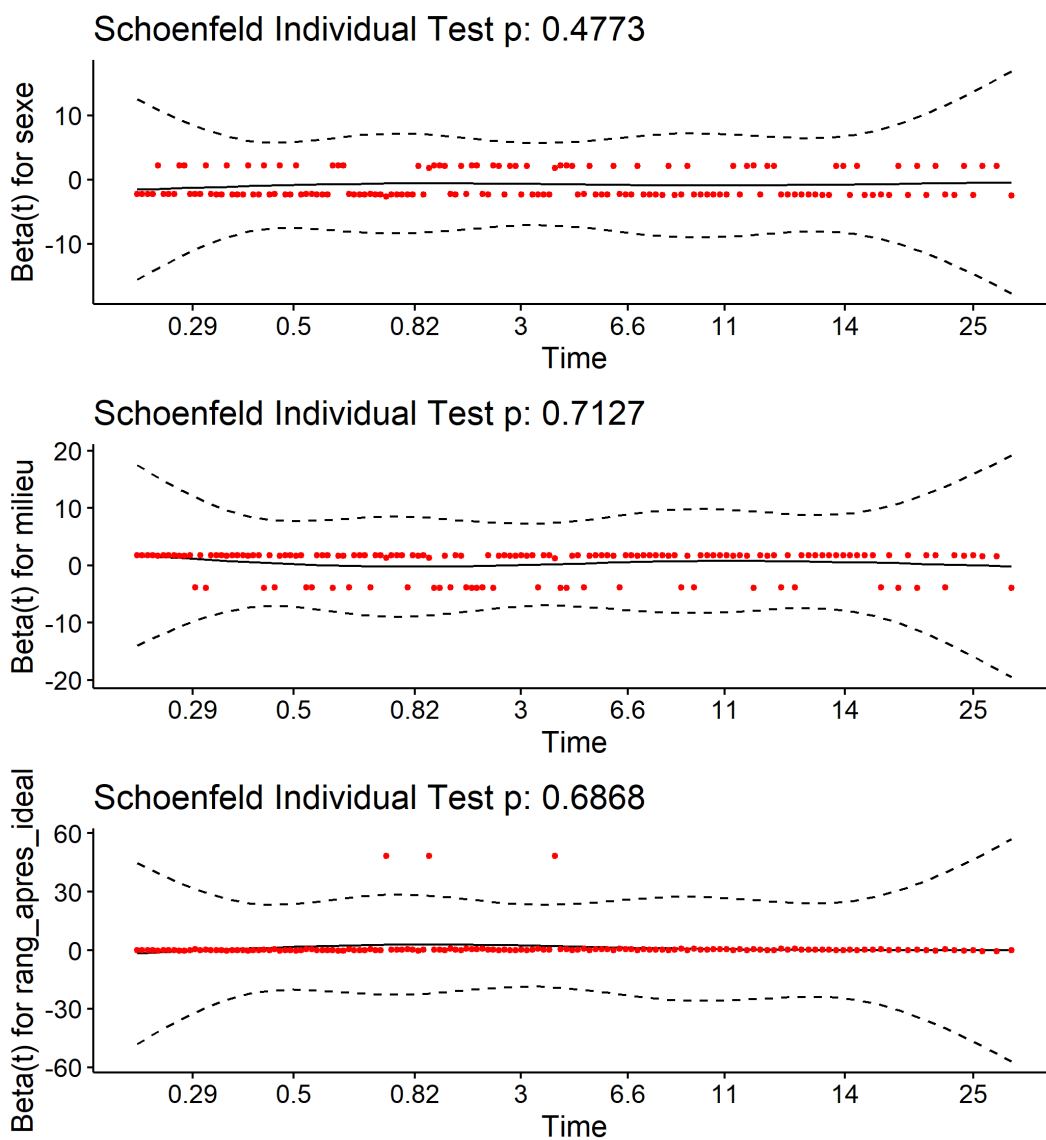
Figure 6. Résidus de Schoenfeld
