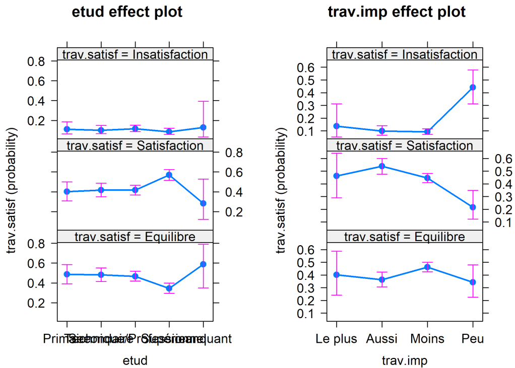
Figure 9. Effets marginaux du modèle multinomial
