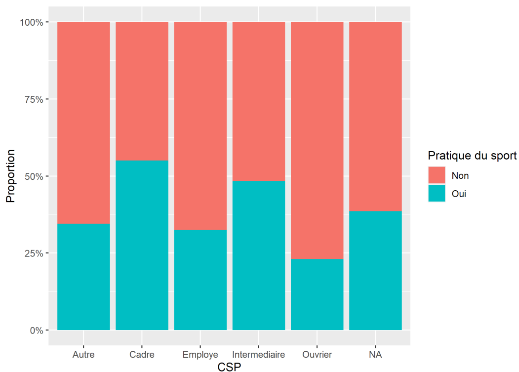
Figure 31. Diagramme en barres cumulées
