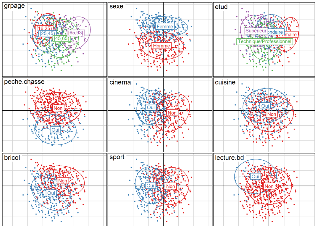
Figure 21. La fonction scatter appliquée au résultat d'une ACM
