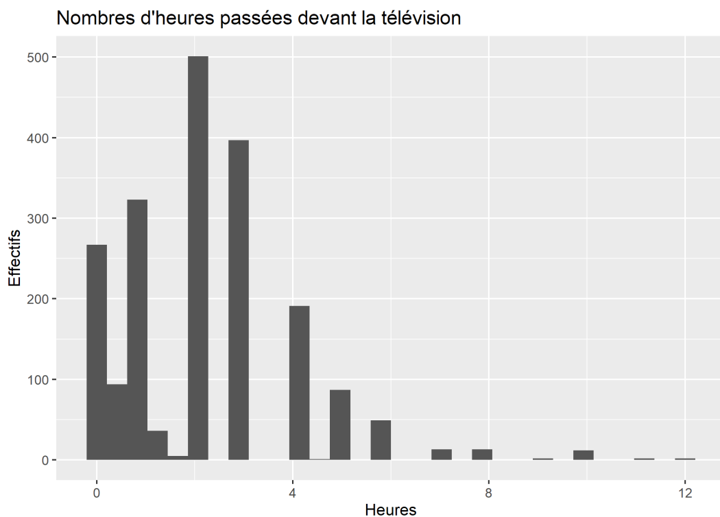
Figure 1. Un histogramme
