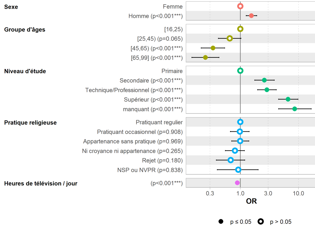
Figure 1. La fonction ggcoef_model
