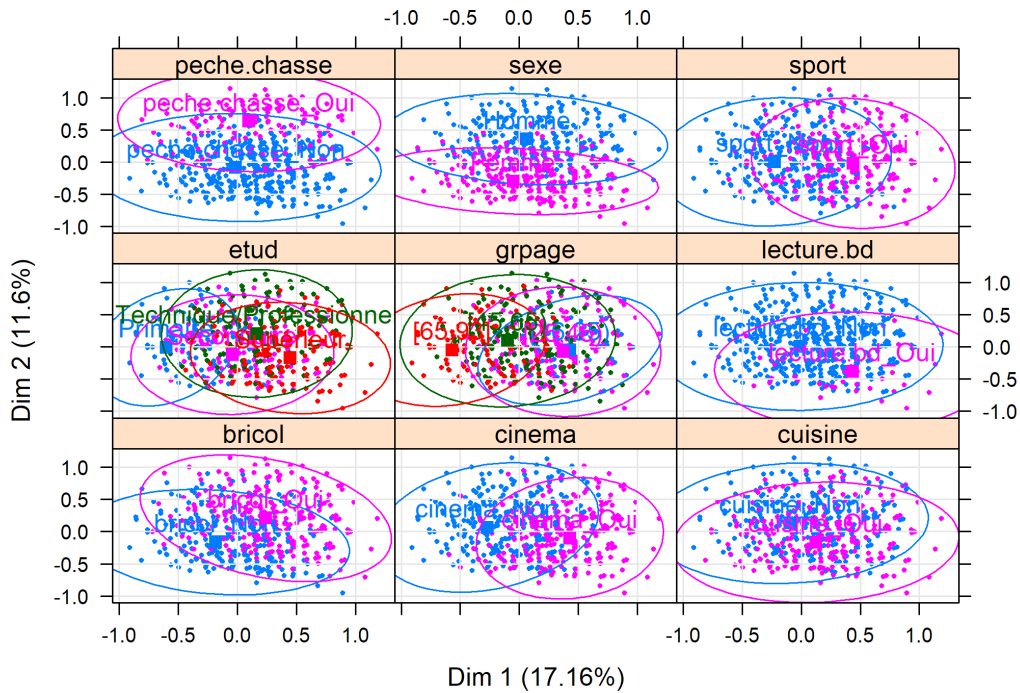
Figure 28. Ellipses de confiance (means=FALSE) dans le plan factoriel
