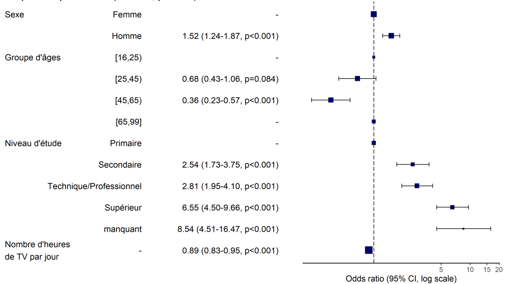
Figure 7. Graphique des odds ratios obtenu avec or_plot
