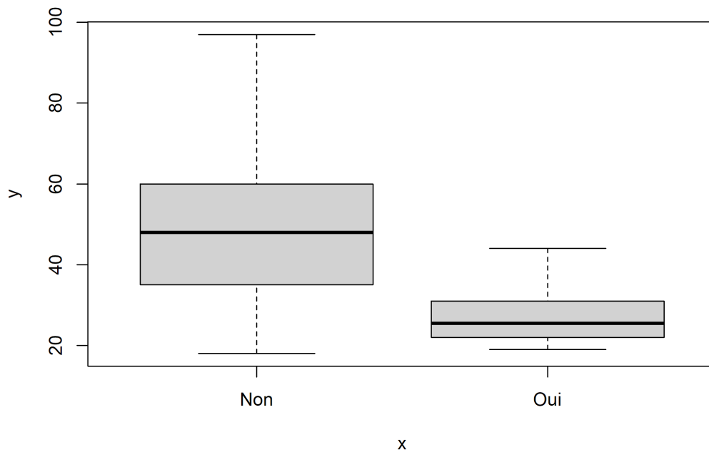
Figure 7. Âge des enquêtés selon qu'ils écoutent ou non du hard rock
