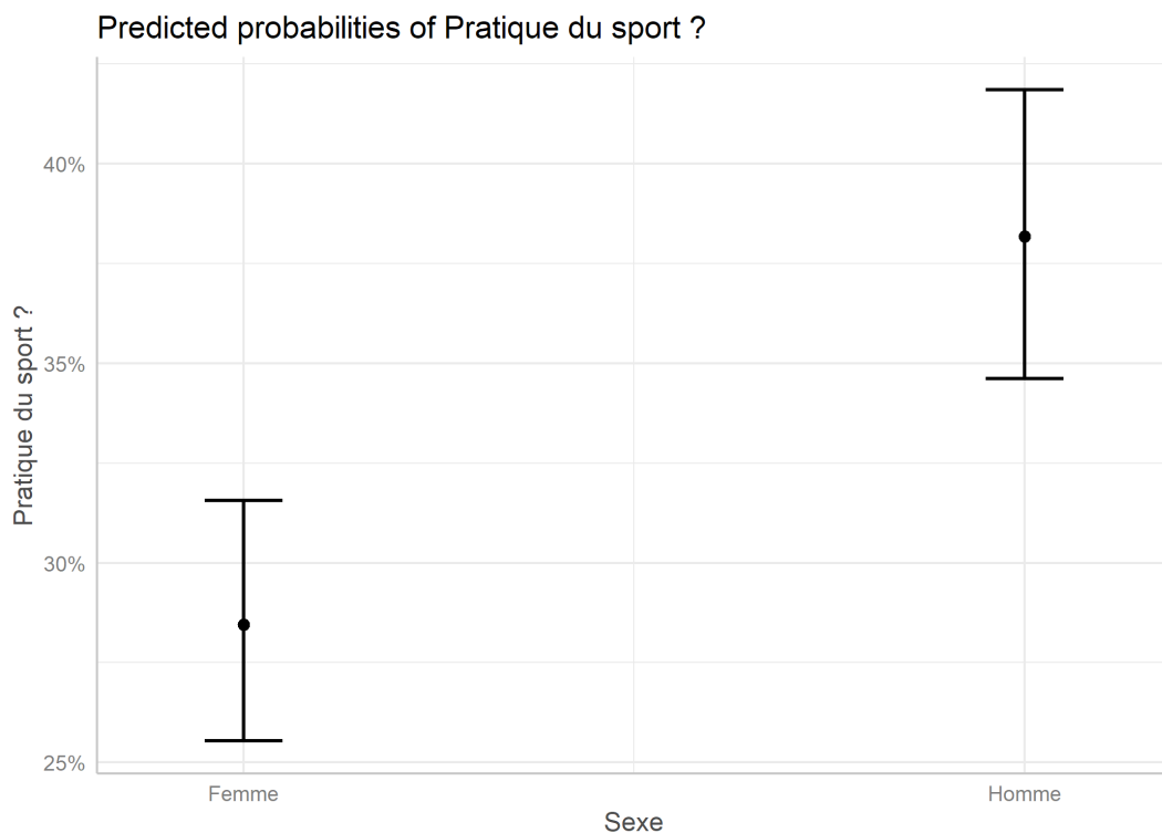
Figure 4. Effet du sexe représenté avec ggeffect
