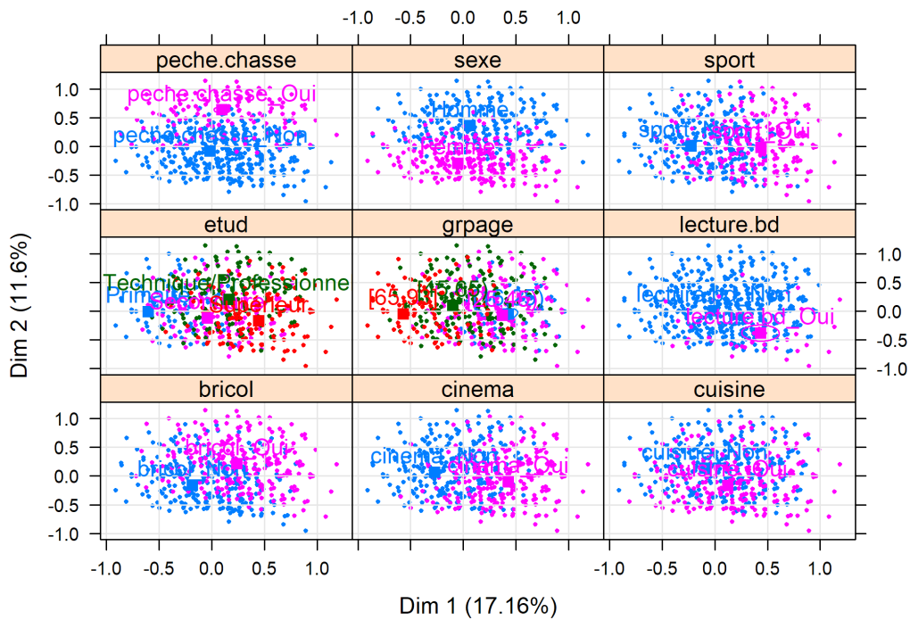
Figure 27. Ellipses de confiance (means=TRUE) dans le plan factoriel
