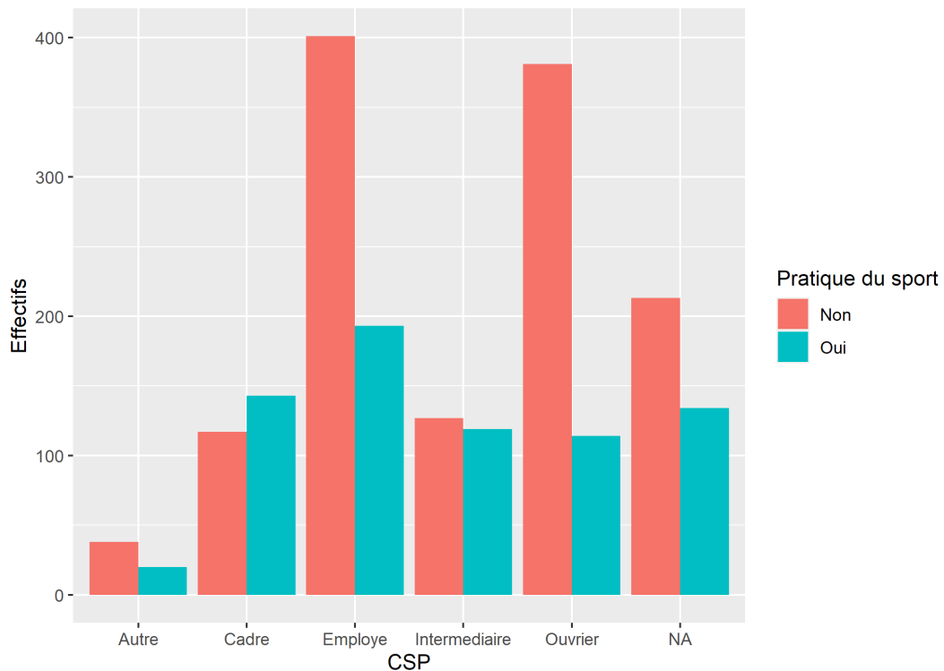
Figure 30. Diagramme en barres côte à côte
