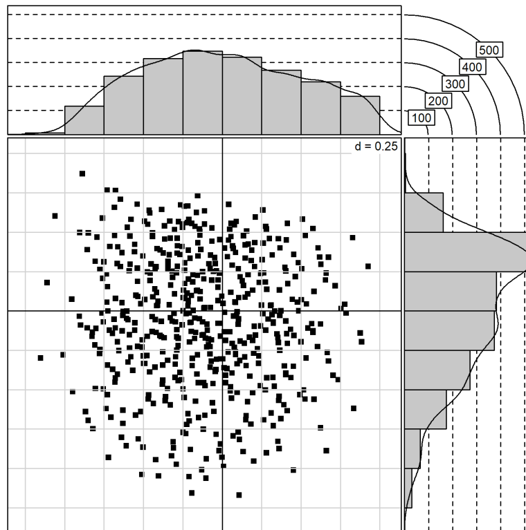
Figure 16. Distribution des individus dans le plan factoriel
