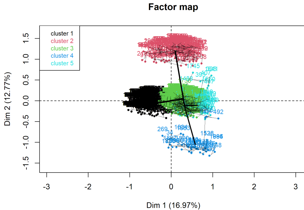
Figure 15. Projection des catégories sur le plan factoriel
