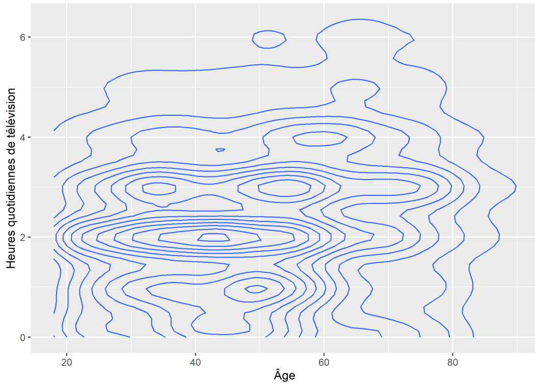
Figure 24. Estimation locale de densité (contours)
