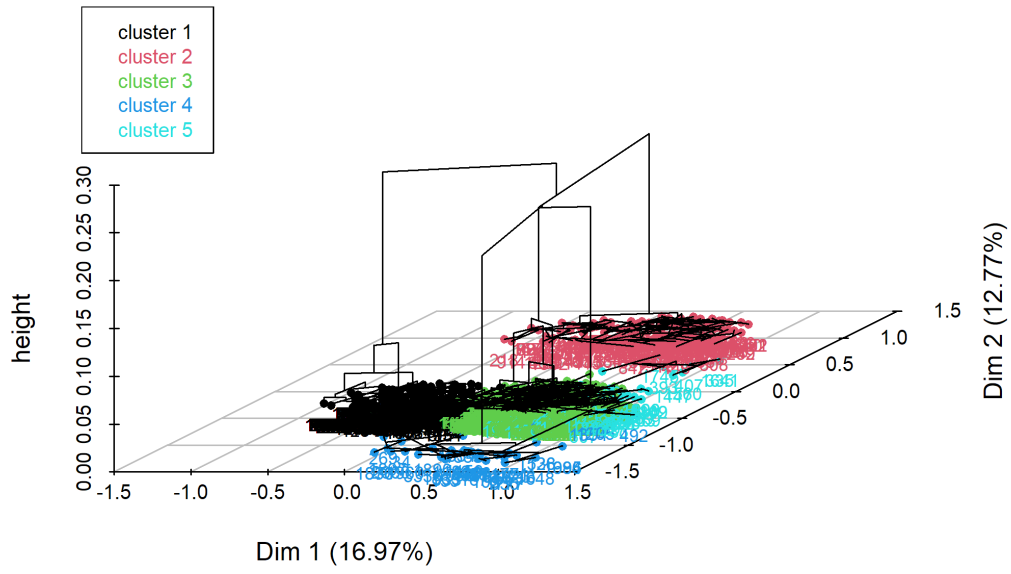
Figure 13. Représentation en 3 dimensions du dendrogramme
