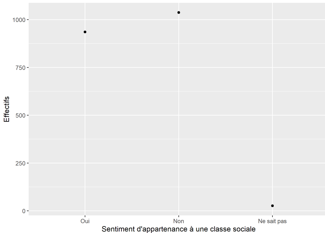
Figure 28. Diagramme de Cleveland
