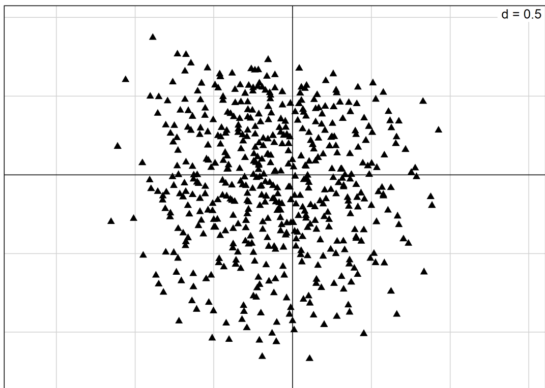
Figure 12. Répartition des individus selon les deux premiers axes
