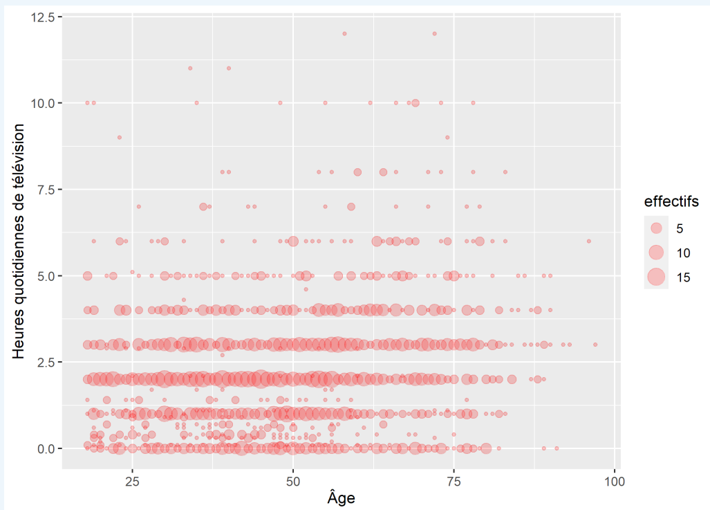
Figure 17. Nuage de points de taille proportionnelle au nombre d'observations
