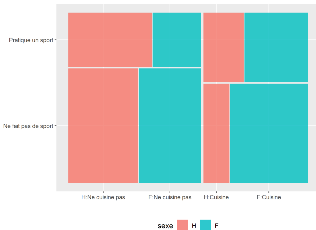
Figure 32. Graphique en mosaïque
