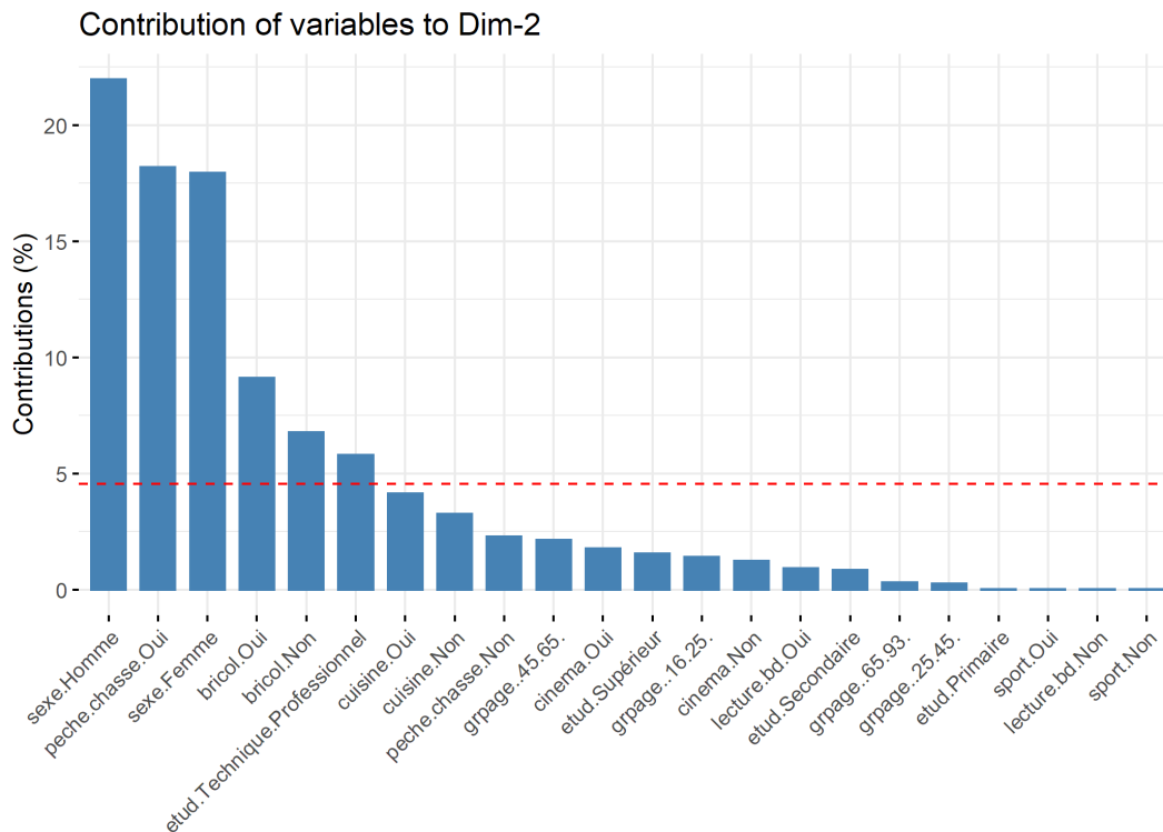
Figure 8. Représentation de la contribution des différentes variables
