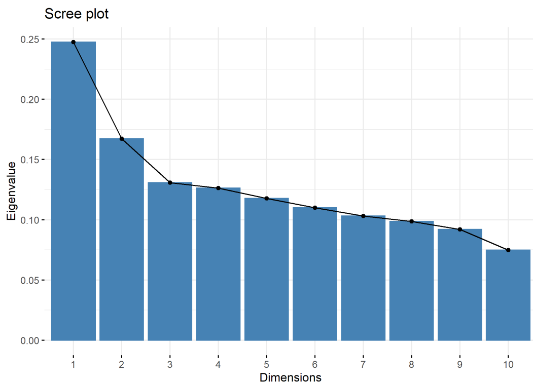
Figure 2. Valeurs propres des axe avec fviz_screplot()
