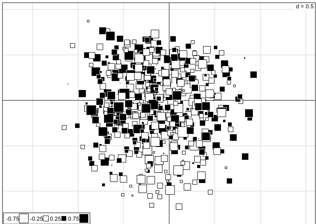
Figure 14. Répartition des individus selon les trois premiers axes
