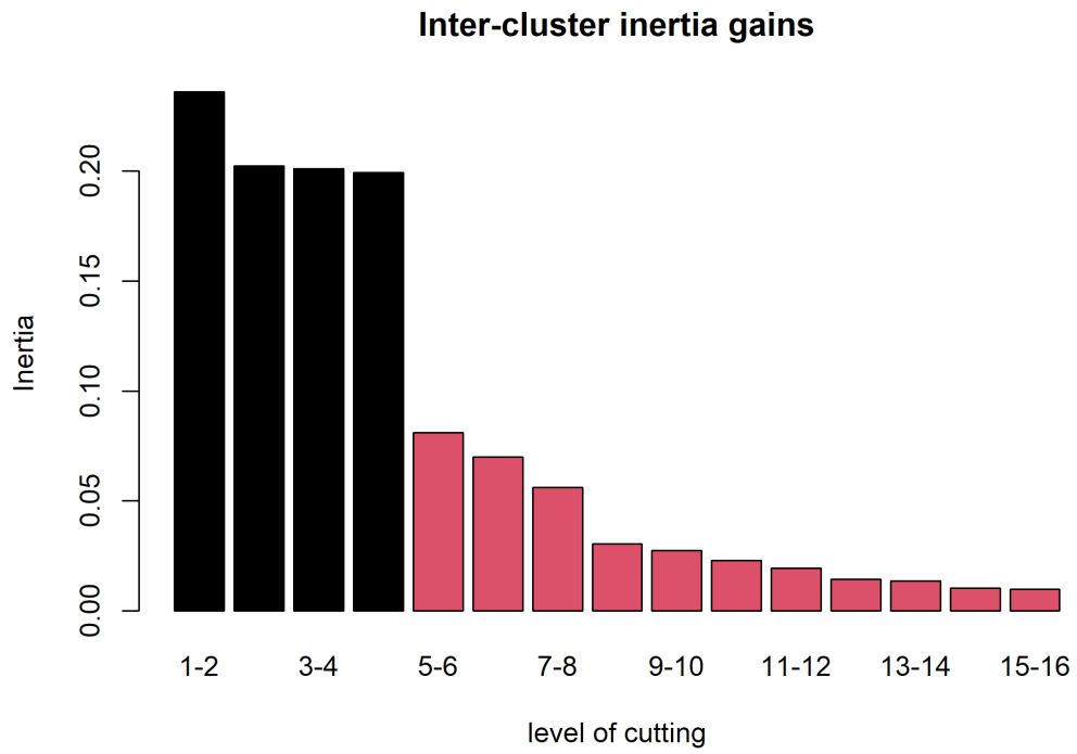
Figure 14. Gains d'inertie
