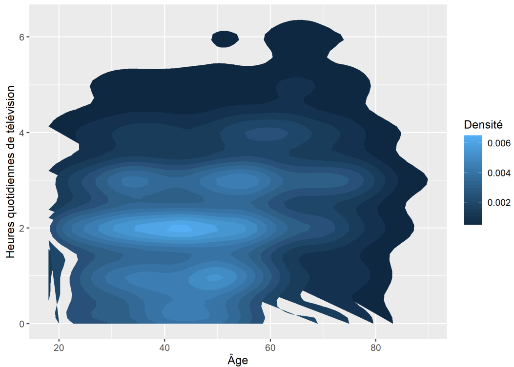
Figure 25. Estimation locale de densité (contours)
