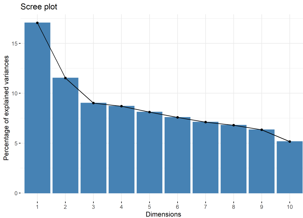
Figure 3. Pourcentage de variance expliquée avec fviz_screepLOT()
