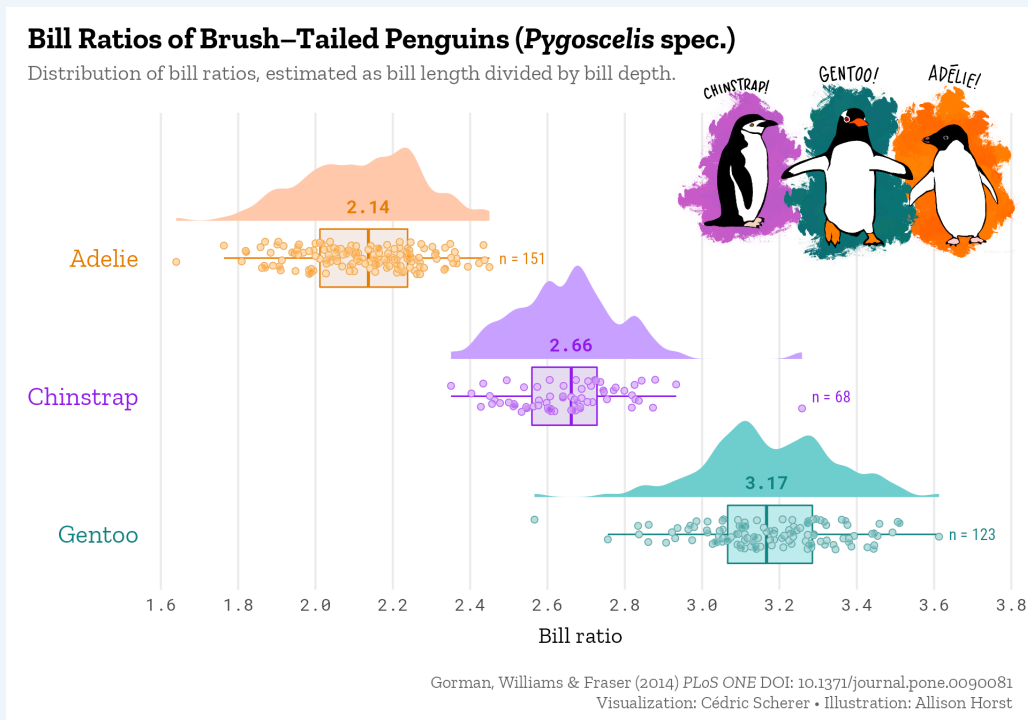
Figure 12. Exemple de graphique raincloud
