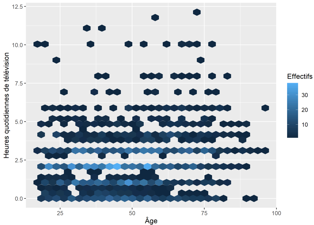
Figure 27. Effectifs en deux dimensions (hexagones)
