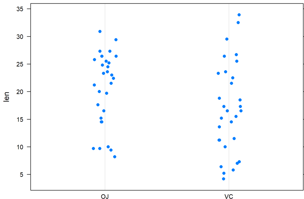
Figure 10. Diagramme en points
