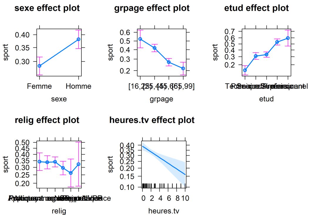
Figure 3. Représentation graphique de l'effet de chaque variable du modèle logistique
