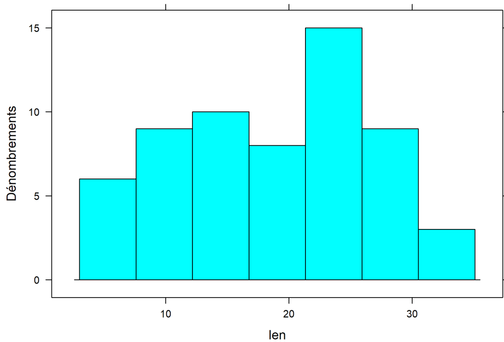
Figure 4. Histogramme d'effectifs
