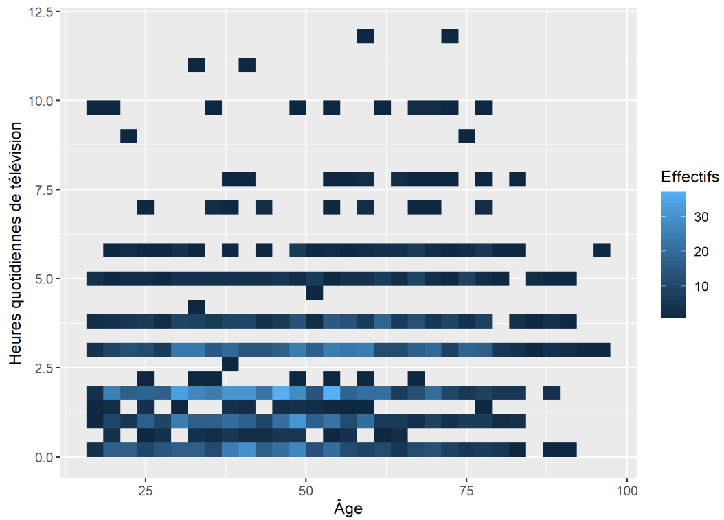
Figure 26. Effectifs en deux dimensions
