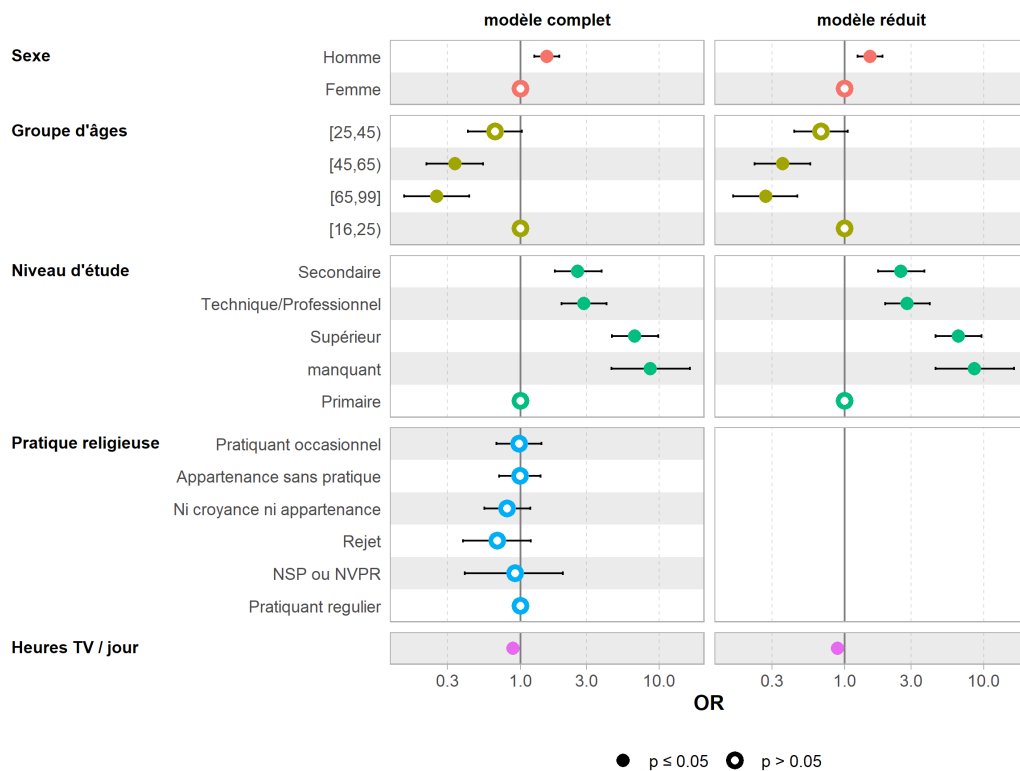
Figure 6. La fonction ggcoef_compare
