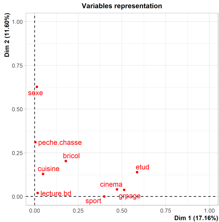
Figure 26. Plan factoriel (seulement les variables)
