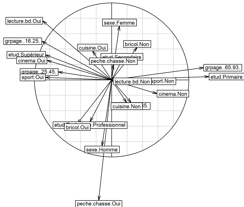
Figure 4. Cercle de corrélations des modalités sur les deux premiers axes
