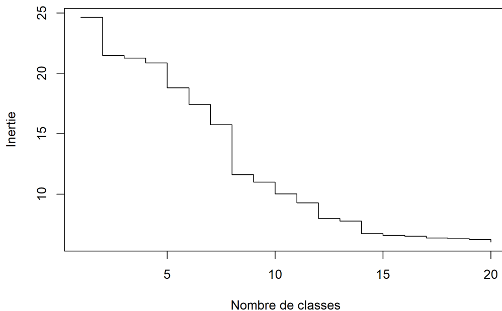
Figure 3. Inertie du dendrogramme
