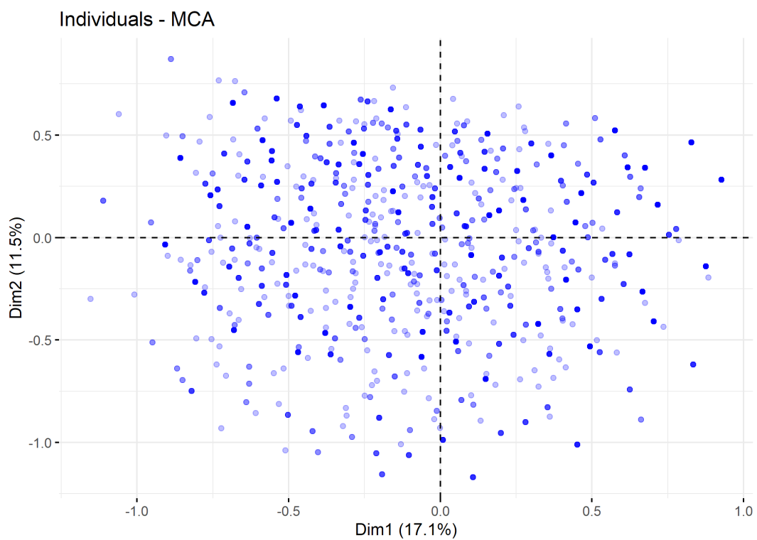
Figure 13. Répartition des individus selon les deux premiers axes avec fviz_mca_ind()
