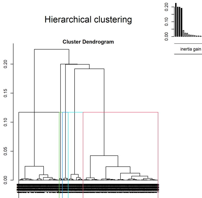
Figure 11. Dendrogramme obtenu avec HCPC (5 axes)
